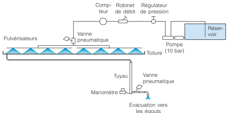
Fig. 6 Représentation schématique du système d’arrosage utilisé par le CSTC afin de déterminer les coefficients de retardement.
