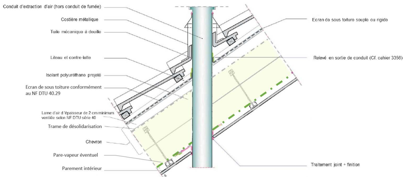
Figure 6 - Traversée de rampants de combles : éléments autres que les conduits de fumées
