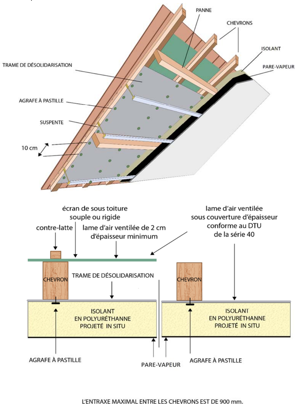
Figure 9 - Isolation avec une trame de désolidarisation agrafée en sous-face des chevrons
