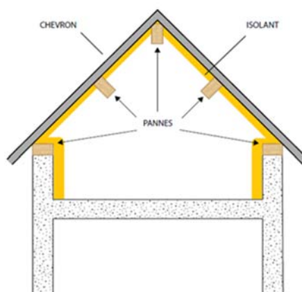
Figure 3 - Jonction avec les pannes
