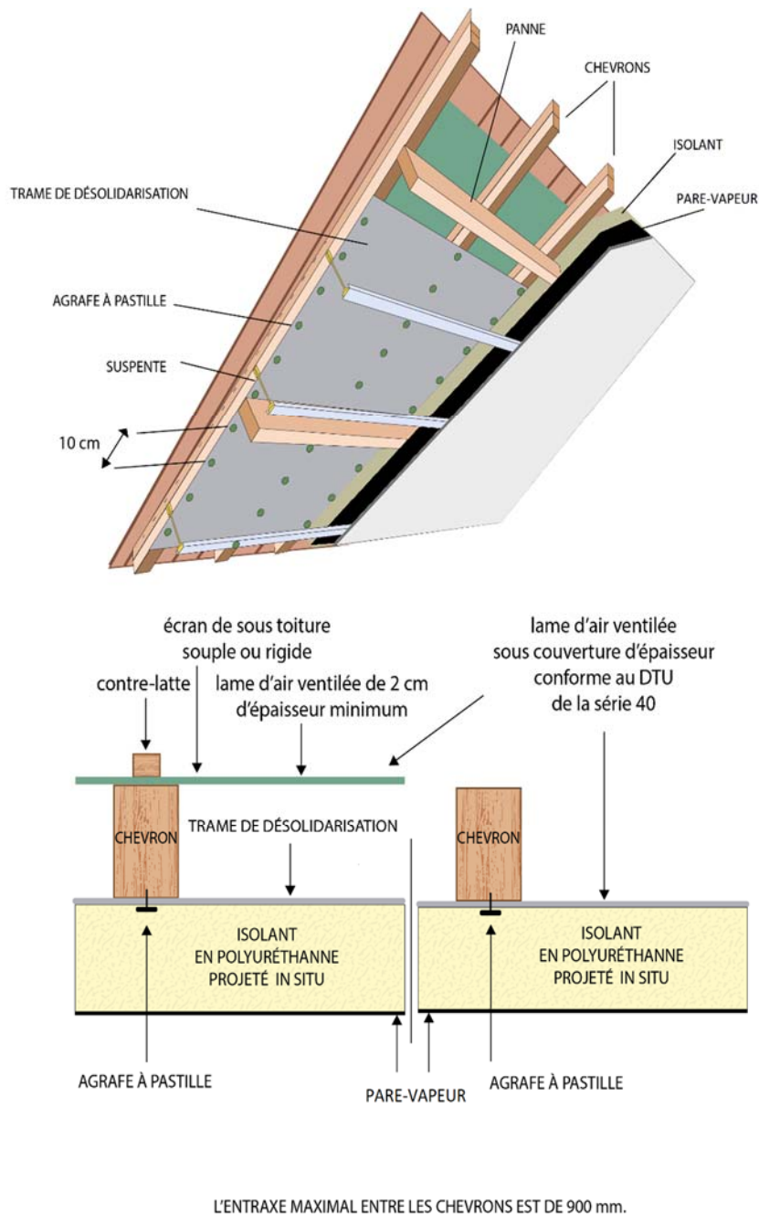
Figure 9 - Isolation avec trame de désolidarisation agrafée en sous-face des chevrons
