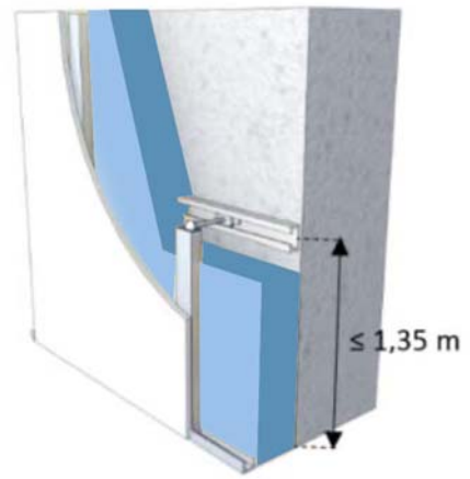
Figure 12 : Détail au droit d'un appui intermédiaire
