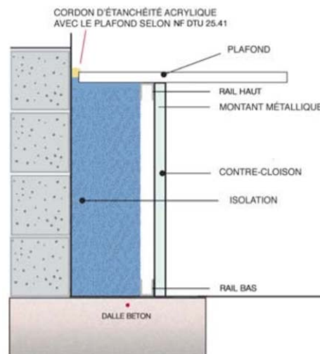
Figure 7 : Cordon d'étanchéité
