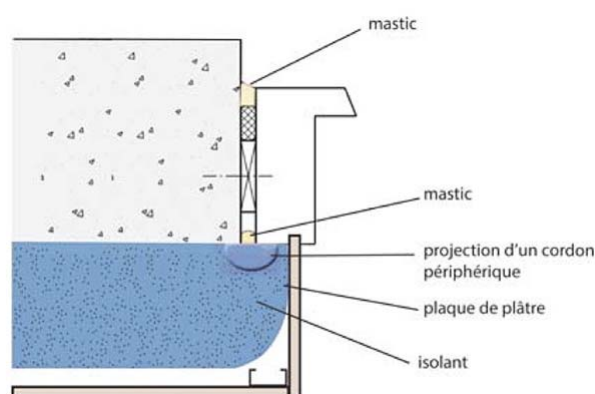
Figure 5 : Ouverture calfeutrée en tunnel, fixée en tableau
