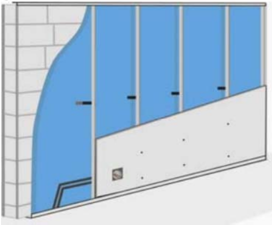
Figure 11 : contre-cloison constituée de fourrures avec appuis intermédiaires clipsés
