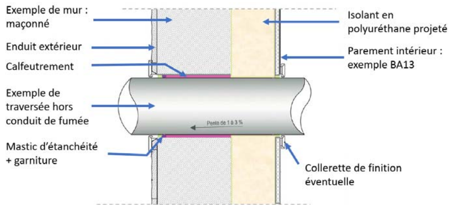
Figure 8 : Traversée de murs maçonnés : éléments autres que les conduits de fumées
