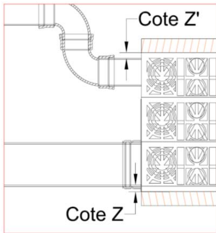
Figure 4a – Vue en coupe, continuité entre le canal d'inspection et le connecteur à bout femelle
