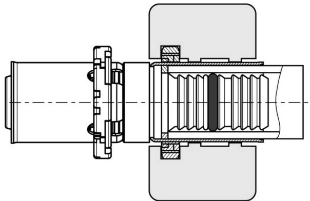
Figure 2 - Schéma de principe des raccords à sertir Skin Press Visu de COMAP
