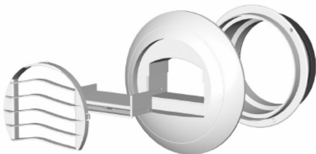
Figure 23 – Bouche d'extraction autoréglable ALIZÉ AUTO
