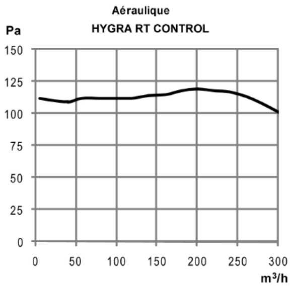
Figure 3 – Groupe d'extraction HYGRA RT CONTROL
