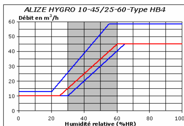
Figure 19d – Caractéristiques hygroaérauliques nominales des bouches d'extraction hygroréglables pour une différence de pression de 80 Pa, modèle ALIZÉ HYGRO 10-45, 25-60 %HR
