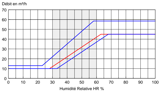
Figure 19e – Caractéristiques hygroaérauliques nominales des bouches d'extraction hygroréglables pour une différence de pression de 80 Pa, modèle ALIZE HYGRO VISION 10-45/45, 28-63%HR
