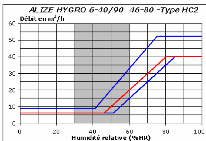
Figure 17a – Caractéristiques hygroaérauliques nominales des bouches d'extraction hygroréglables pour une différence de pression de 80 Pa, modèle ALIZÉ HYGRO 6-40/90, 46-80 %HR
