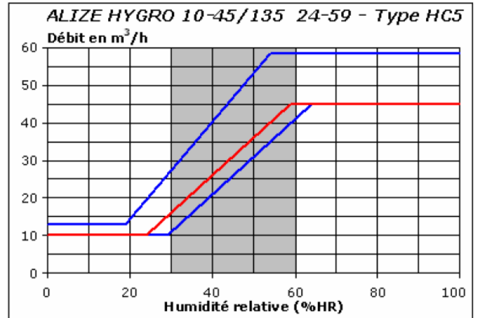
Figure 17d – Caractéristiques hygroaérouliques nominales des bouches d'extraction hygroréglables pour une différence de pression de 80 Pa, modèle ALIZÉ HYGRO 10-45/135, 24-59 %HR
