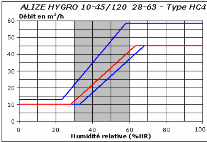
Figure 17c – Caractéristiques hygroaérouliques nominales des bouches d'extraction hygroréglables pour une différence de pression de 80 Pa, modèle ALIZÉ HYGRO 10-45/120, 28-63 %HR
