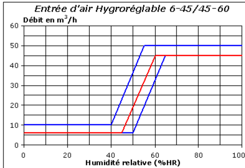
Figure 6 – Caractéristiques hygroaérauliques nominales données pour une différence de pression de 20 Pa pour les entrées d'air hygroréglables.
