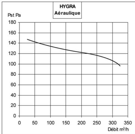
Figure 1 – Groupe d'extraction Hygra
