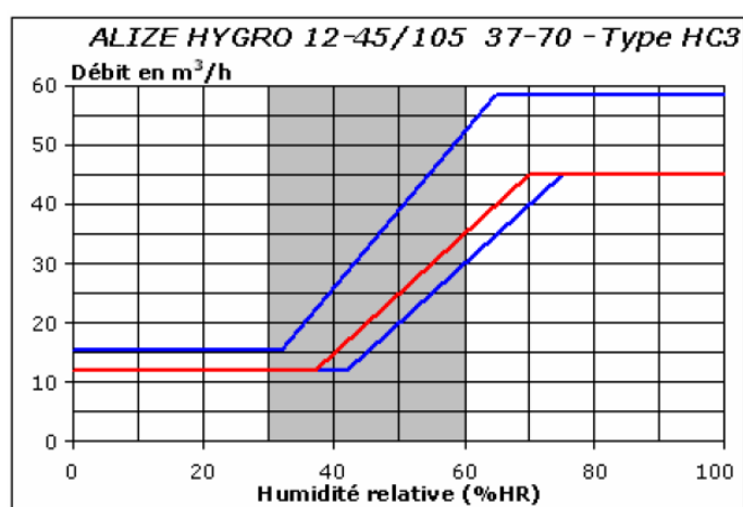
Figure 17b – Caractéristiques hygroaérauliques nominales des bouches d'extraction hygroréglables pour une différence de pression de 80 Pa, modèle ALIZÉ HYGRO 12-45/105, 37-70 %HR
