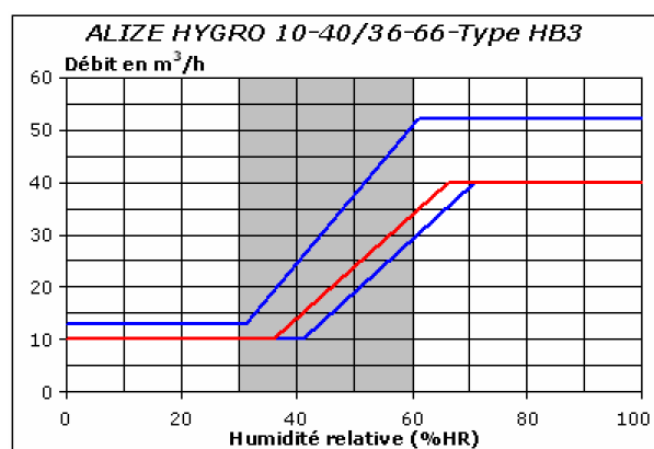
Figure 19c – Caractéristiques hygroaérauliques nominales des bouches d'extraction hygroréglables pour une différence de pression de 80 Pa, modèle ALIZÉ HYGRO 10-40, 36-66 %HR
