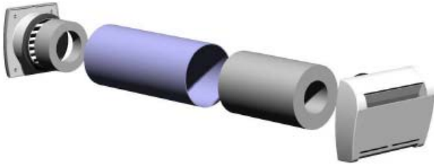
Figure 15 – Silencieux SC + EM HY
