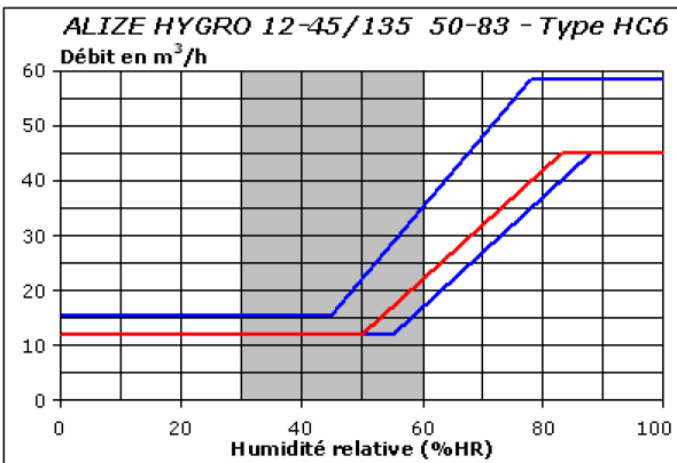
Figure 17e – Caractéristiques hygroaérouliques nominales des bouches d'extraction hygroréglables pour une différence de pression de 80 Pa, modèle ALIZÉ HYGRO 12-45/135, 50-83 %HR
