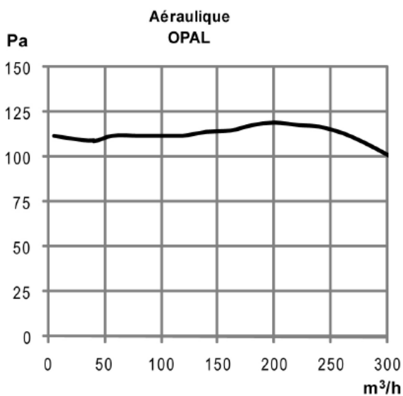
Figure 2 – Groupe d'extraction OPAL
