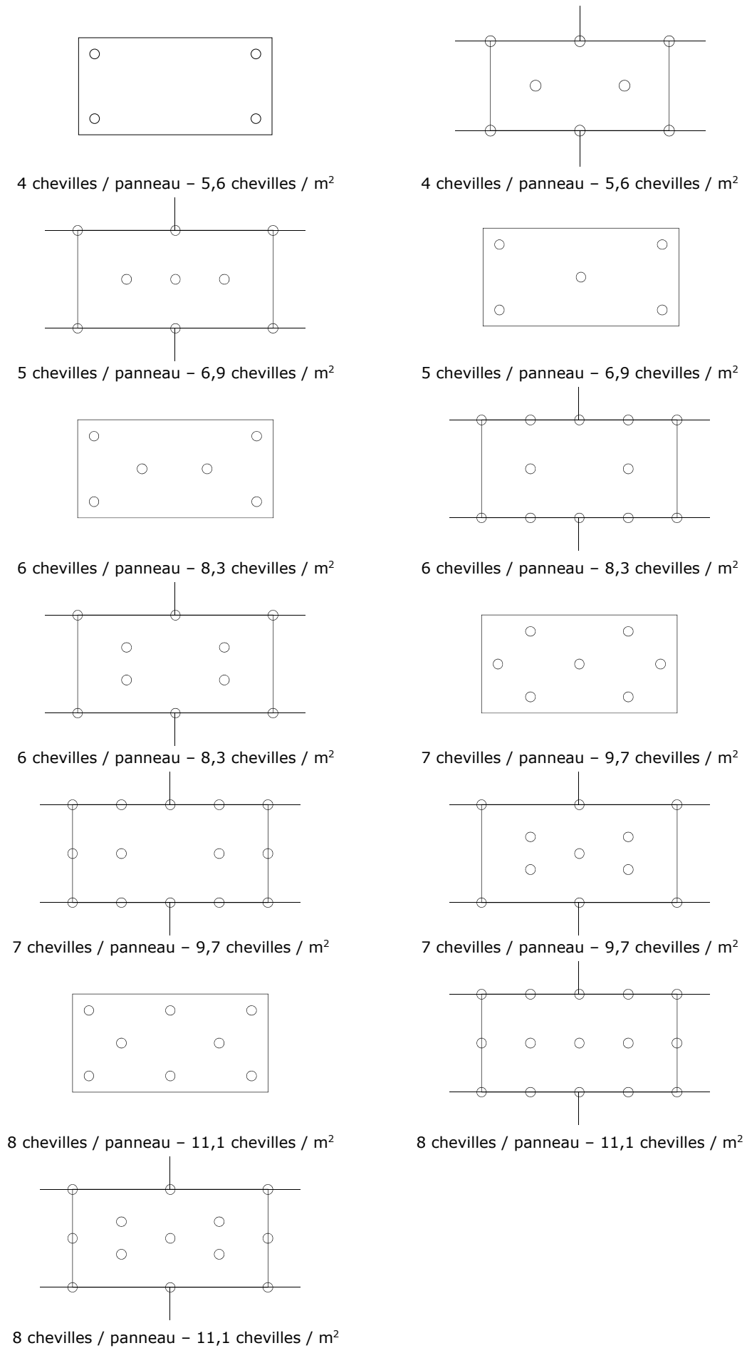
Figure 1b : Plans de chevillage - panneaux de dimensions 1200 x 600 mm
