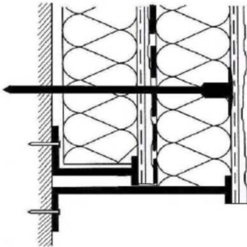
Figure 4c : nouveau profilé de départ inversé sans dépose de l'existant
