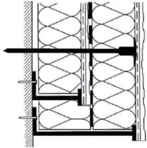
Figure 4b : nouveau profilé de départ sans dépose de l'existant
