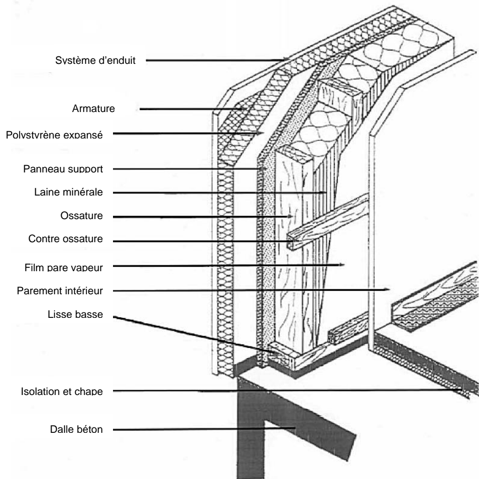
Figure 1 : Principe du système ARMATERM BOIS POUFRE PSE (fixation du polystyrène expansé non représentée)
