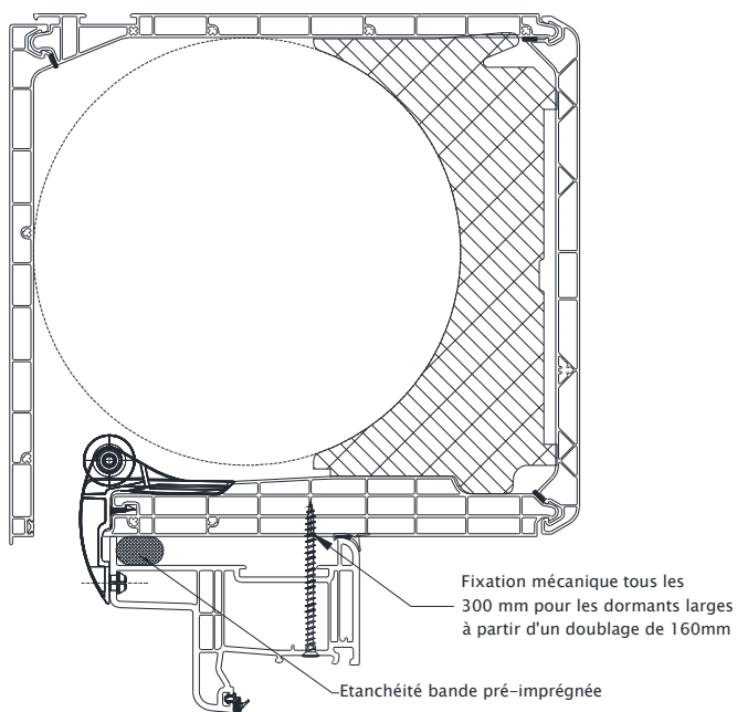
Largeur de coffre 0 à 2000
