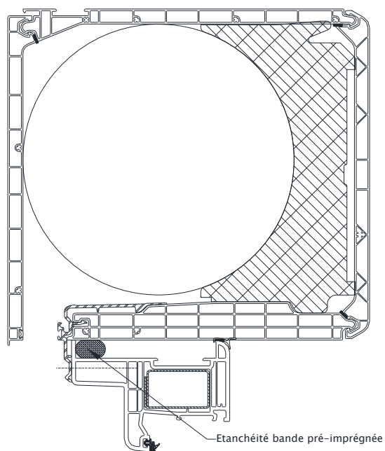
Largeur de coffre > 2000
