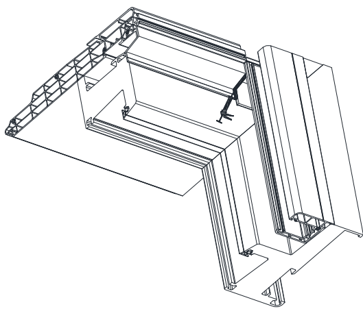
Raccord d'Etanchéité Adaptateur
