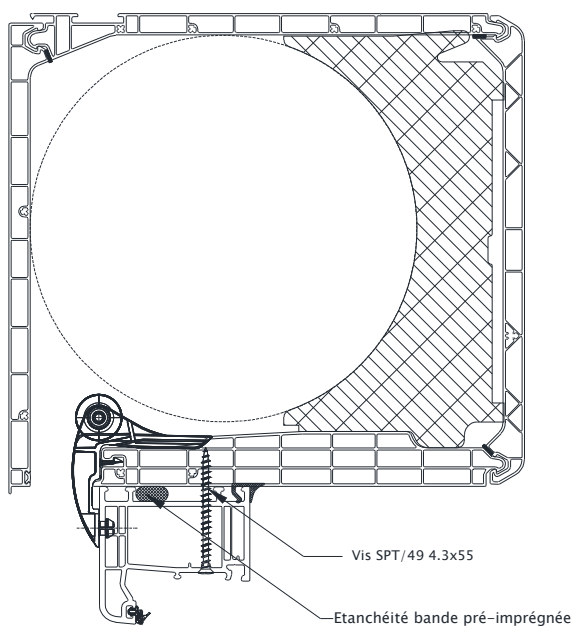
Largeur de coffre 0 à 2000
