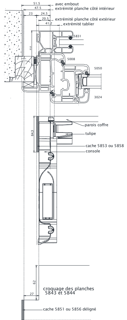
Mise en oeuvre frappe en réno
