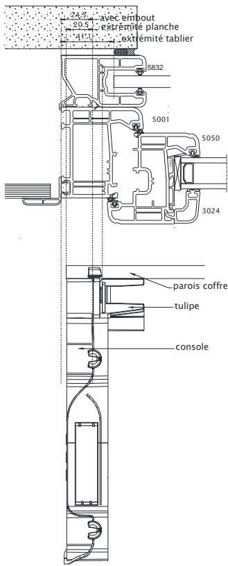
Mise en oeuvre en applique interieur
