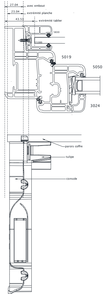
Mise en oeuvre en applique interieur doublage de 100 mm
