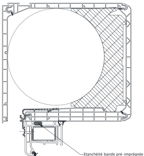
Largeur de coffre > 2000
