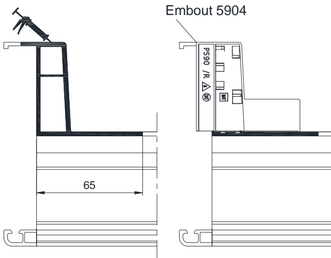
Mise en place Embout avant montage VR
