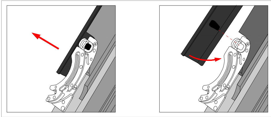
Emboîtement Profilé
