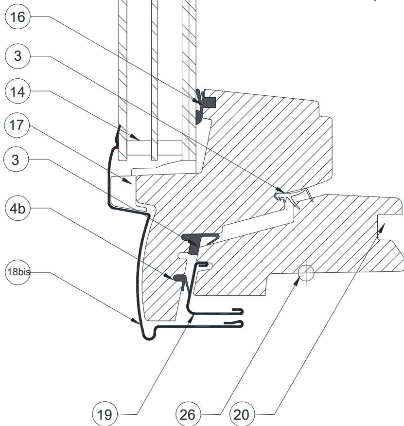
Coupe verticale Variante capot 1
