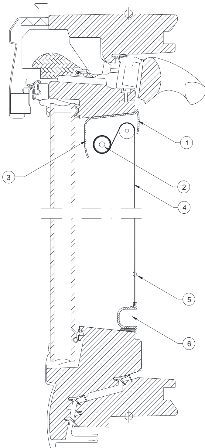
Coupe verticale
