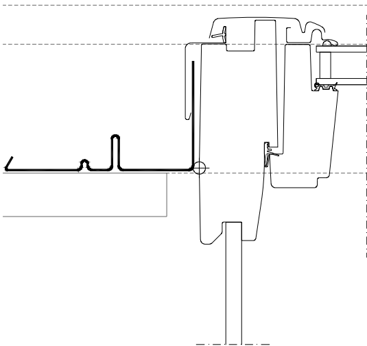
FENETRE ET POSITION GENERATION 1992 ET ANTERIEURE
