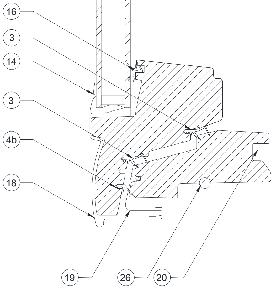
Coupe verticale Variante capot 2
