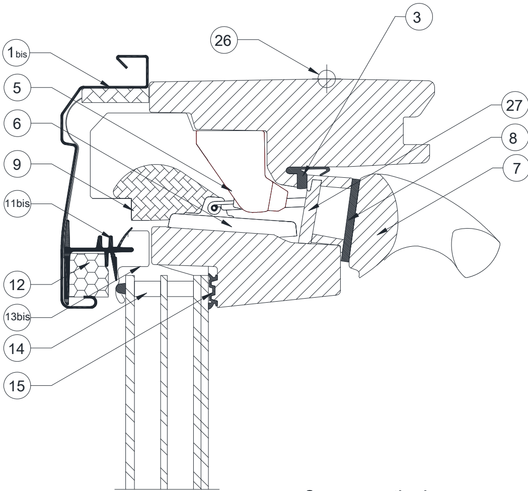
Coupe verticale Variante capot 2
