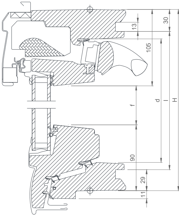
Coupe verticale
