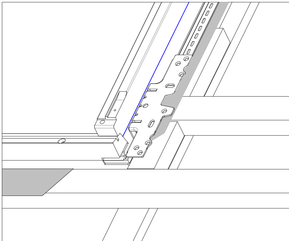
POSE ENCASTREE NIVEAU TRAIT BLEU
