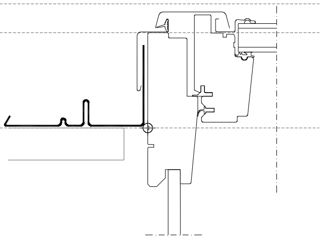
FENETRE NOUVELLE GENERATION ET POSITION 'RENOVATION'
