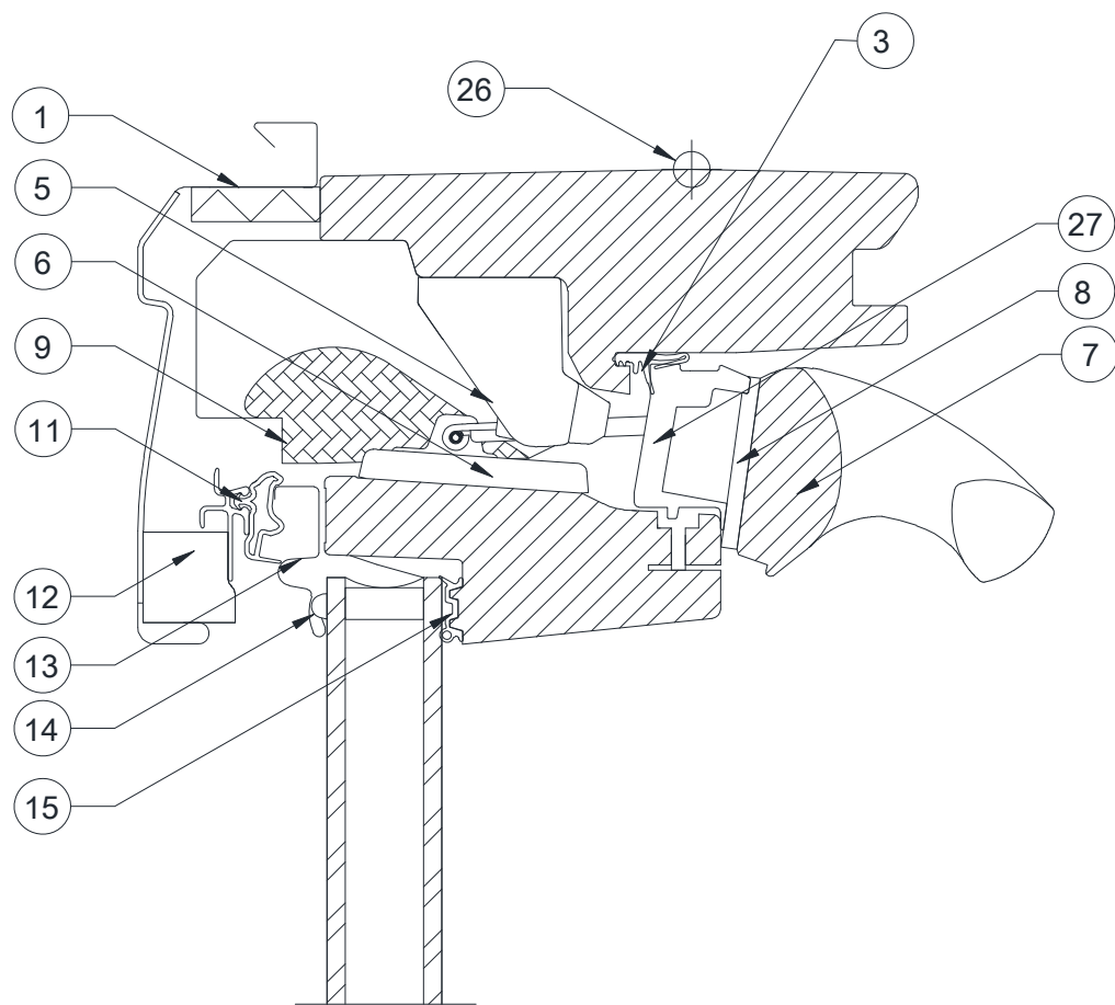
Coupe verticale Variante capot 1
