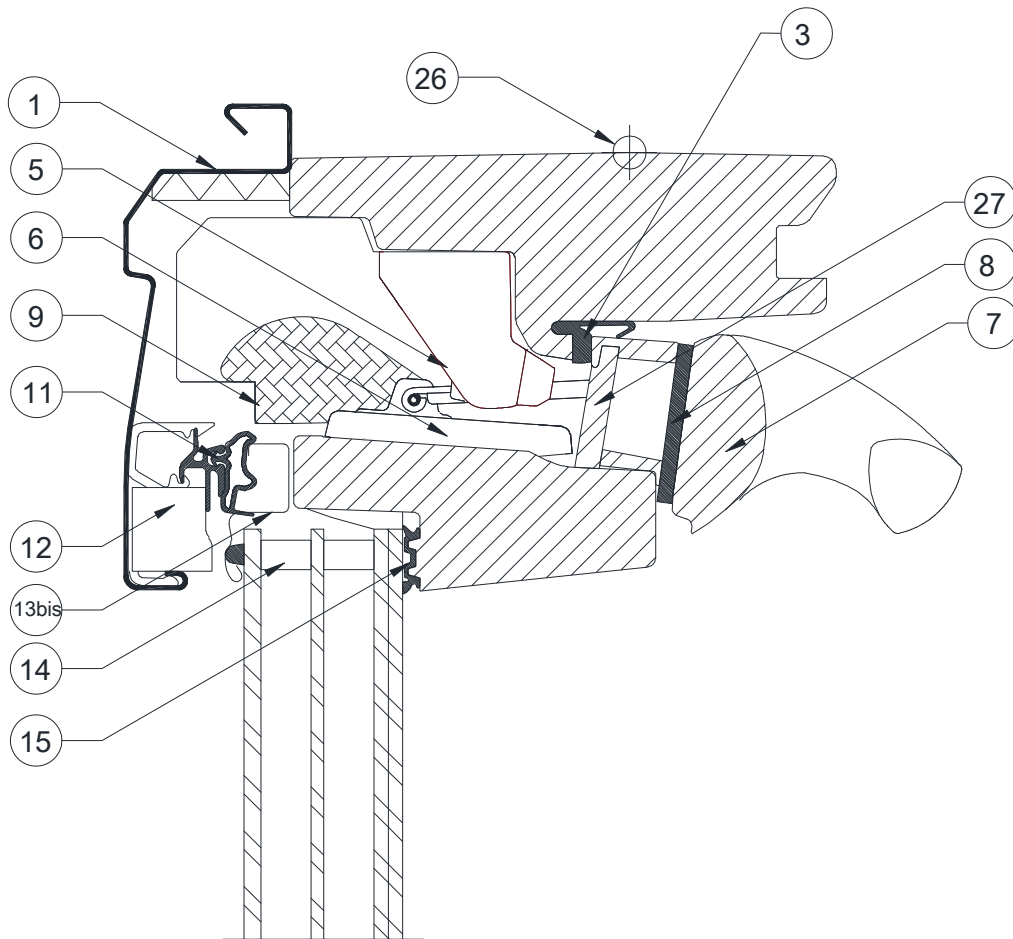
Coupe verticale Variante capot 1
