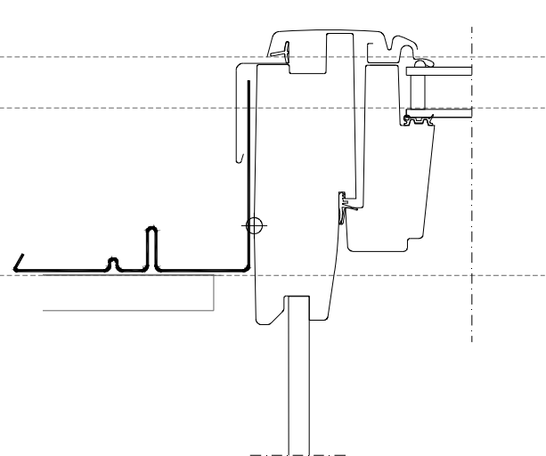
FENETRE NOUVELLE GENERATION ET POSITION 'RENOVATION'
