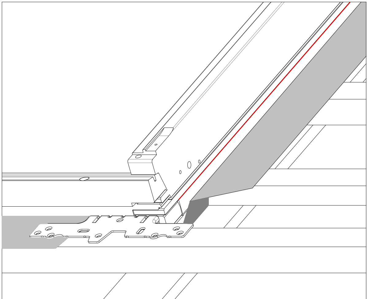
POSE STANDARD NIVEAU TRAIT ROUGE
