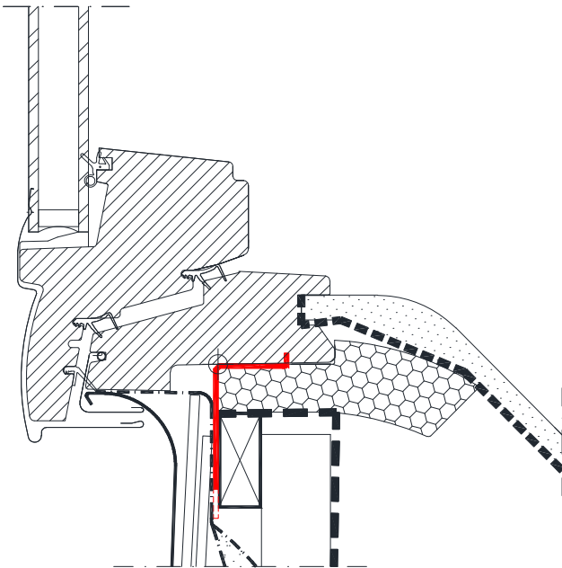
POSE STANDARD NIVEAU TRAIT ROUGE
