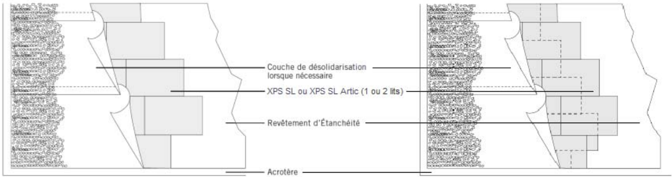
Figure 11 – Vue de dessus de principe d'une toiture inversée
