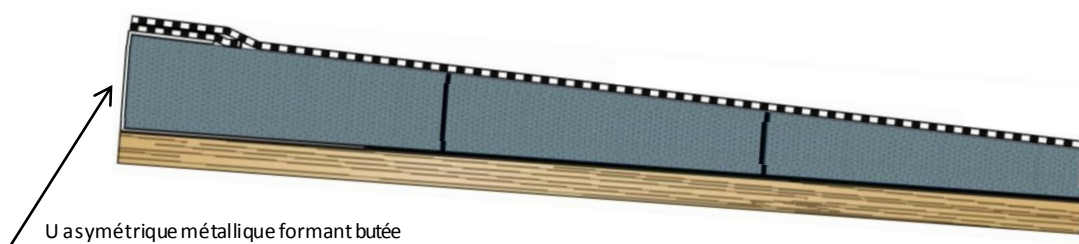
Figure 6b – Coupe de principe sur rive sans acrotère, sur élément porteur bois - panneaux à base de bois 1
