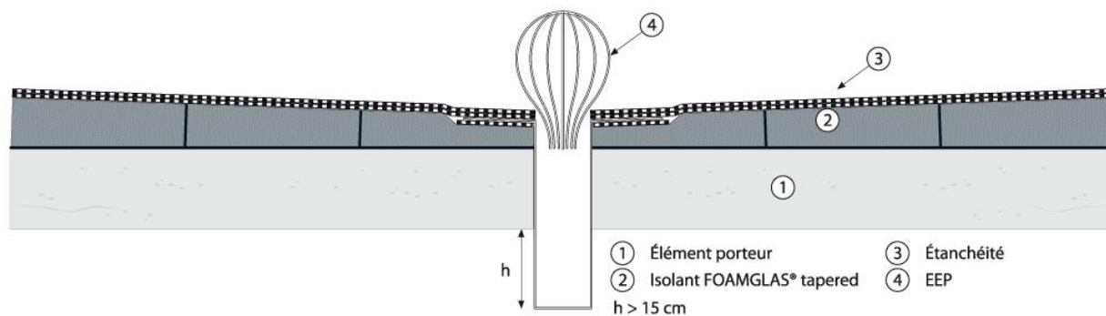
Figure 5 – Coupe sur une Entrée d'Eaux Pluviales (EEP)
