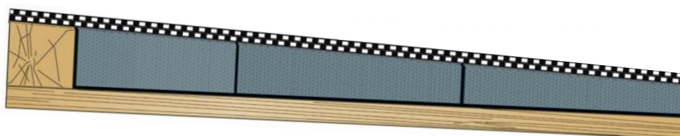
Figure 6c – Coupe de principe sur rive avec butée en bois, sur élément porteur bois - panneaux à base de bois 1
