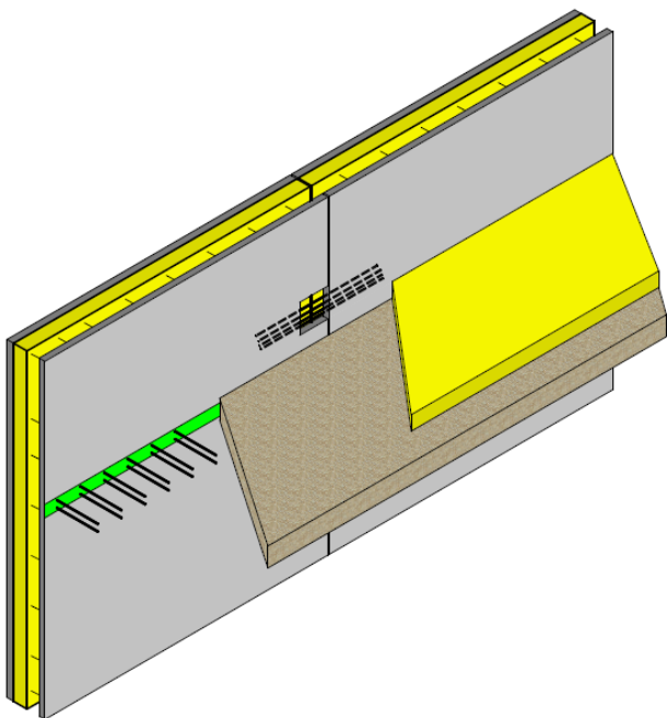
Figure 46 : Acrotère haut réalisé par prolongement de l'Inov'Mur (i) dont la paroi « intérieure » n'est pas isolée
