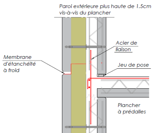
Figure 50a : Détails sur joints horizontaux : paroi extérieure plus haute de 15 mm vis-à-vis du plancher
