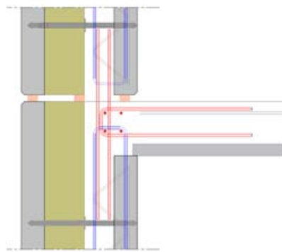
Figure 24 : Liaison dalle/ Inov'Mur (1) encastrée
