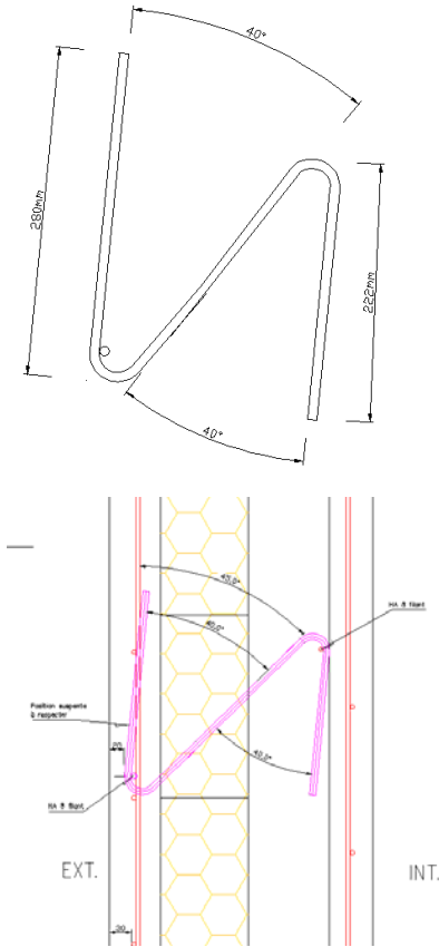
Figure 6 : Coupes sur les suspentes Inox de l'Inov'Mur (i)
