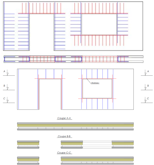
Figure 13a : Réalisation de chaînage en Inov'Mur (i)
