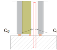
Figure 15 : Position des armatures en attente dans l'Inov'Mur (1)
