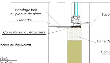
Coupe C
