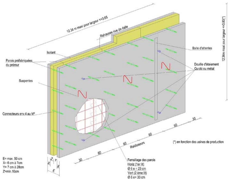
Figure E1.1 : Eclaté de l'Inov'Mur (1)
