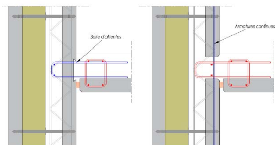
Figure 23 : Liaison rotulée de l'Inov'Mur (1) avec une dalle suspendue (hors exigence de vérification sismique)
