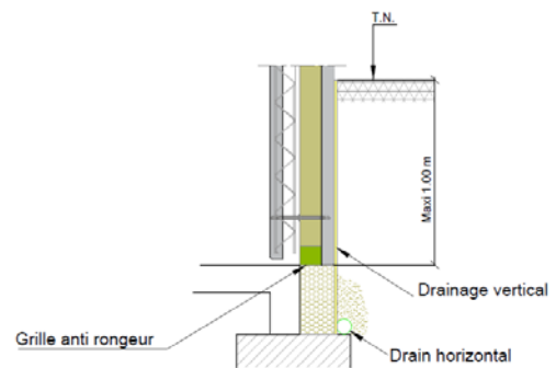
Figure 8a : Murs semi-enterrés de hauteur <= 1,00 m
