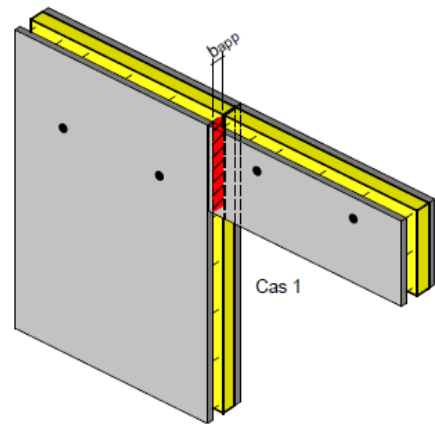
Figure 42 : Appui de poutre → Cas 1
