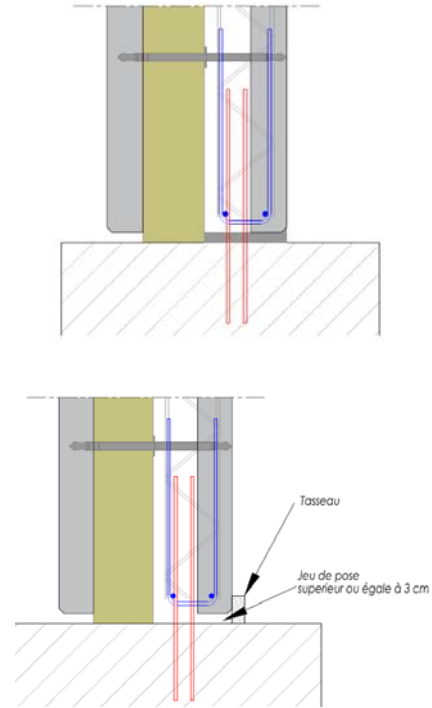
Figure 20 : Encastrement de l'Inov'Mur(i)/radier → Liaison de type Er1
