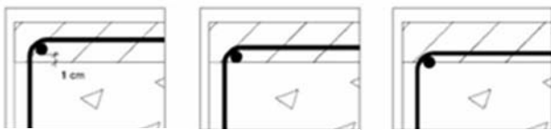
Cas A Périmètre utile = u Cas B Périmètre utile = 0,80 \times u Cas C Périmètre utile = 0,50 \times u
