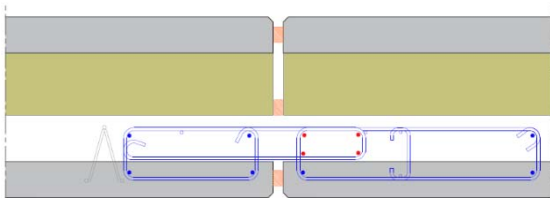
Figure 28 : Joint vertical encastré - Type de type Ev1
