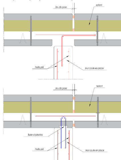
Figure 26 : Liaison en T entre un Inov'Mur (1) et un mur coulé en place.
