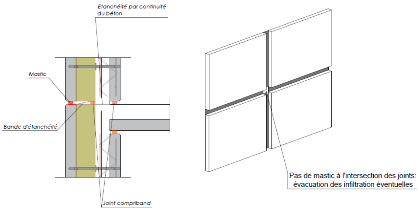
Figure 1.3.1 : Traitement des joints verticaux et horizontaux
