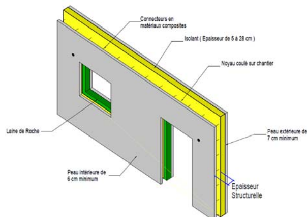
Figure 1 : Définition de l'Inov'Mur (1)
