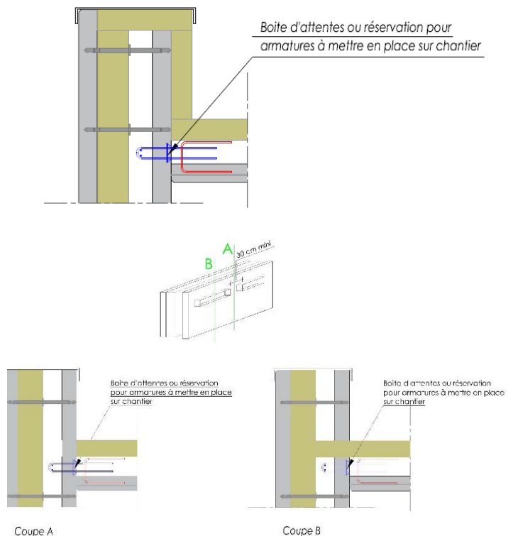
Figure 44 : Acrotères avec dalle suspendue – hors zone sismique
