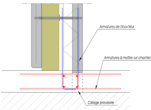
Figure 19b : Encastrement de l'Inov'Mur(i)/radier → Liaison de type E2
