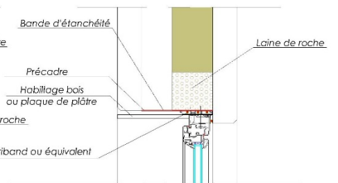
Coupe B
