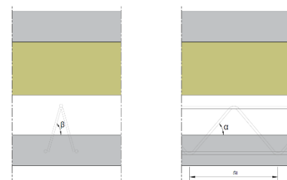
Figure 13c : Définition des raidisseurs de l'Inov'Mur (i)
