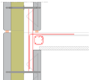
Figure 22 : Liaison rotulée de l'Inov'Mur (1) avec une dalle
