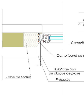
Coupe A
