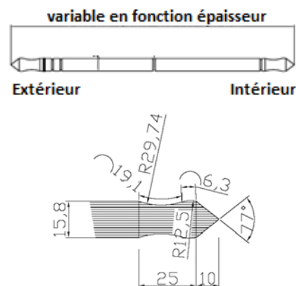
Figure 4 : Vue du connecteur - le diamètre courant de 15,8 mm et des gorges de 13 mm
