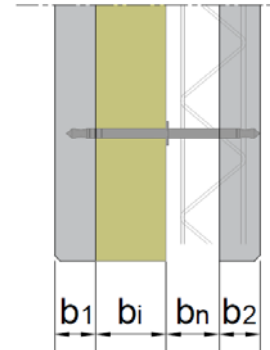
Figure 10 : Définition pour les calculs thermiques
