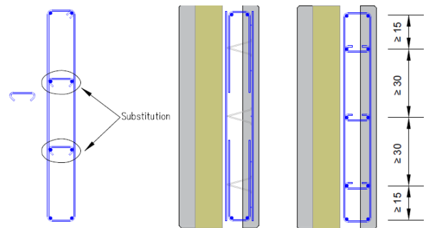
Figure 13b : Solution traditionnelle et de l'Inov'Mur (i)
