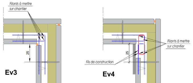
Figure 30 : Liaisons d'angle encastrées - Type Ev3 (à gauche) et Ev4 (à droite)
