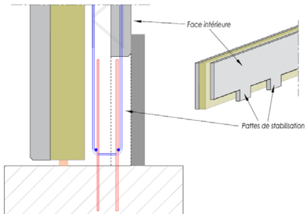
Figure 21 : Encastrement de l'Inov'Mur(i)/radier → Liaison Er2
