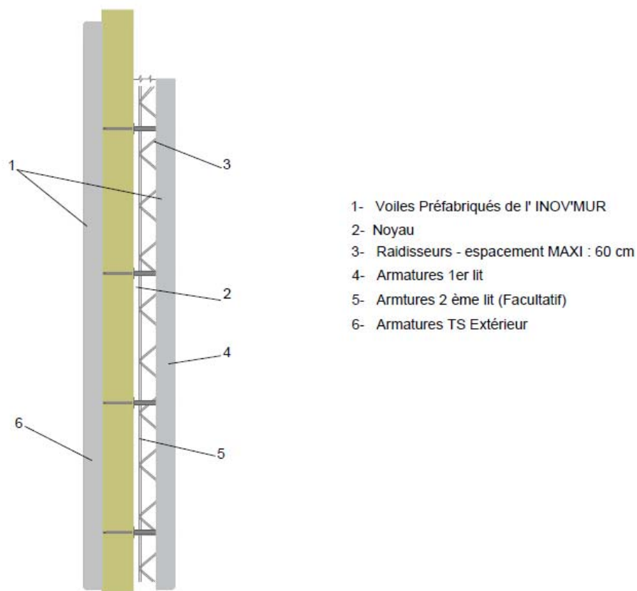
Figure E1.2 : Coupes verticales courantes de l'Inov'Mur (1)
