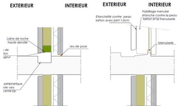
Figure 52b : Balcon sans rupteur de pont thermique.
