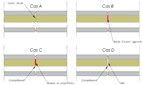
Figure 9 : Isolation au droit des joints pour l'Inov'Mur(i)
