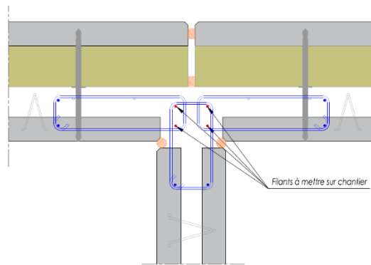
Figure 31 : Liaison verticale en T encastrée - Type Ev5
