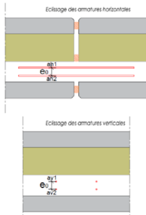
Figure 16 : Eclissage des armatures dans l'Inov'Mur (1)
