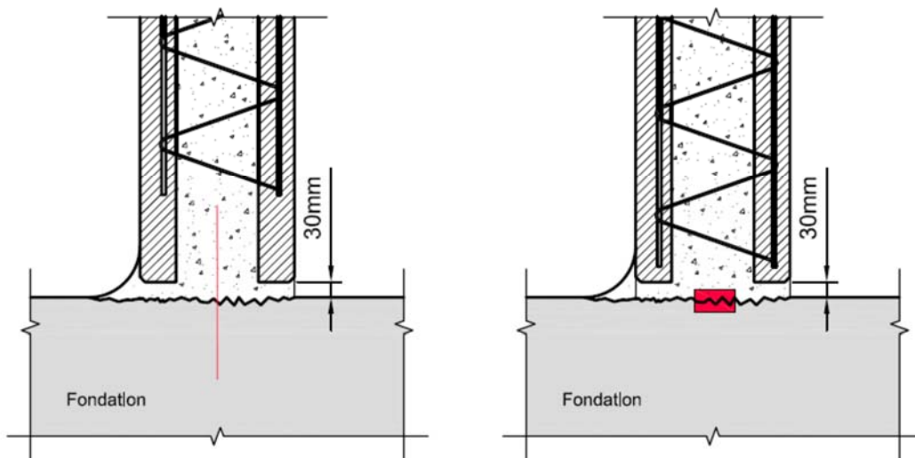
Figure 8 - Dispositifs d'étanchéités spécifiques
