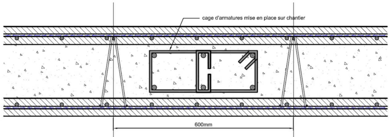
Figure 4 - Poteau en renfort
