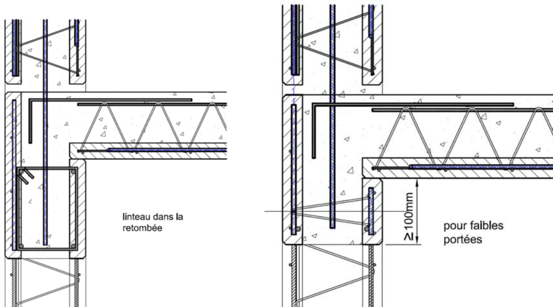
Figure 5 - Linteaux réalisés avec MUR 2000+
