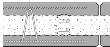
Exemple d'éclissage vertical
