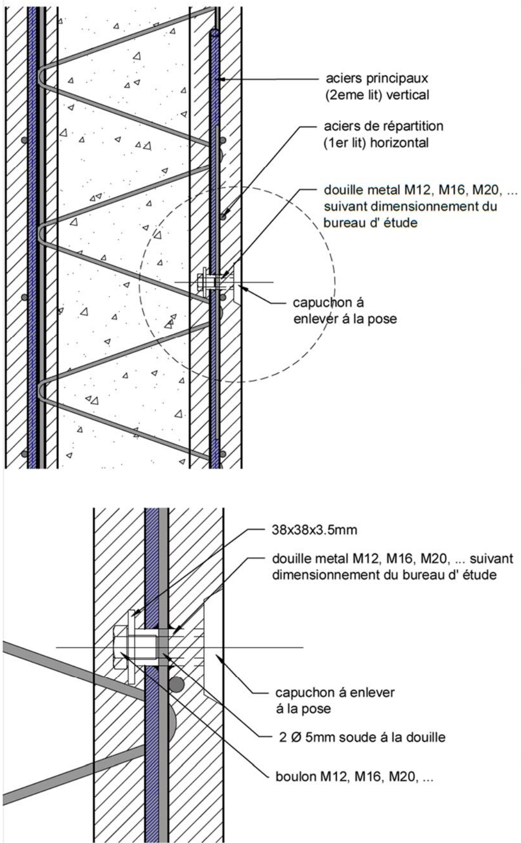
Figure 3 - Douilles de fixations intégrées aux MURS 2000+
