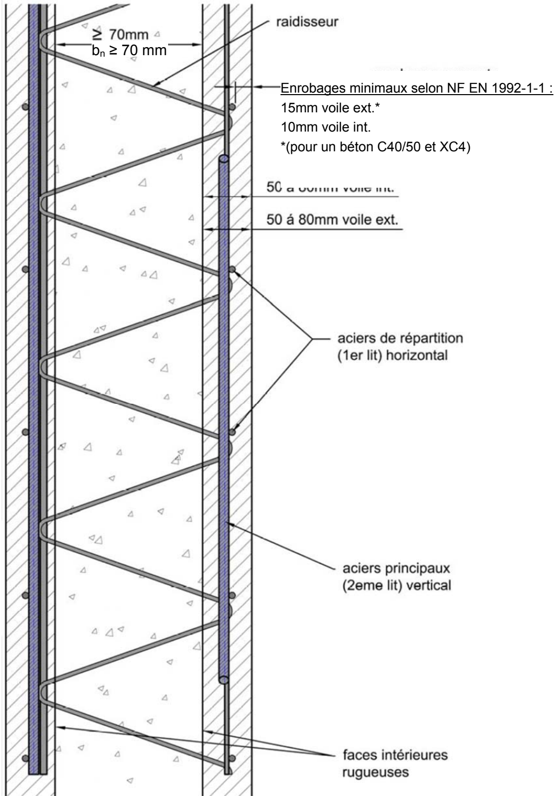
Figure 2 - Principes de ferrailage
