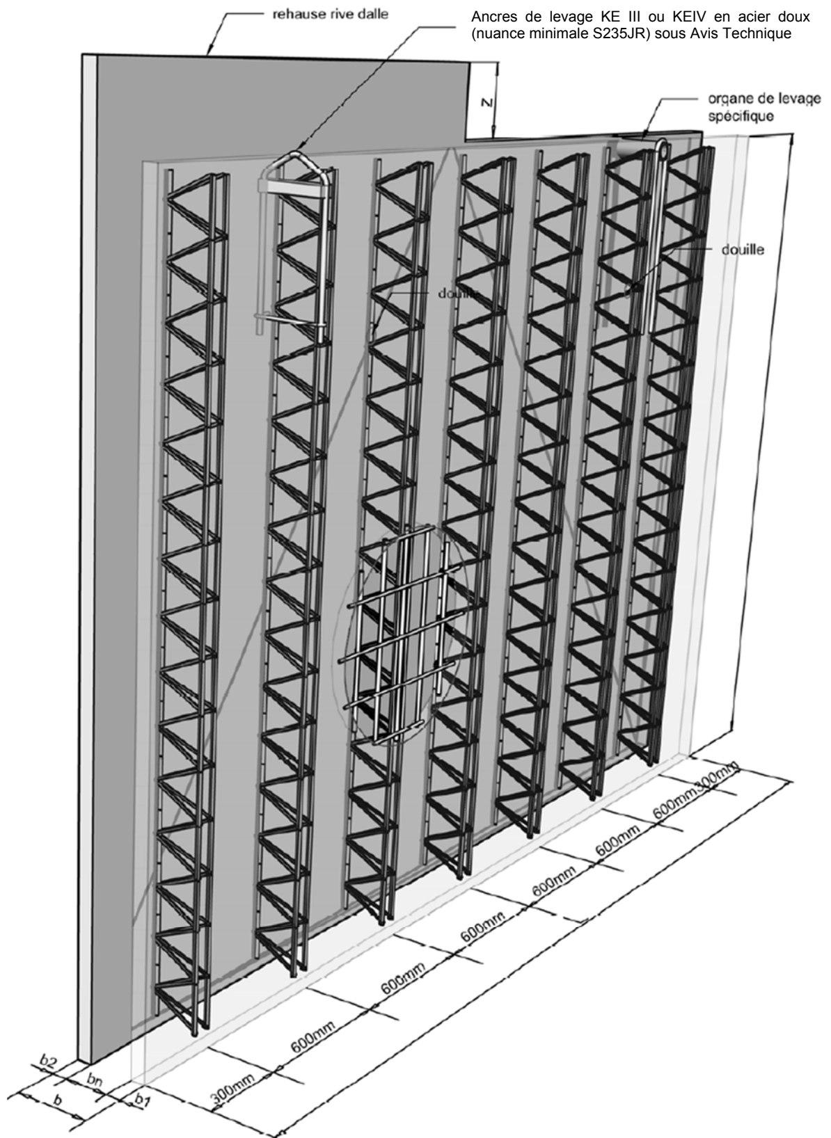
Figure 1 - Principes généraux MUR 2000+
