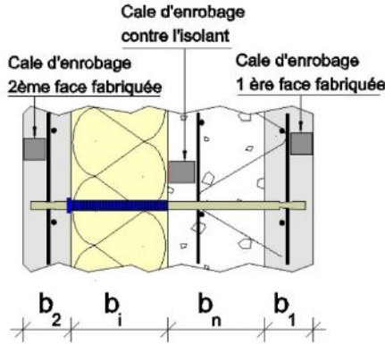
Figure 6 - Positionnement des connecteurs TM90°
