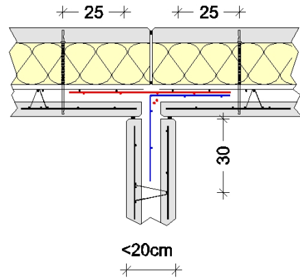
Figure 113 - 1 + 1 lit d'armatures, parois décroisées
