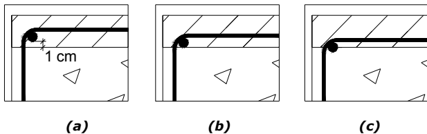
Figure 19 - Enrobage des aciers structuraux et périmètre utile
