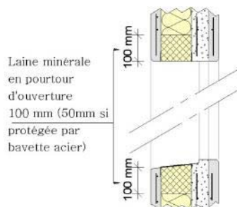
Figure 44 - Laine minérale en pourtour d'ouverture
