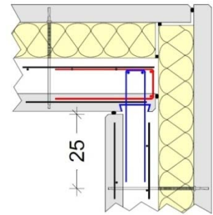
Figure 105 - Liaison par boîte d'attente
