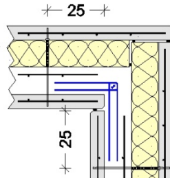
Figure 104 - 2 lits d'armatures de liaison
