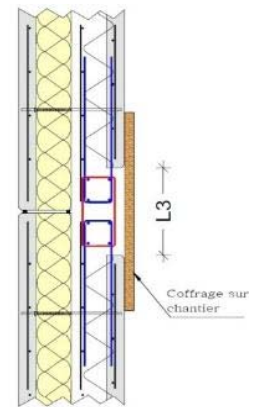
Figure 127 - Solution avec coffrage sur chantier
