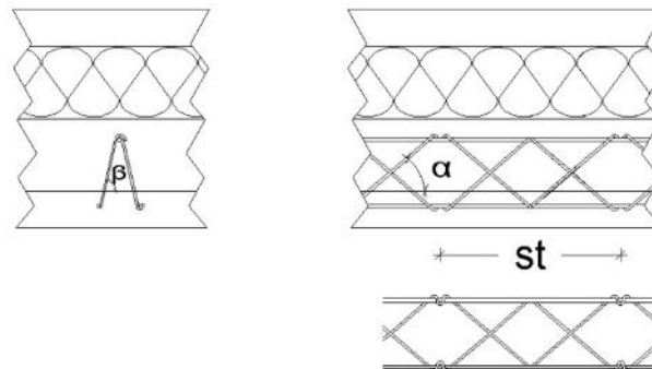
Figure 58 – Géométrie des raidisseurs double sinusoïde
