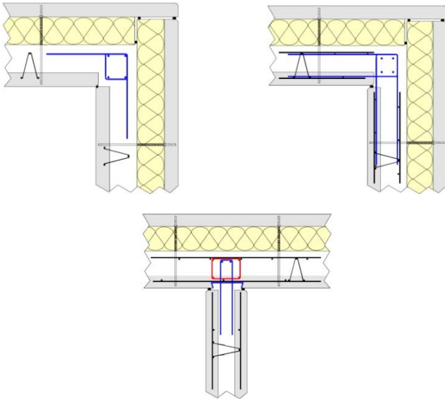
Figure 26 - Exemple d'intersections de mur
