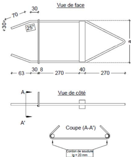
Figure 142 – Détail du boucle de levage
