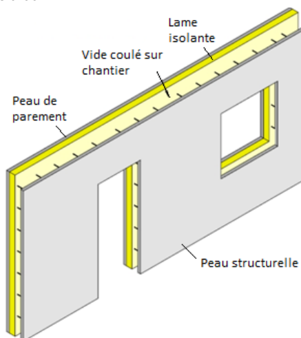
Figure 2 – Exemple d'élément «Duomur Isolant»
