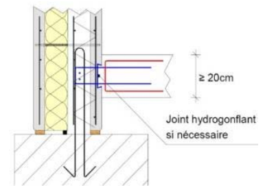
Figure 87 - Liaison couturée avec plancher bas
