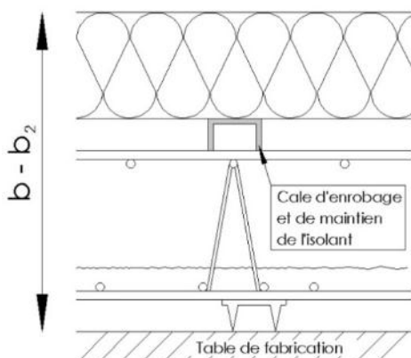
Figure 49 – Cale d'enrobage contre l'isolant
