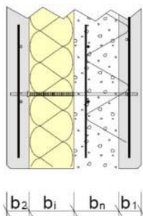
Figure 40 - Section et épaisseurs d'un «Duomur Isolant»
