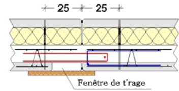
Figure 100 - Liaison couturée
