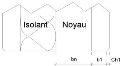
Figure 32 – Définition de géométrie de la section
