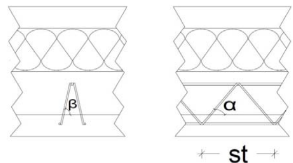
Figure 18 - Géométrie du raidisseur
