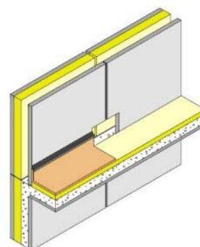
Partie haute fractionnée, partie basse continue
