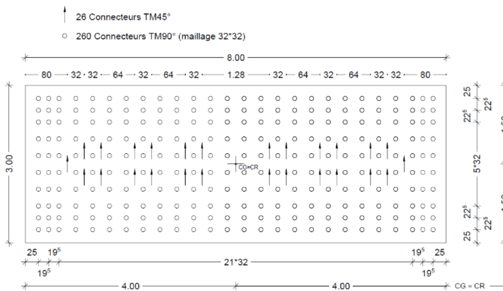
Figure 141 – Exemple de disposition de connecteur zone sismique 3
