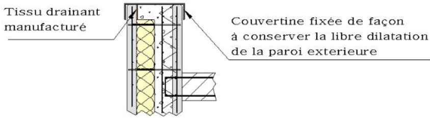
Figure 66 – Tête de «Duomur Isolant»
