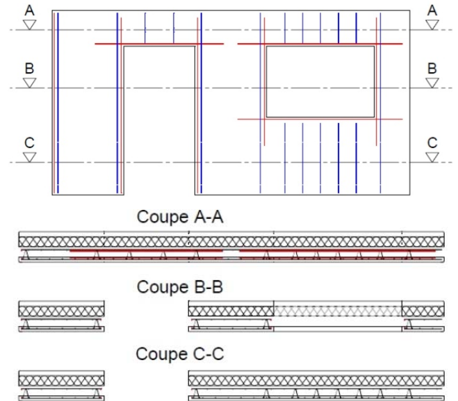
Figure 17 - Dispositions équivalentes de renforcement des bords libres verticaux solution «Duomur Isolant»
