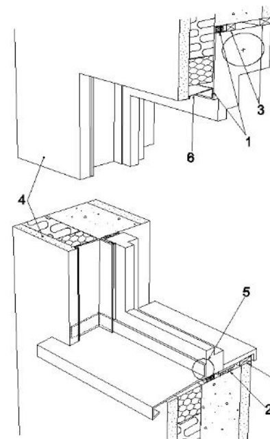
Figure 48 – Exemple de mise en place de volet roulant
