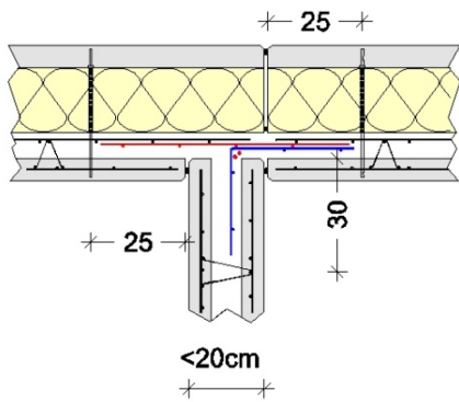
Figure 112 - 1 + 1 lit d'armatures, parois croisées
