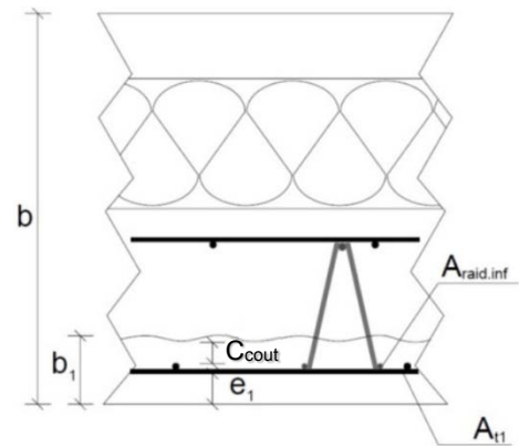
Figure 15 - Définition des chaînes de cotes
