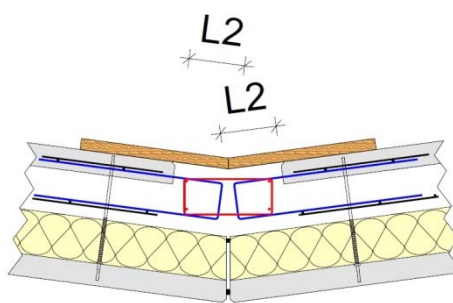
Figure 110 - Angles > à 165° L2 = 32 Ø + 7 cm
