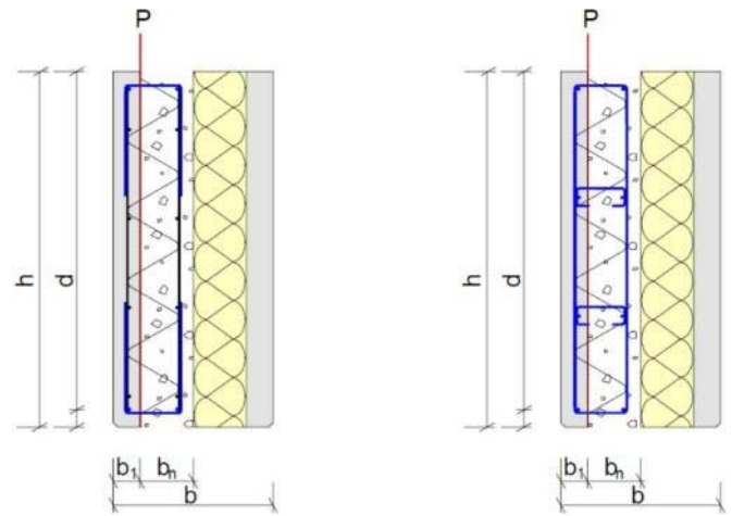
Figure 31 - Plans de cisaillement dans la section d'une poutre
