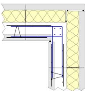
Figure 109 - «Duomur Isolant» posé avant réalisation du support
