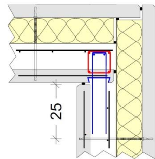
Figure 108 - Liaison par boîte d'attente
