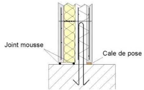
Figure 28 - Liaisons en pied de murs courants
