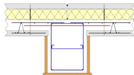
Figure 79 - Poteau excentré coulé en place au droit 'un joint vertical
