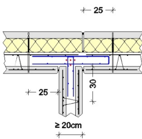
Figure 116 - 2 + 2 lits d'armatures, parois croisées
