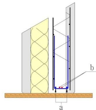
Figure 129 - Tirants intégrés au «Duomur Isolant» avec joint vertical
