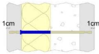
Figure 13 - Retrait minimum des connecteurs : 1 cm
