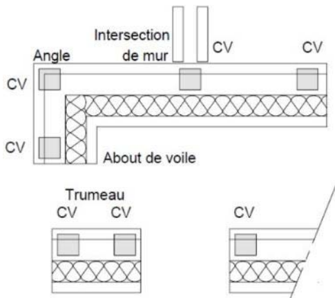
Figure 27 - Implantation type des chaînages verticaux CV
