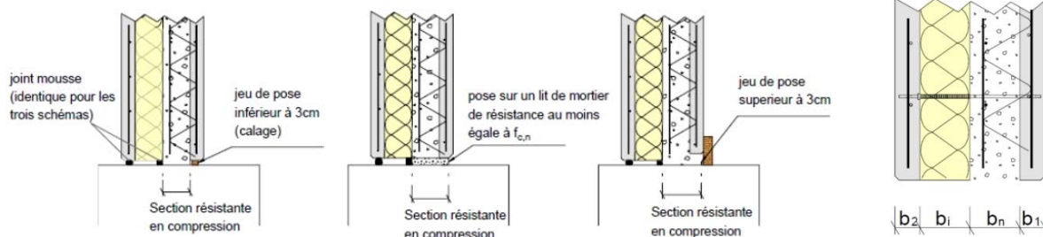
Figure 12 - Exemple de section résistante en compression
