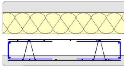
Figure 83 - Raidisseurs + U de fermeture
