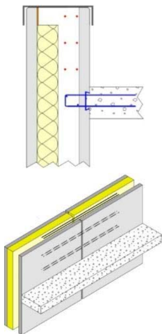
Eclisses mises en place dans le noyau
