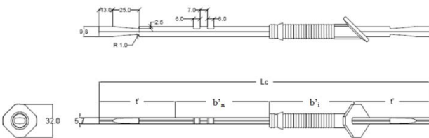
Figure 7 - Détail d'un connecteur TM45°
