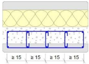
Figure 30 - Section de poteau nécessitant des armatures structurales
