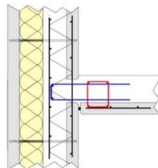
Figure 95 - Plancher suspendu avec attentes mises sur chantier
