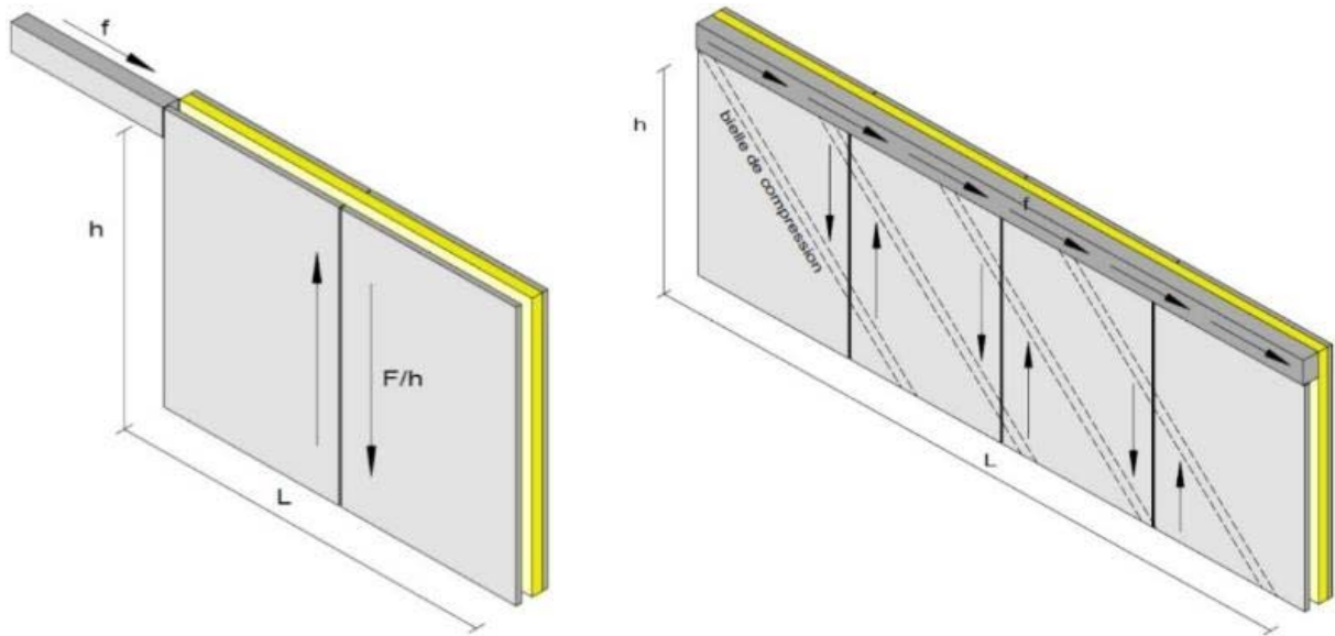
Figure 52 – Effort sollicitant dans le cas d'un contreventement
