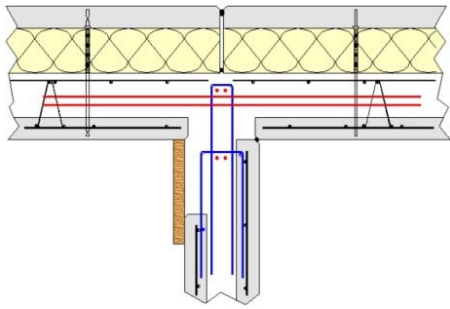
Figure 119 - Coffrage de la face intérieure
