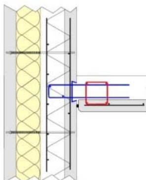
Figure 94 - Plancher suspendu avec boîte d'attente. Celles-ci doivent respecter les dispositions de l'annexe F de la section A du prCPT "PLANCHERS" TITRE II (édition décembre 2014)
