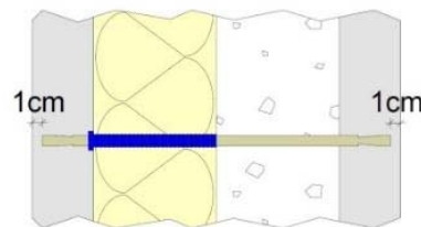
Figure 11 – Enrobage nominal des connecteurs
