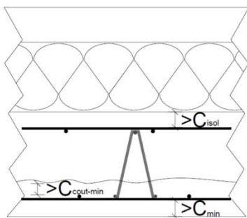
Figure 14 - Définition des enrobages
