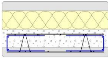
Figure 29 - Section de poteau résistant par le béton seul
