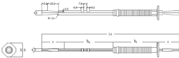
Figure 5 - Détail d'un connecteur TM90°
