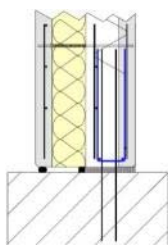
Figure 88 - Pose sur lit de mortier
