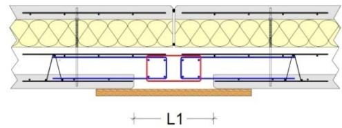
Figure 102 - Coffrage d'une face sur chantier solution avec ou sans aciers en attente
