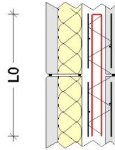
Figure 124 - 2 lits d'armatures verticales L0 = 2ls + 15 \text{ cm}
