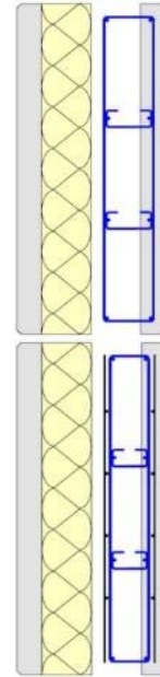
Figure 82 - Cadres + épingles
