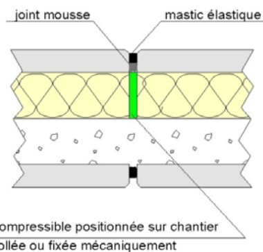
Figure 43 - Jonction entre épaisseurs isolantes
