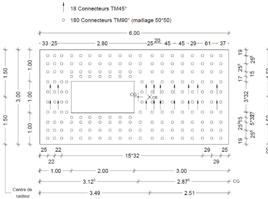
Figure 140 – Exemple de disposition de connecteur zone sismique 3
