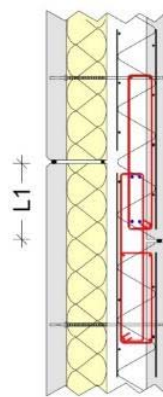
Figure 126 - Solution avec décalage de parois
