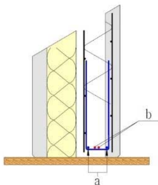
130 - Tirants inférieurs mis en place sur chantier avec ou sans joint vertical. a et b : tirants inférieurs
