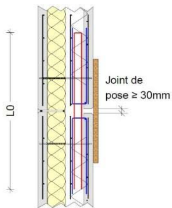
Figure 125 - Jeu de pose \geq 30 mm L0 = 2ls + 15 cm
