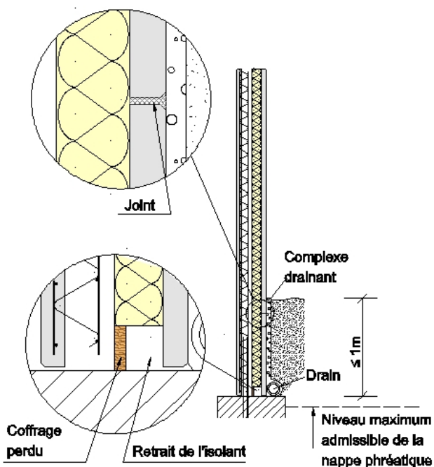
Figure 41 - Murs semi enterrés faible hauteur
