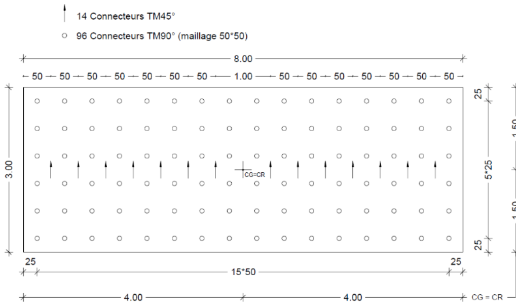
Figure 139 – Exemple de disposition de connecteur zone sismique 1
