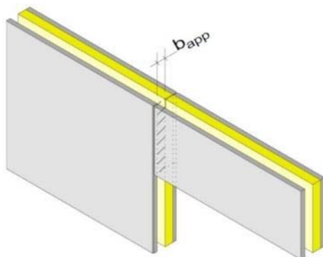
Figure 33 - Appui de poutre – cas 1
