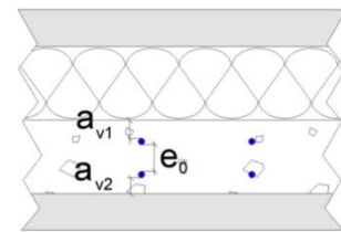
Figure 22 - Exemple de l'éclissage des armatures verticales
