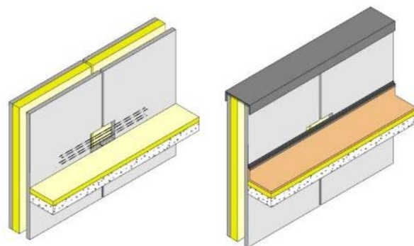
Partie haute fractionnée, partie basse continue
