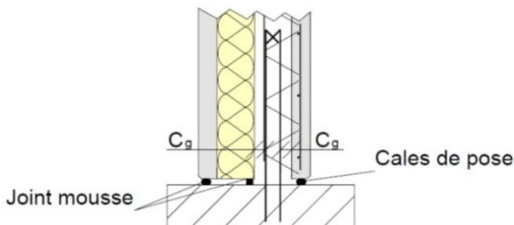
Figure 20 - Position des aciers en attente dans un «Duomur Isolant»
