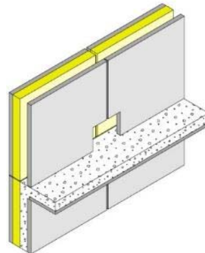
Figure 39 - Détail de réalisation du fractionnement des acrotères hauts
