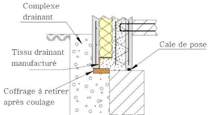
Figure 67 – Pied de murs protégé par le béton de remplissage
