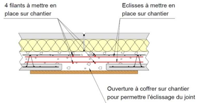
Figure 25 - Liaison verticale en zone sismique sans justification par le calcul
