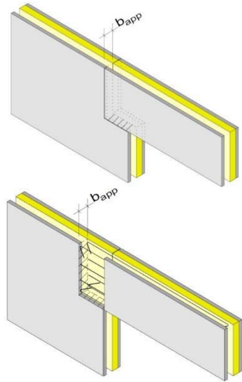
Figure 34 - Appui de poutre – cas 2
