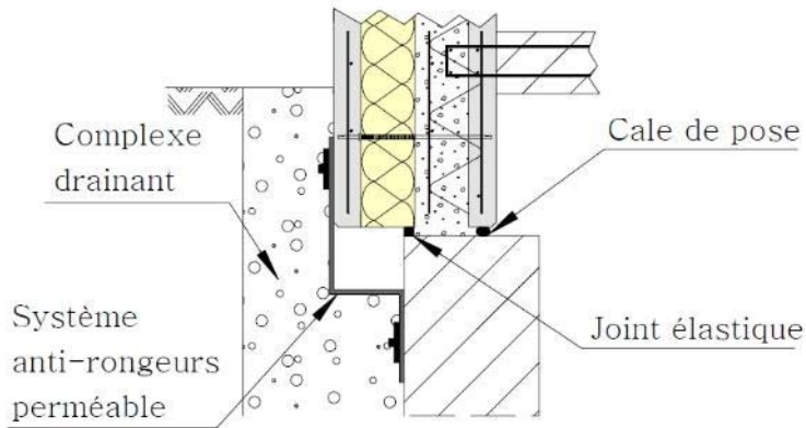
Figure 67 – Pied de mur protégé par système anti-rongeur
