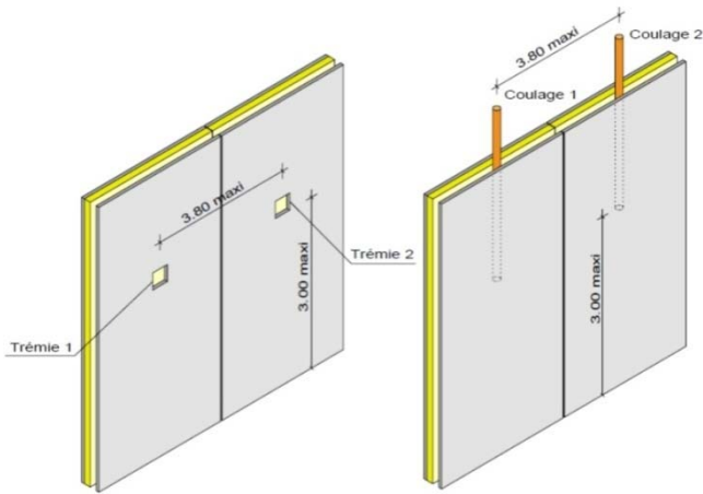
Figure 23 - Hauteur de bétonnage équivalente à (a) hauteur sous trémie et (b) hauteur sous tube souple
