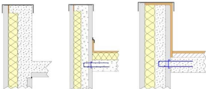
Figure 35 - Protection de l'étanchéité
