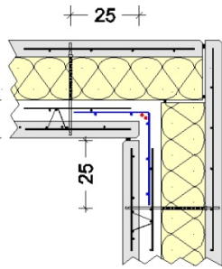
Figure 103 - 1 lit d'armatures de liaison
