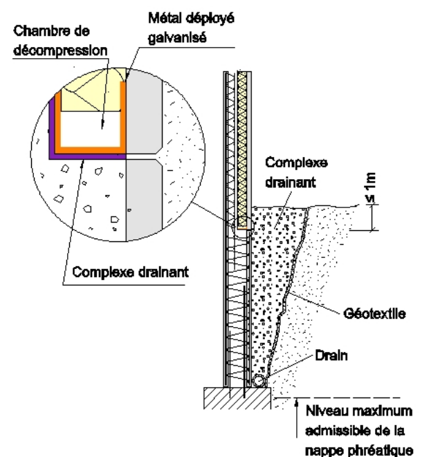
Figure 42 - Murs semi enterrés hauteur importante
