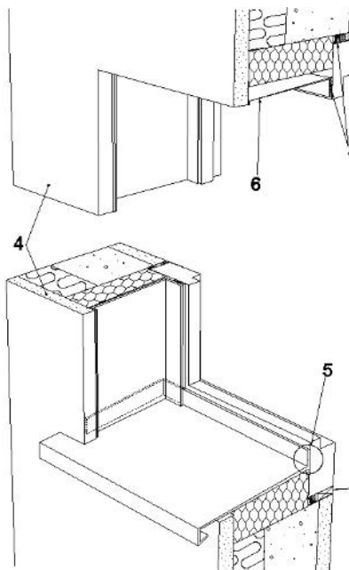
Figure 47 – Exemple de menuiserie au nu intérieur du «Duomur Isolant»
