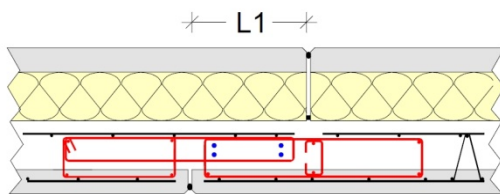
Figure 101 - «Duomur Isolant» posé avant réalisation du support
