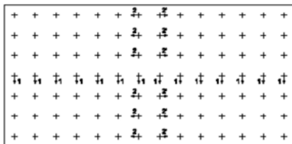
Figure 10 – Exemple de disposition des connecteurs TM
