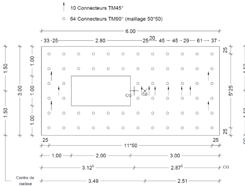
Figure 138 – Exemple de disposition de connecteur zone sismique 1
