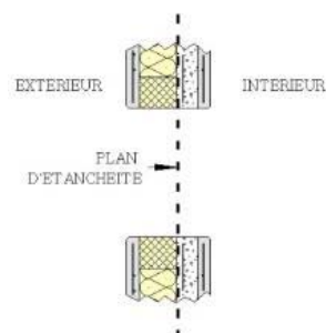
Figure 45 - Plan d'étanchéité de la façade
