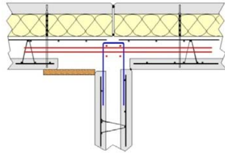
Figure 120 - Coffrage face intérieure, sollicitations importantes
