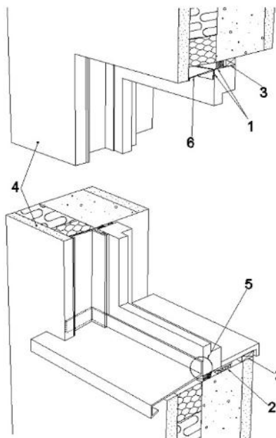
Figure 46 – Exemple de menuiserie à l'interface isolant/béton de remplissage
