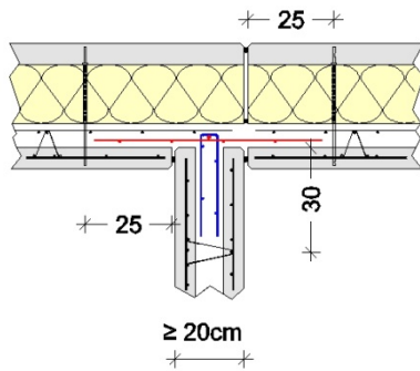
Figure 114 - 1 + 2 lits d'armatures, parois croisées
