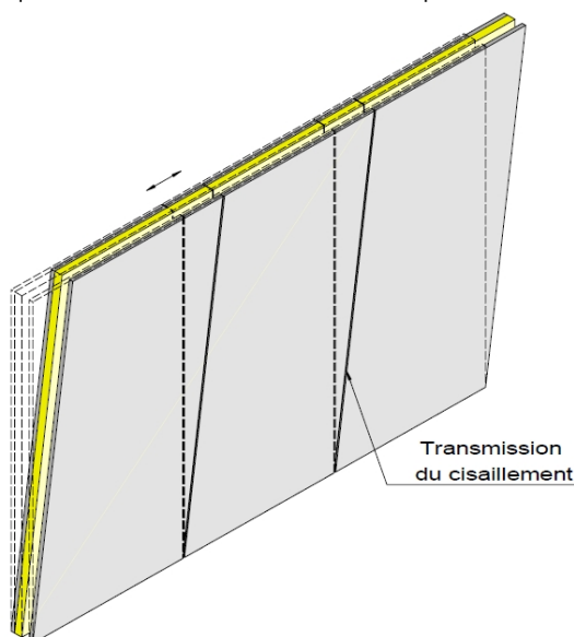
Figure 24 - Schéma d'un comportement monolithique des panneaux
