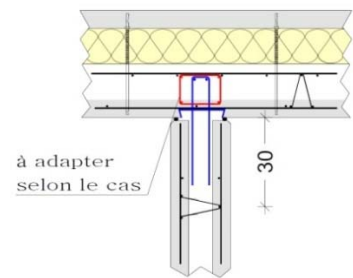
Figure 118 - Liaison par boîte d'attente
