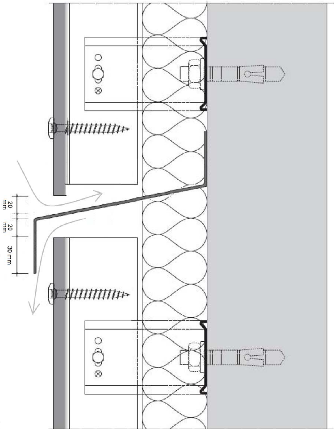
Figure 10 – Fractionnement de la lame d'air
