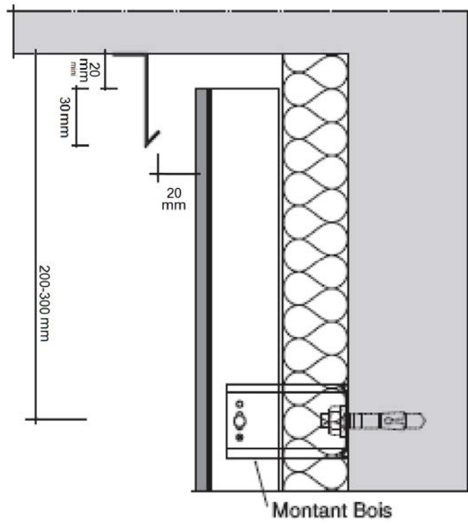
Figure 14 – Arrêt haut sous acrotère
