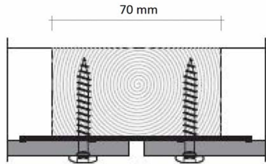
Figure 4 – Coupe verticale sur joint horizontal (joint fermé)
