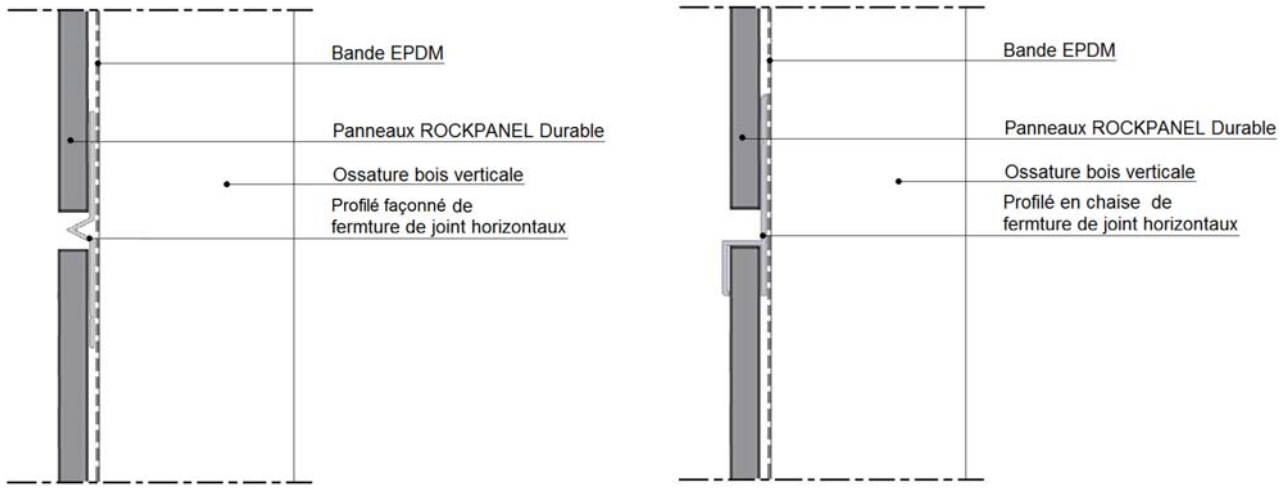
Figure 25 – Joint horizontal fermé COB supérieure à 10 m
