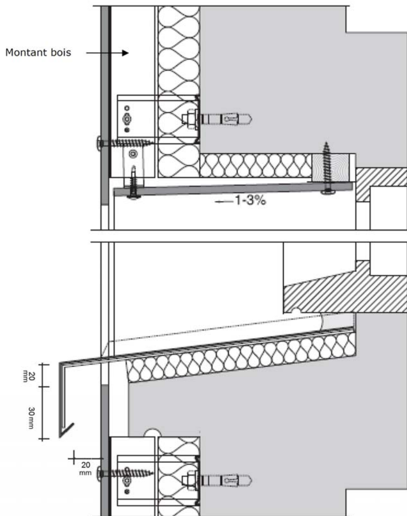
Figure 20 – Coupe verticale sur baie
