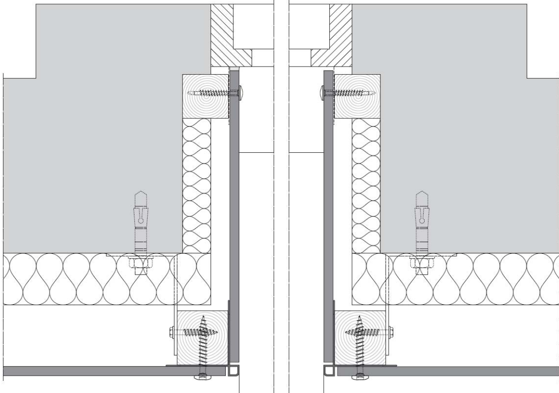
Figure 19 – Habillage latéral de baie
