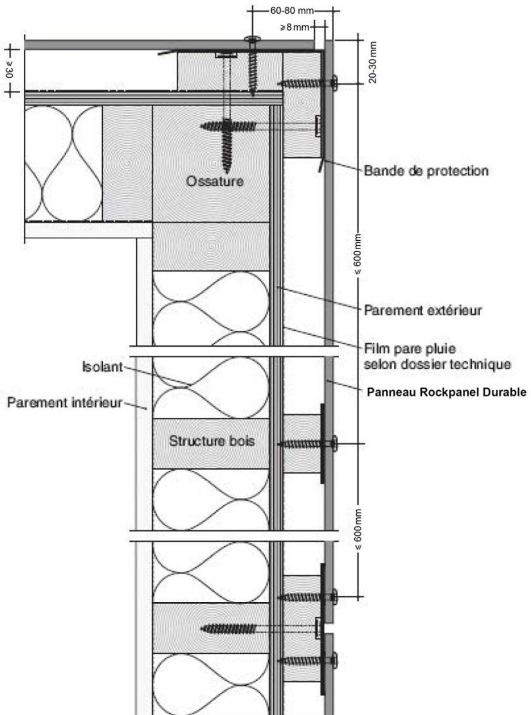
Figure 24 – Pose sur COB
