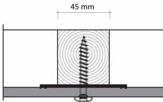
Figure 3 – Coupe verticale sur joint horizontal (joint ouvert)
