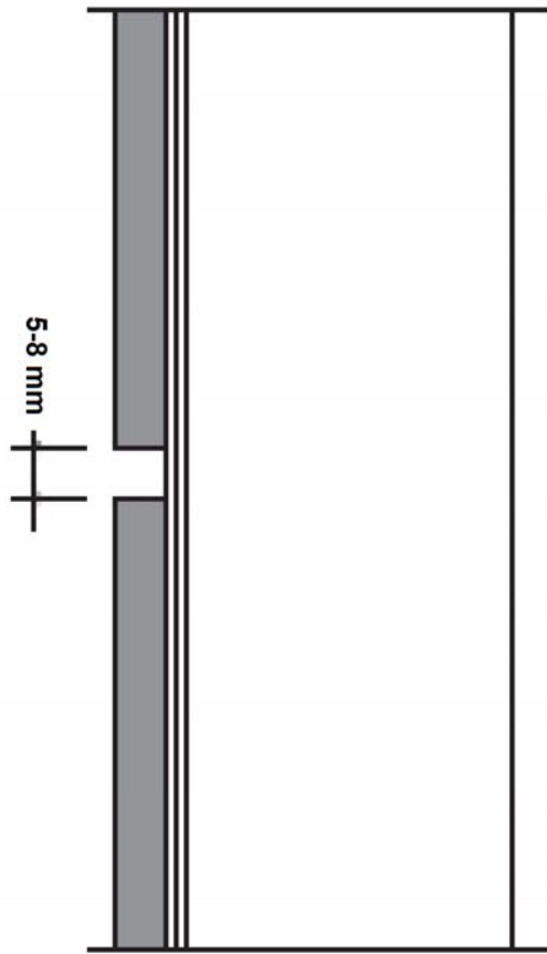
Figure 3 – Coupe verticale sur joint horizontal (joint ouvert)
