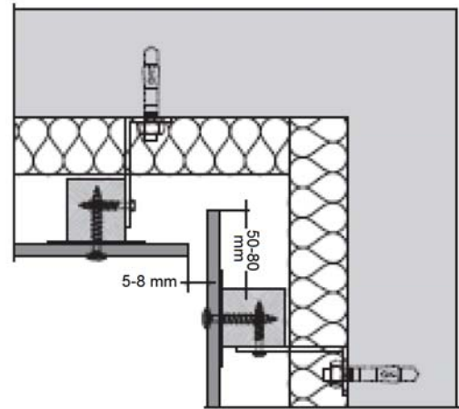
Figure 16 – Angle rentrant sans profilé
