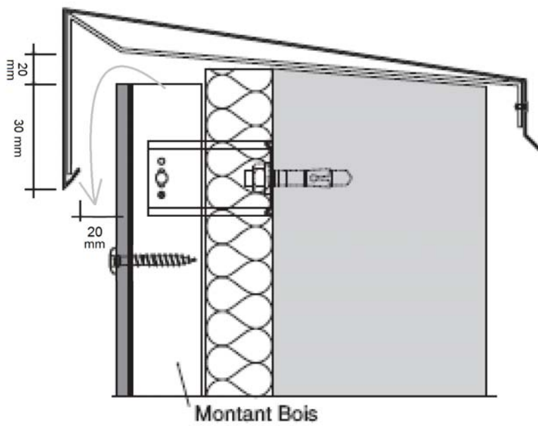
Figure 13 – Arrêt haut avec couvertine
