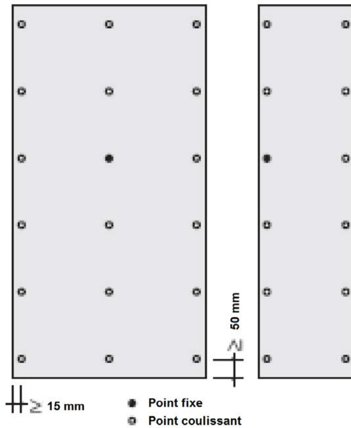
Figure 2 – Exemple de positionnement de points fixes (format 1200 x 2000 mm)
