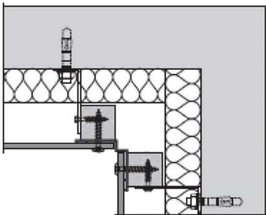
Figure 15 – Angle rentrant avec profilé
