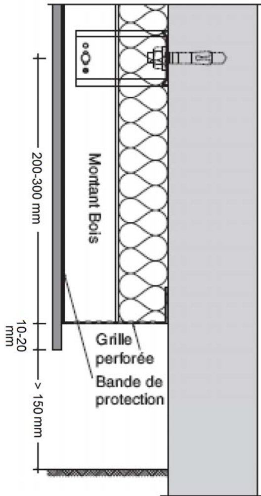
Figure 12 – Départ de balcon privatif
