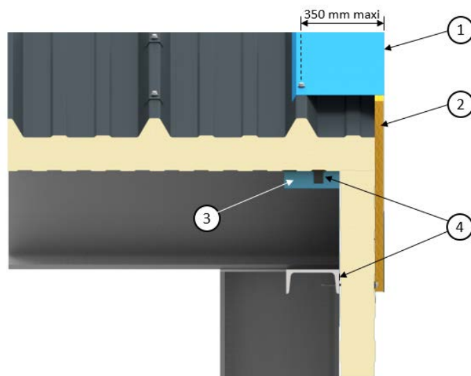
Figure 9 – haut de bardage, en pose horizontale
