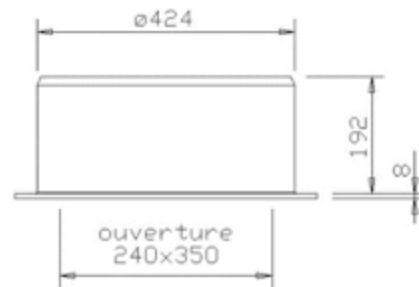
Figure 9a – Détail d'un puits d'inspection et d'un puits de ventilation pour bassin à une couche de modules WAVIN Q-Bic Plus LC sous espace verts
