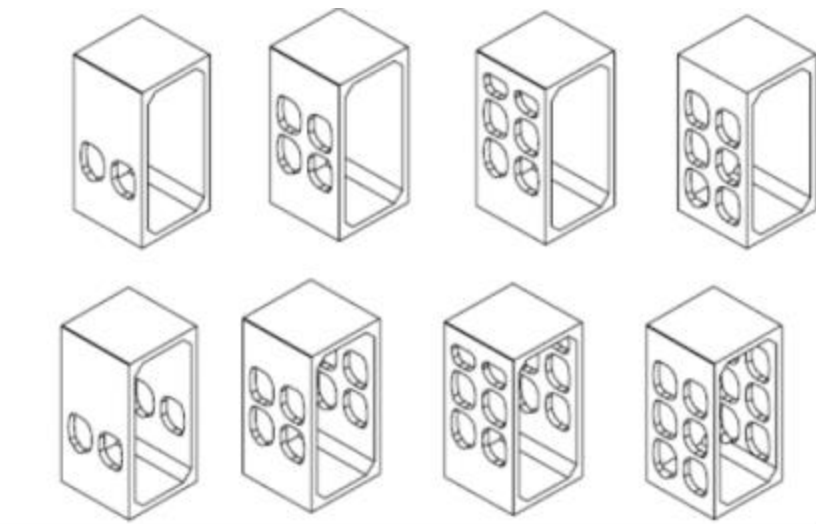
Figure 11 - Caractéristiques dimensionnelles des cadres
