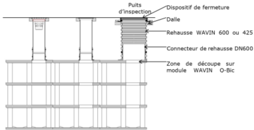
Figure 9c - Coupe de principe ouvrage WAVIN Q-Bic Plus LC intégrant puits d'inspection intégré, modules à canaux de curage WAVIN Q-Bic Plus LC et regard de sortie
