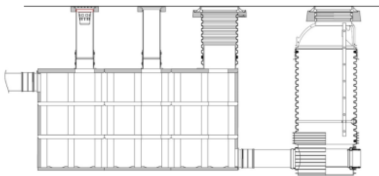
Figure 10 - Gamme de cadres pour la réalisation de la galerie d'accès
