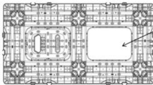
Figure 8a – Connecteur de rehausse DN/ID 600
