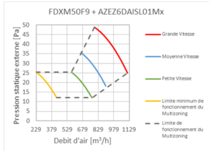
Figure 14 – Unité intérieure FDXM50F9 Courbes débit/pression
