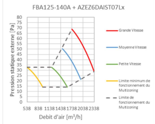
Figure 8 – Unités intérieures FBA125A et FBA140A Courbes débit/pression
