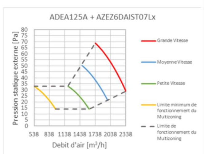
Figure 12 – Unité intérieure ADEA125A Courbes débit/pression
