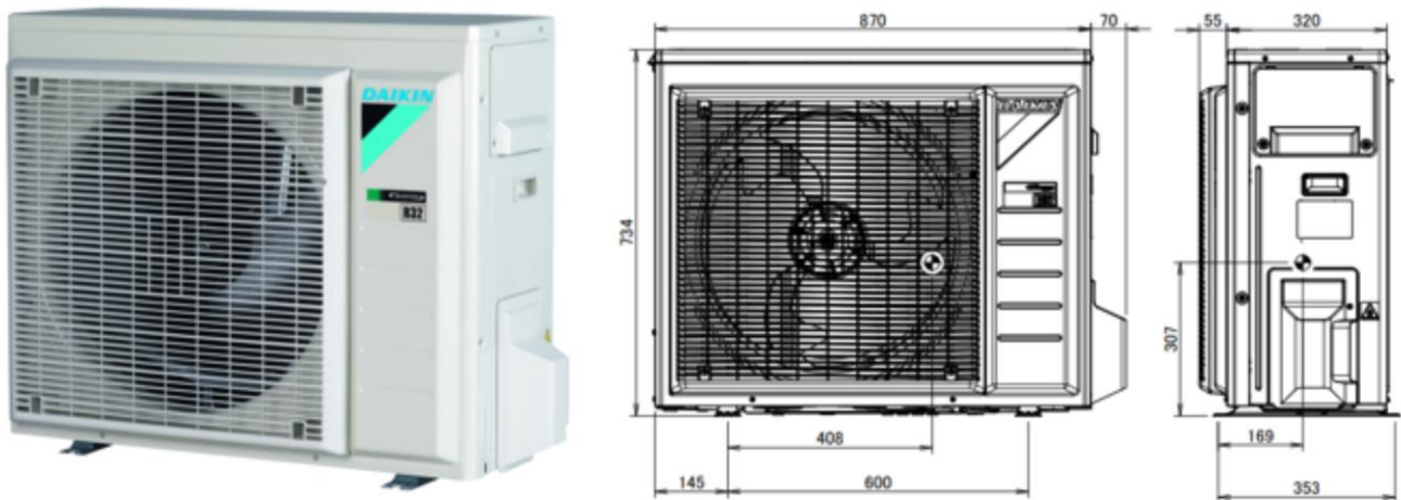
Figure 2 – Unités extérieures thermodynamiques RXM50R – visuel et caractéristiques dimensionnelles
