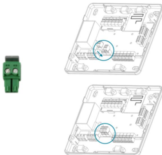
Figure 7 – Schéma d'inhibition de la fonction rafraîchissement via l'accessoire AZX6MCS
