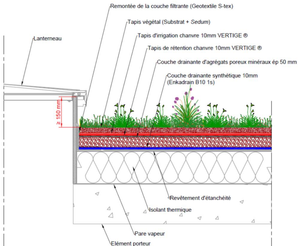
Figure 21 - Coupe sur émergence en toiture sur élément porteur en maçonnerie de pente comprise entre 0 et 2 % sans couche de substrat complémentaire (VERTIGE® EXTENSIF ORIGINAL)
