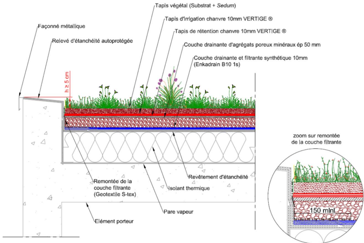
Figure 12 - Coupe type sur relevé (sans zone stérile), élément porteur en maçonnerie, 0 \% \leq \text{pente} < 2 \% , (VERTIGE® EXTENSIF ORIGINAL)
