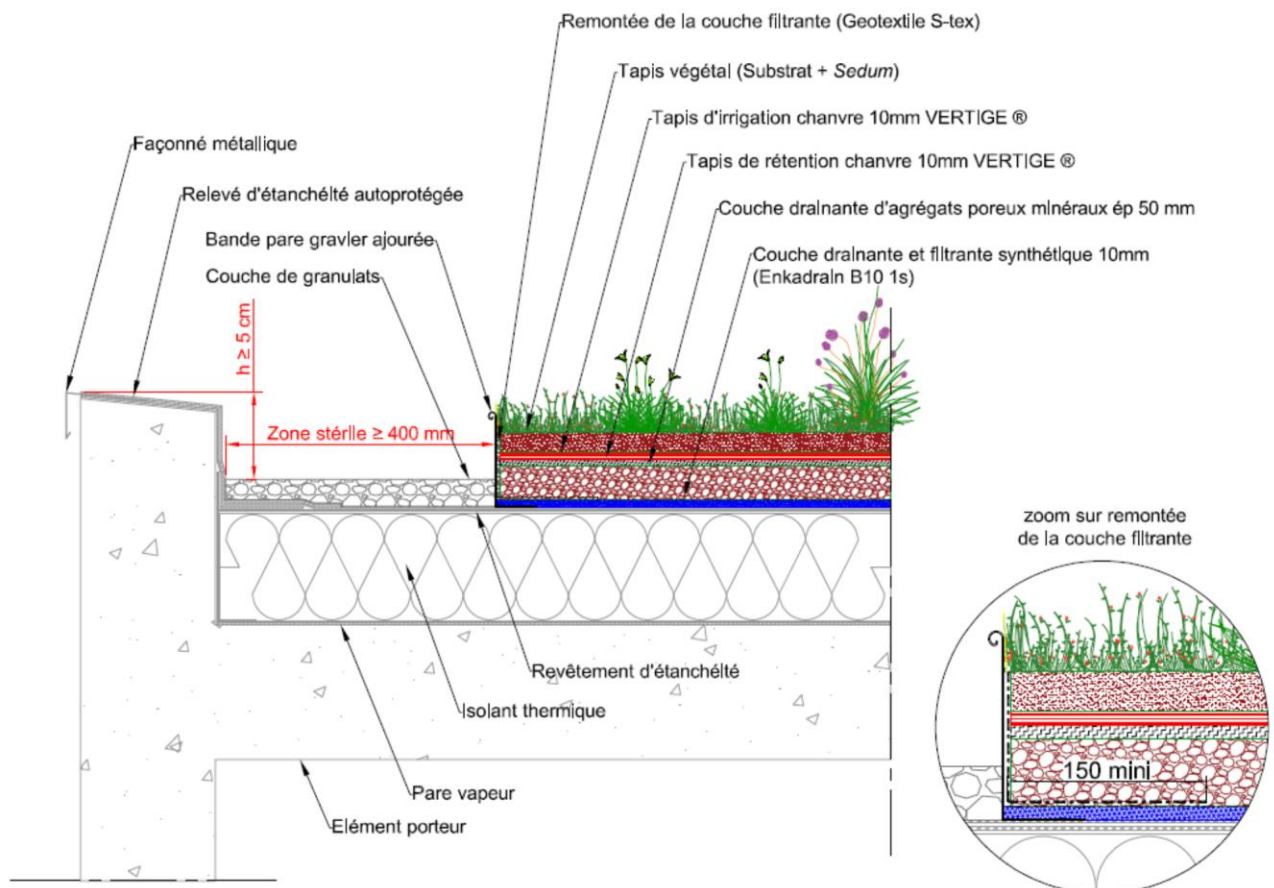
Figure 11 - Coupe type sur relevé avec zone stérile, élément porteur en maçonnerie, 0\% \leq \text{pente} < 2\% , (VERTIGE® EXTENSIF ORIGINAL)
