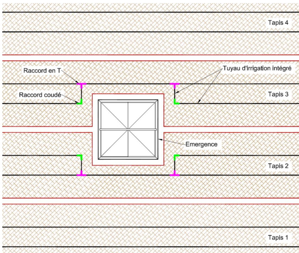
Figure 23 - Schéma de principe du système d'irrigation - Contournement d'une émergence en toiture - cas 2
