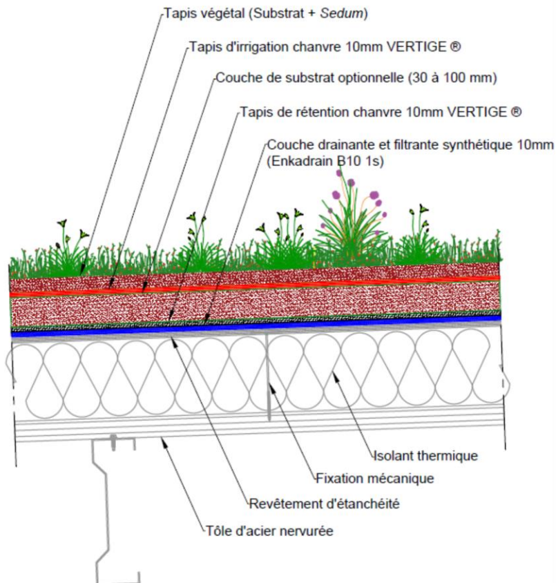
Figure 17 - Coupe en partie courante sur élément porteur en tôle d'acier nervurée de pente comprise entre 3 % et 20 % avec couche de substrat complémentaire d'épaisseur 3 à 9 cm, ou de pente comprise entre 3 % et 5 % avec couche de substrat d'épaisseur jusqu'à 6 cm
