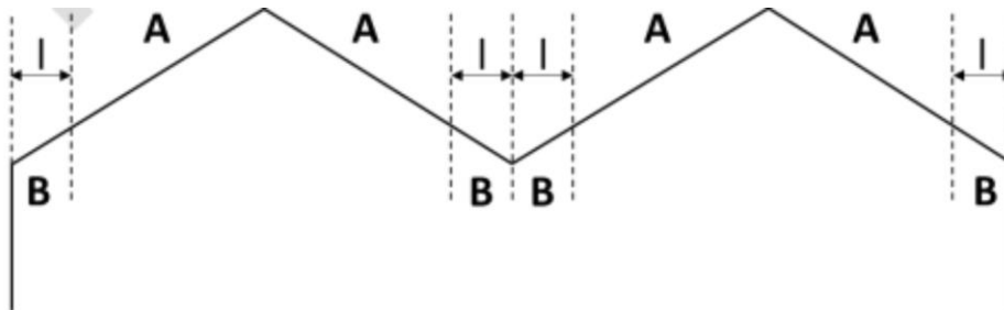
Figure 8 - Principe des zones de la toiture suivant les pentes (dessin sans échelle)
