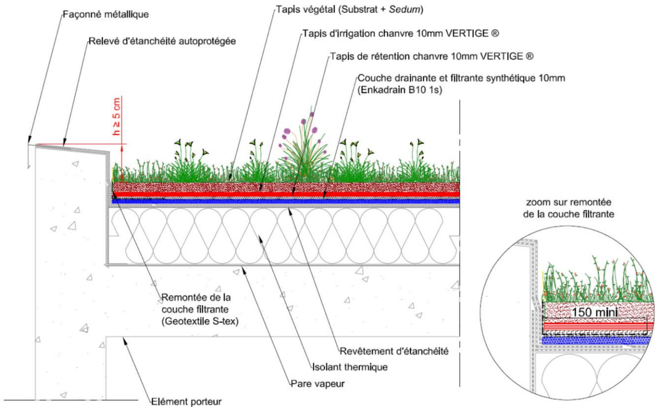
Figure 14 – Coupe type sur relevé (sans zone stérile), élément porteur en maçonnerie, de pente comprise entre 2 % et 20 %, sans couche de substrat complémentaire, (VERTIGE® EXTENSIF ORIGINAL)
