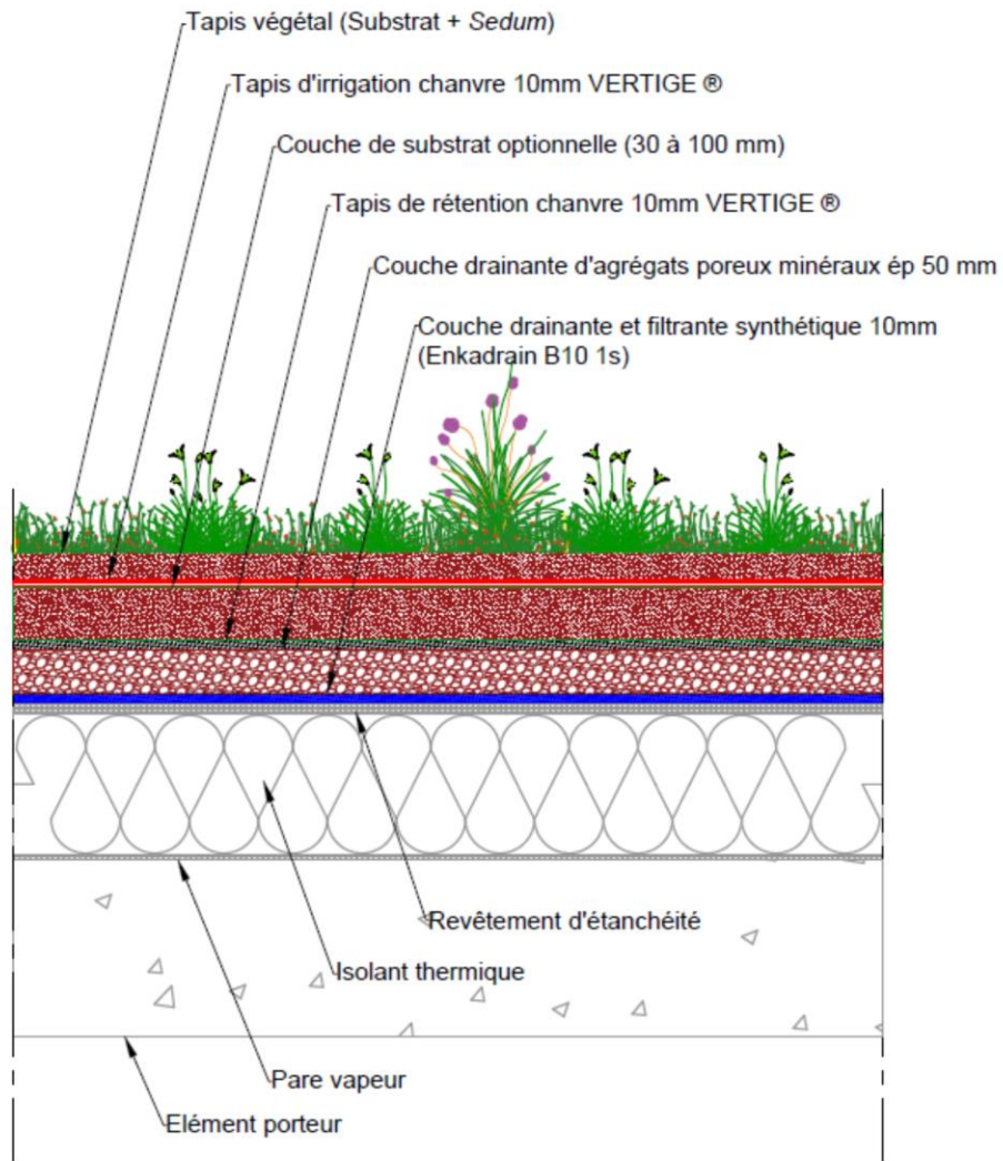
Figure 19 - Coupe en partie courante sur élément porteur en maçonnerie de pente comprise entre 0 et 2 % avec couche de substrat complémentaire d'épaisseur 3 à 9 cm
