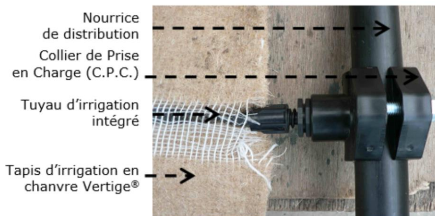
Figure 5 - Détail de raccordement entre la nourrice de distribution et le tapis du système d'irrigation Vertige®
