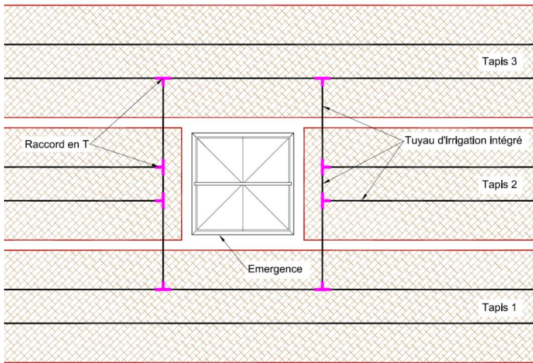
Figure 22 - Schéma de principe du système d'irrigation - Contournement d'une émergence en toiture - cas 1
