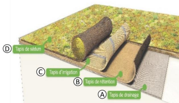
Figure 1 - Complexe de végétalisation Vertige® (EXTENSIF ORIGINAL)
