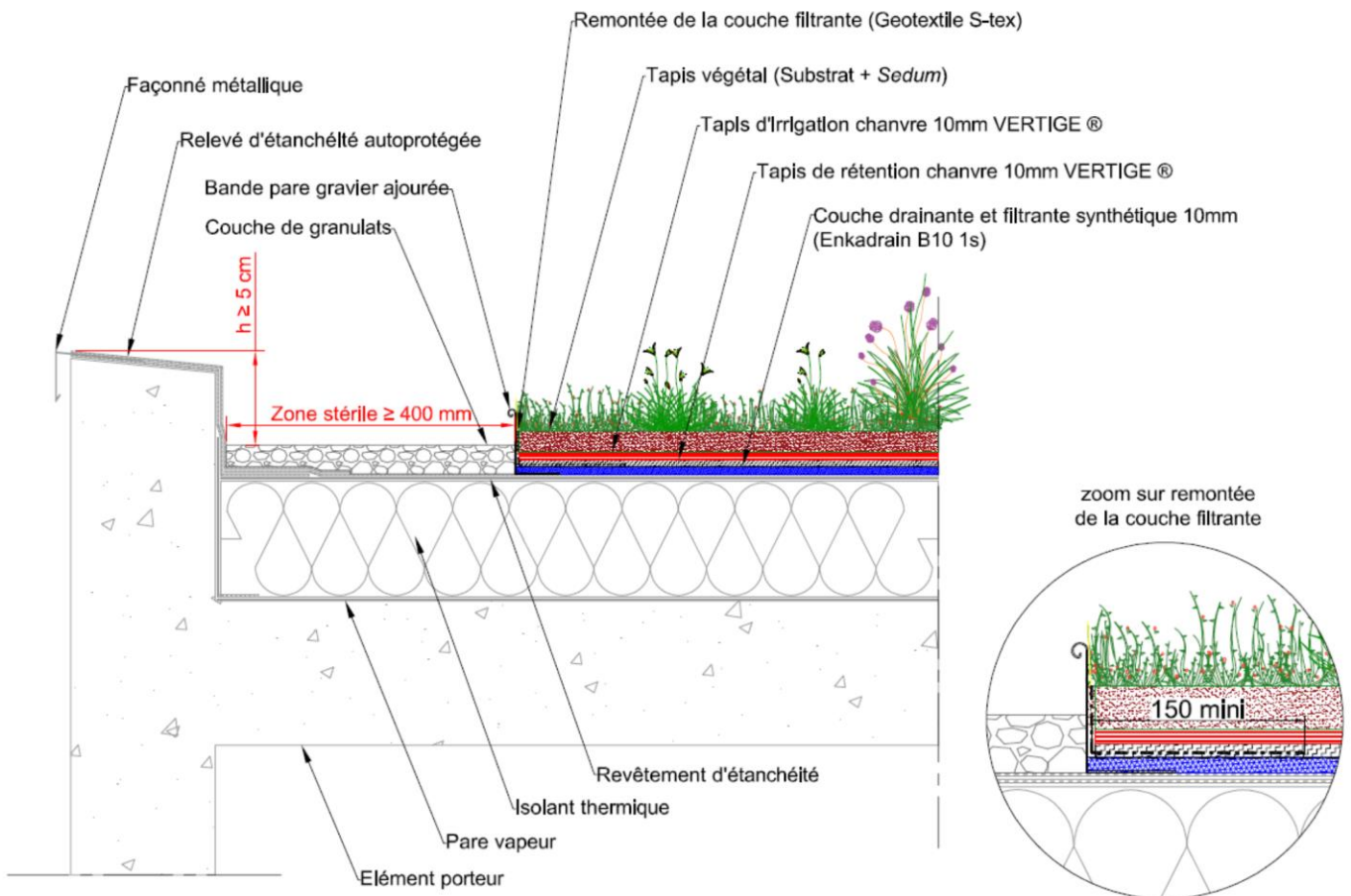
Figure 13 - Coupe type sur relevé avec zone stérile, élément porteur en maçonnerie, de pente comprise entre 2 % et 20 %, sans couche de substrat complémentaire, (VERTIGE® EXTENSIF ORIGINAL)
