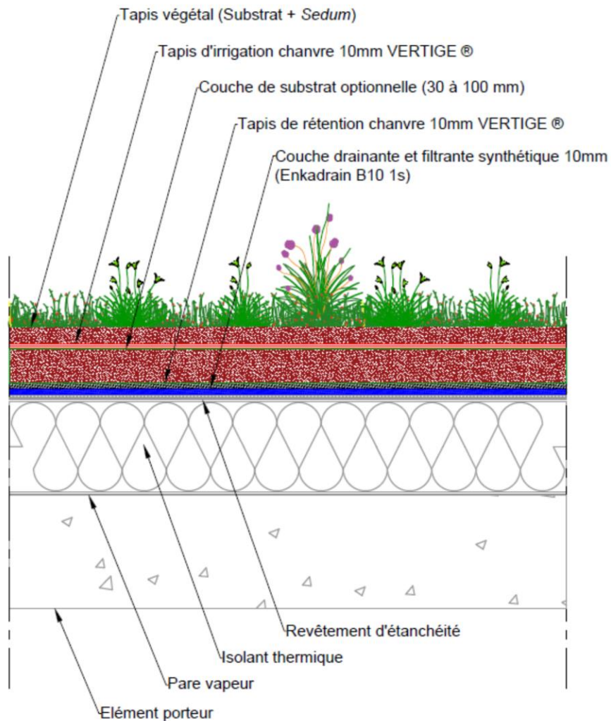
Figure 18 - Coupe en partie courante sur élément porteur en maçonnerie de pente entre 2 % et 20% avec couche de substrat complémentaire d'épaisseur 3 à 9 cm, ou de pente comprise entre 2 % et 5 % avec couche de substrat d'épaisseur jusqu'à 6 cm
