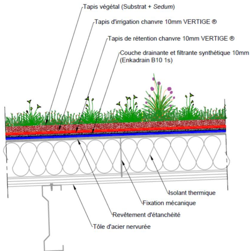
Figure 15 – Coupe type en partie courante sur élément porteur tôle d'acier nervurée de pente comprise entre 3 % et 20 %, sans couche de substrat complémentaire, (VERTIGE® EXTENSIF ORIGINAL)
