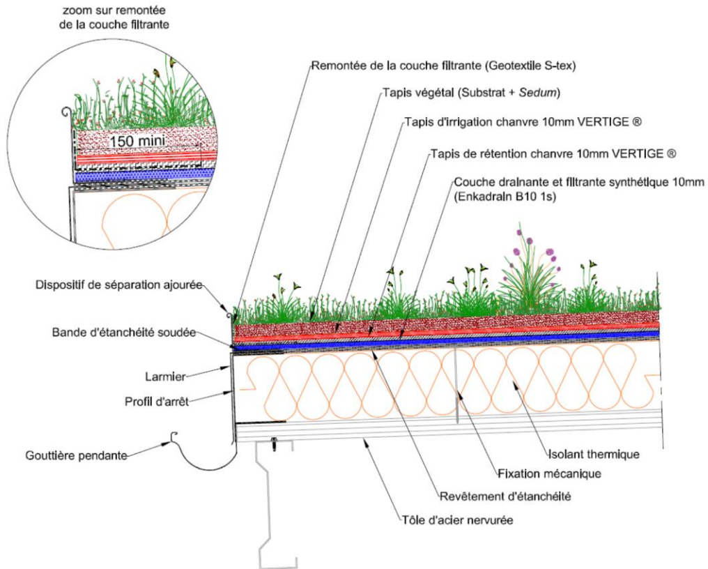
Figure 16 – Coupe type en rive courante sur élément porteur tôle d'acier nervurée de pente comprise entre 3 % et 20 %, sans couche de substrat complémentaire, (VERTIGE® EXTENSIF ORIGINAL)
