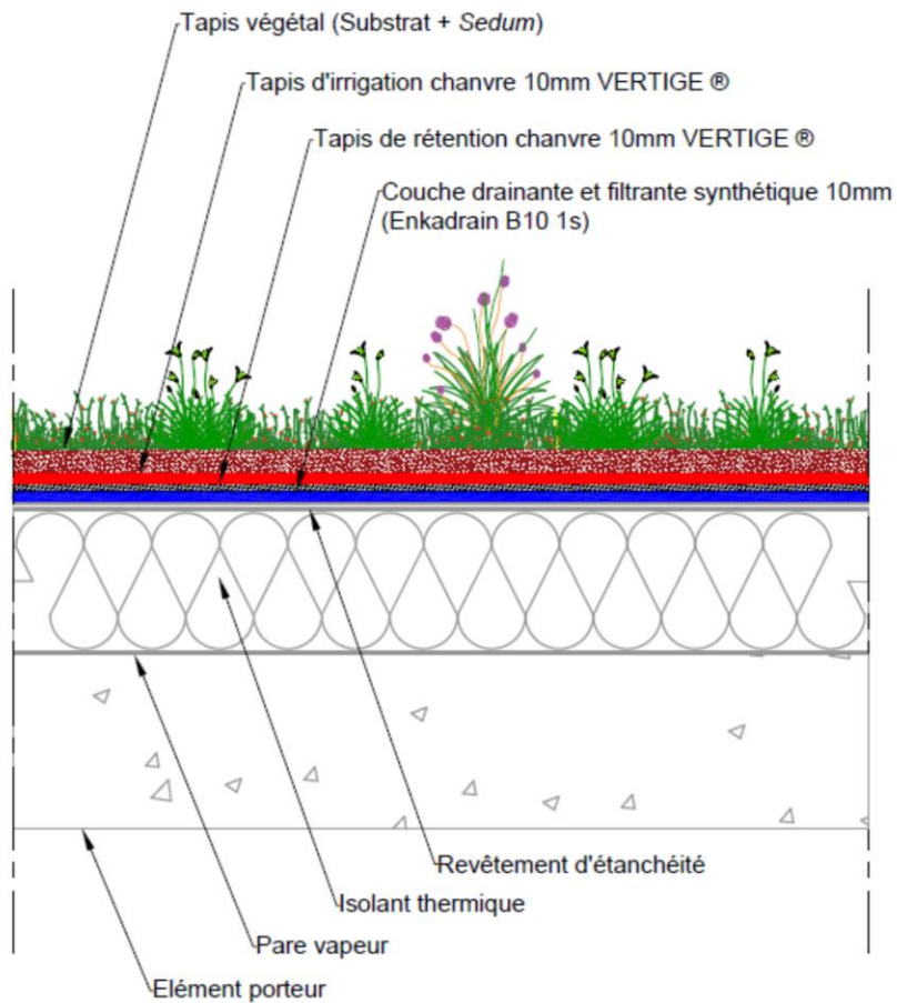
Figure 10 - Coupe en partie courante sur élément porteur en maçonnerie de pente \geq 2\% , sans couche de substrat complémentaire (VERTIGE® EXTENSIF ORIGINAL)
