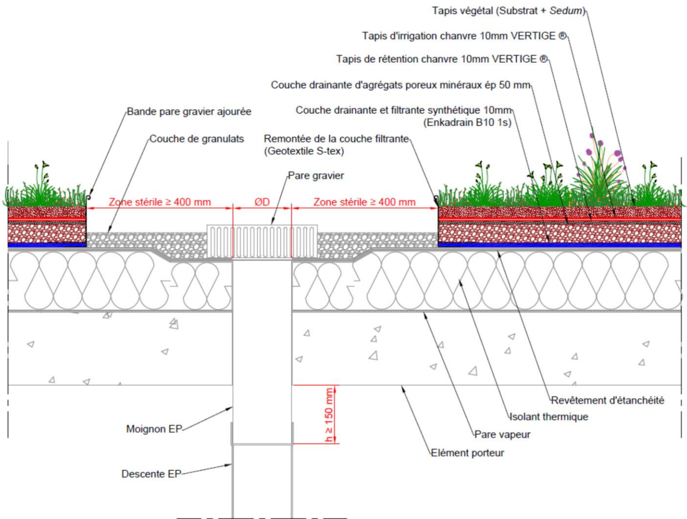
Figure 20 - Coupe sur descente d'eaux pluviales sur élément porteur en maçonnerie de pente comprise entre 0 et 2 % sans couche de substrat complémentaire (VERTIGE® EXTENSIF ORIGINAL)
