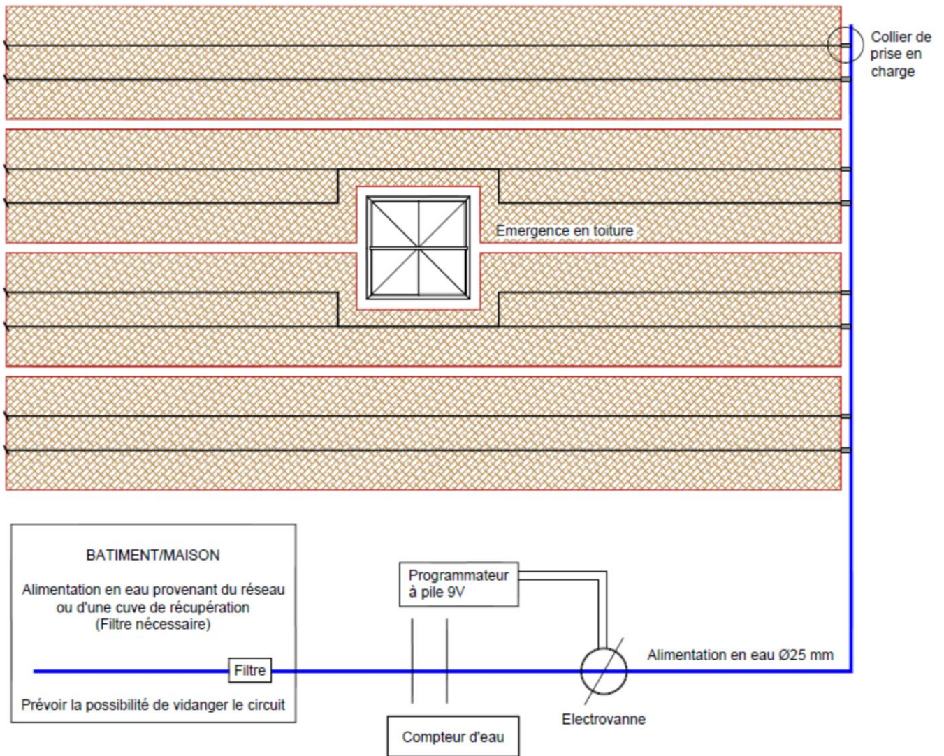
Figure 9 - Schéma de principe du système d'irrigation
