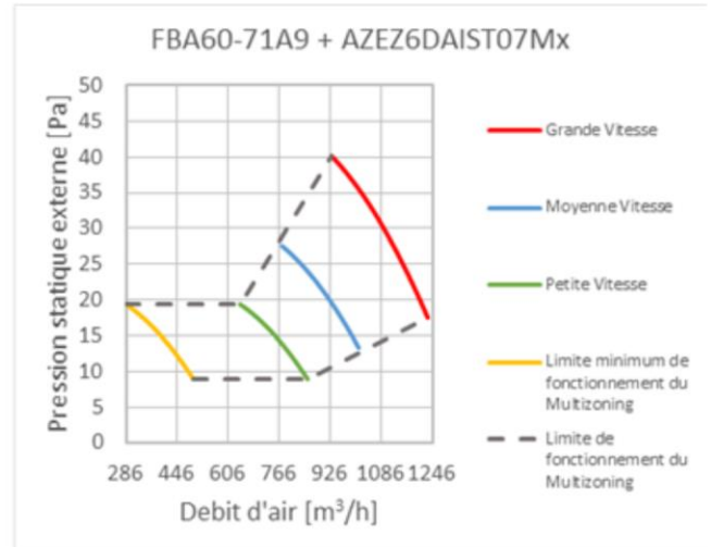
Figure 6 – Unités intérieures FBA60A9 et FBA71A9 Courbes débit/pression
