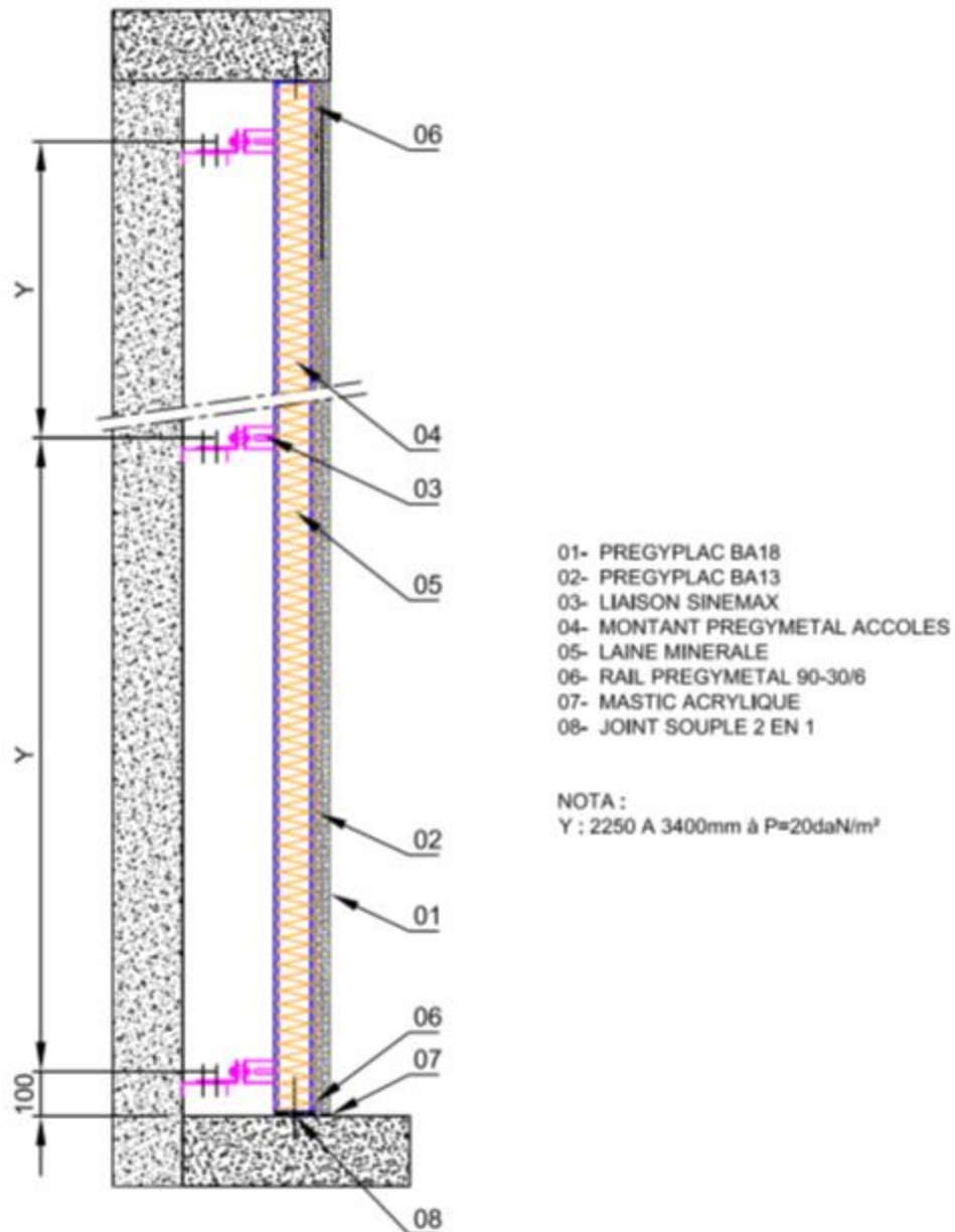
Figure 10 – Coupes de principe contre-cloison SINEMAX®
