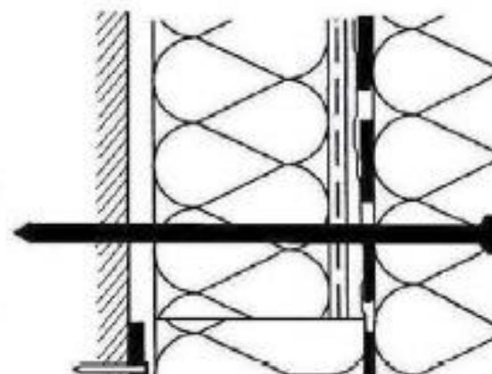
Figure 2d : nouveau profilé de départ après élimination de l'existant
