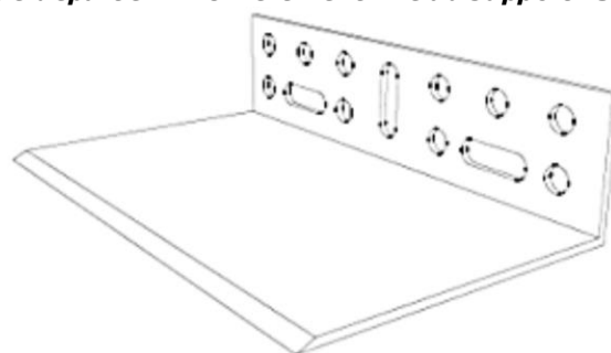
Figure 3a : Profilé de départ en PVC – élément fixé au support : Sto-Profil Départ PH - K
