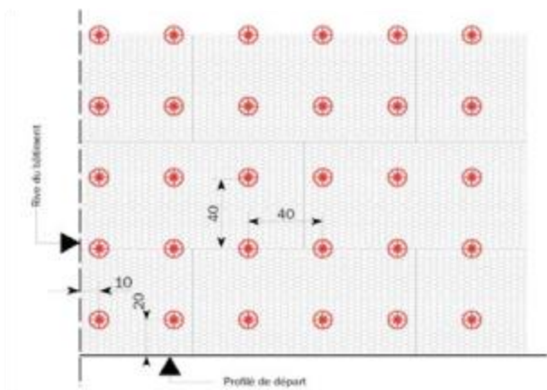
Figure 3a : Calepinage 40 cm x 40 cm
