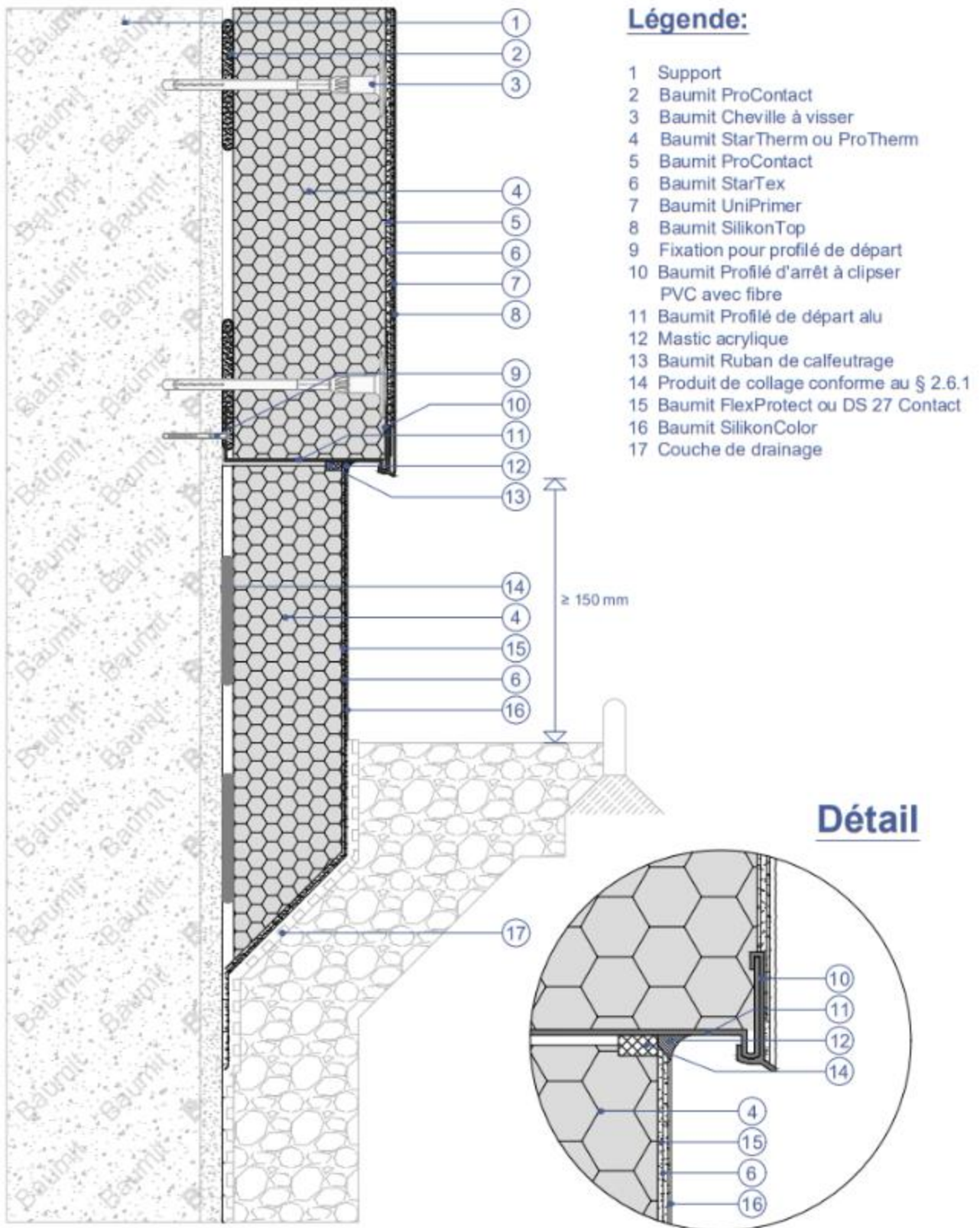
Figure 9a : Départ en partie semi-enterrée - décroché entre la partie semi-enterrée et la partie courante
