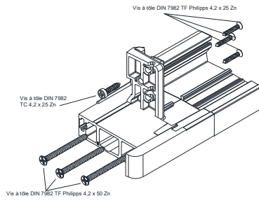
Montages DK40-RT entre dormants
