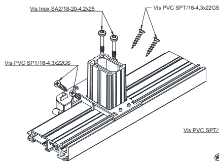
Montage dormants de base, rénovation et monobloc.
