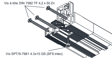
Montages DK20-RT entre dormants
