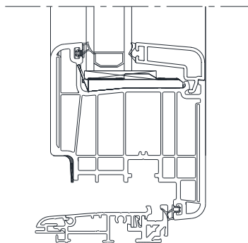
Ouvrant de 82, battée 2252.
