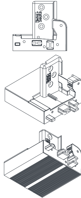
Patte DK40-EDI-5001 avec Mousse d'étanchéité
