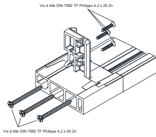
Montages des embases de tapée d'isolation
