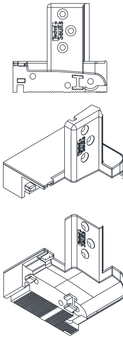
Patte DK20-SDI-5001 avec Mousse d'étanchéité
