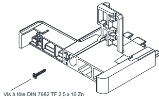
Montages des embases de tapée d'isolation
