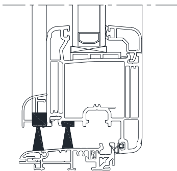
2 brosses en quinconce (diffusion restreinte )
