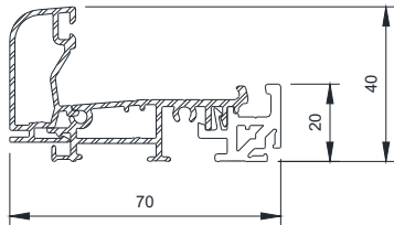
Seuil de 40 ATL40.
