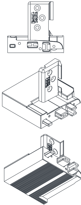
Patte DK20-EDI-5001 avec Mousse d'étanchéité
