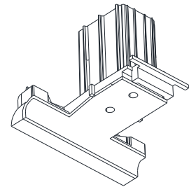
CM80 : pour Meneaux 3081-3082-5182, avec platine d'étanchéité.
