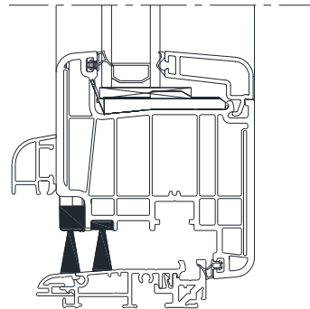
2 brosses en quinconce (diffusion restreinte )
