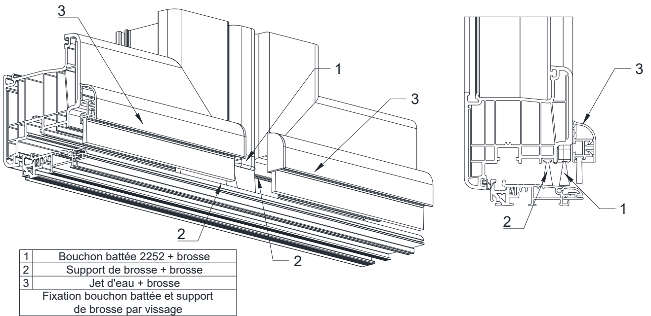
Ouvrant de 70, bouchon battée 2252
