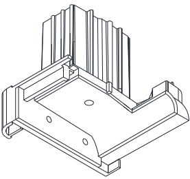
CB70 : pour dormant 5001-5014, avec platine d'étanchéité.
