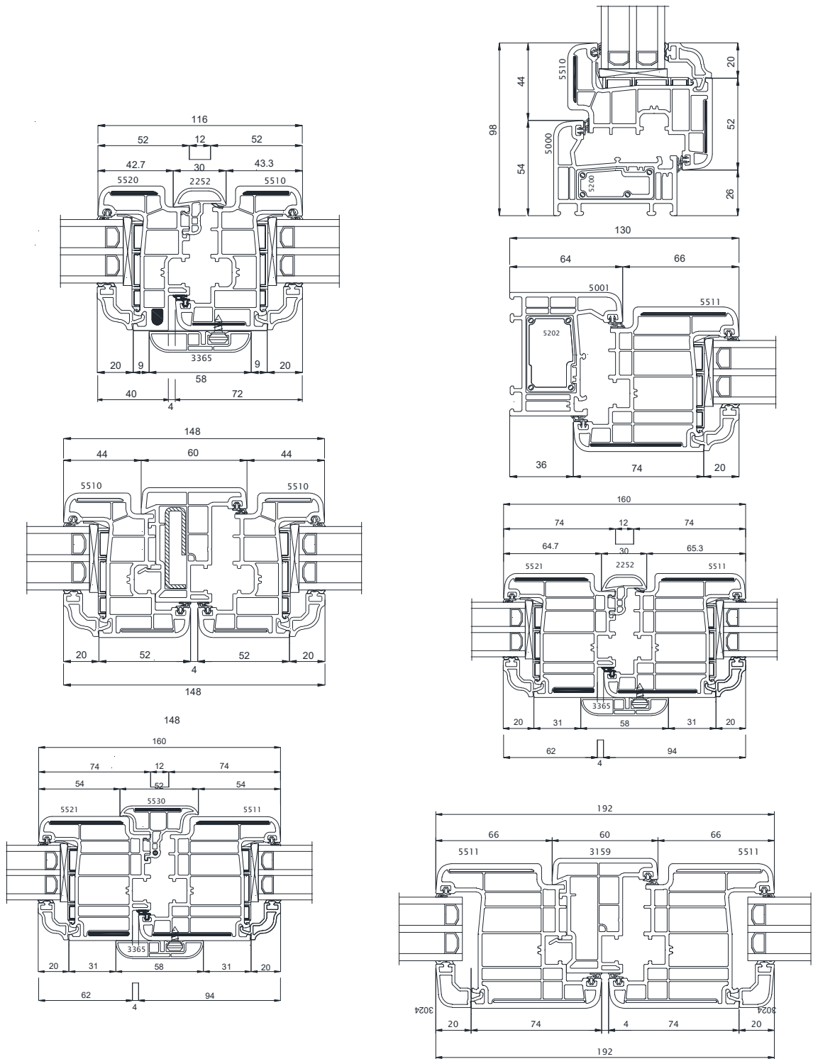
COUPES DE PRINCIPE ZENDOW#NEO
