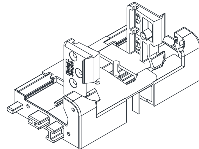
Patte DK40-EDI-5182 avec Mousse d'étanchéité
