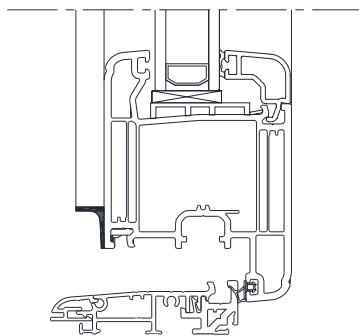
Ouvrant de 70, battée 2252.
