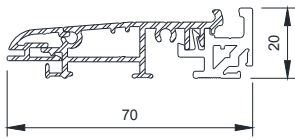
Seuil de 20 ATL20 .
