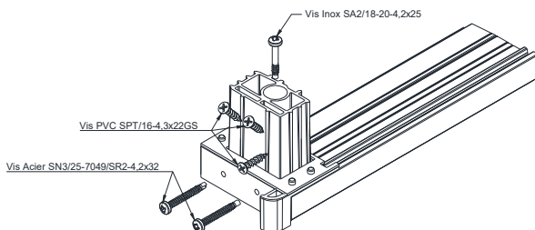
Montage dormants de base, rénovation et monobloc.
