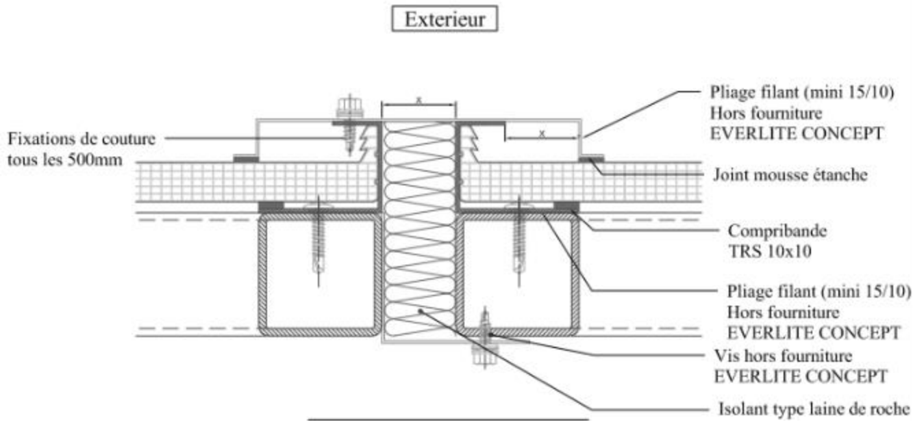
Figure 14 - Point particulier – Joint de dilatation sur panneaux entiers
