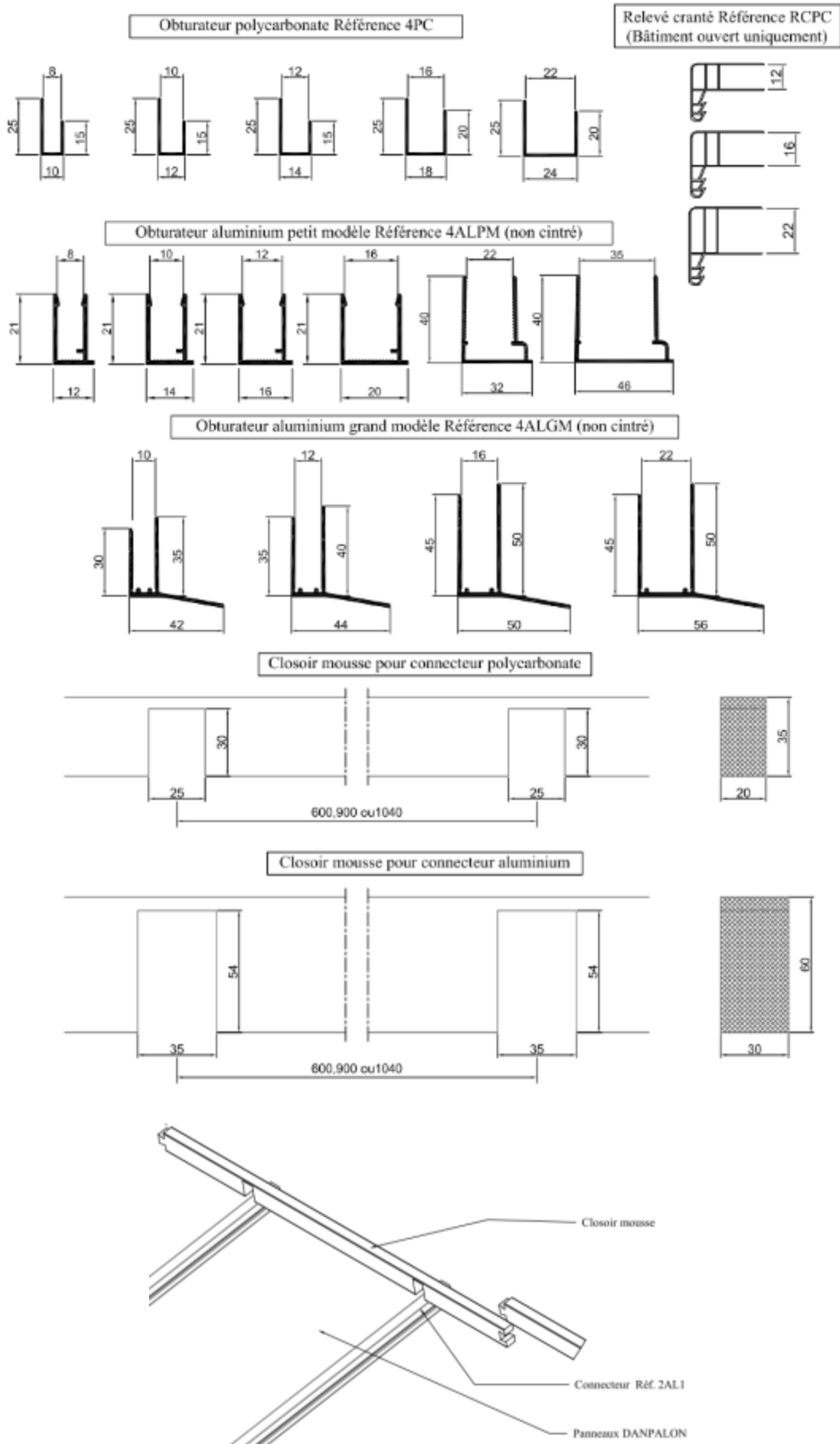
Figure 5 - Obturbateurs et cloisirs mousses
