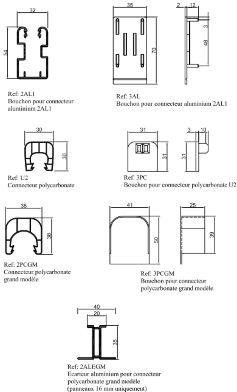
Figure 2 – Connecteurs et bouchons
