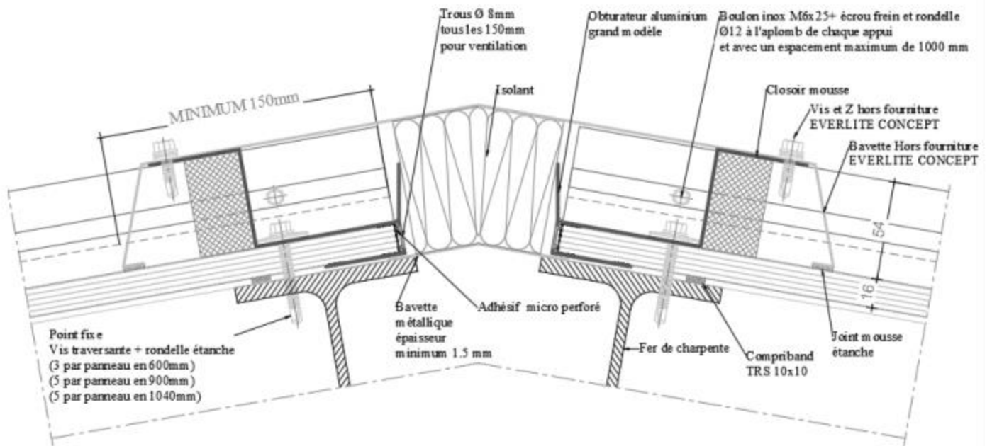
Figure 10 - Point particulier – Faîtage
