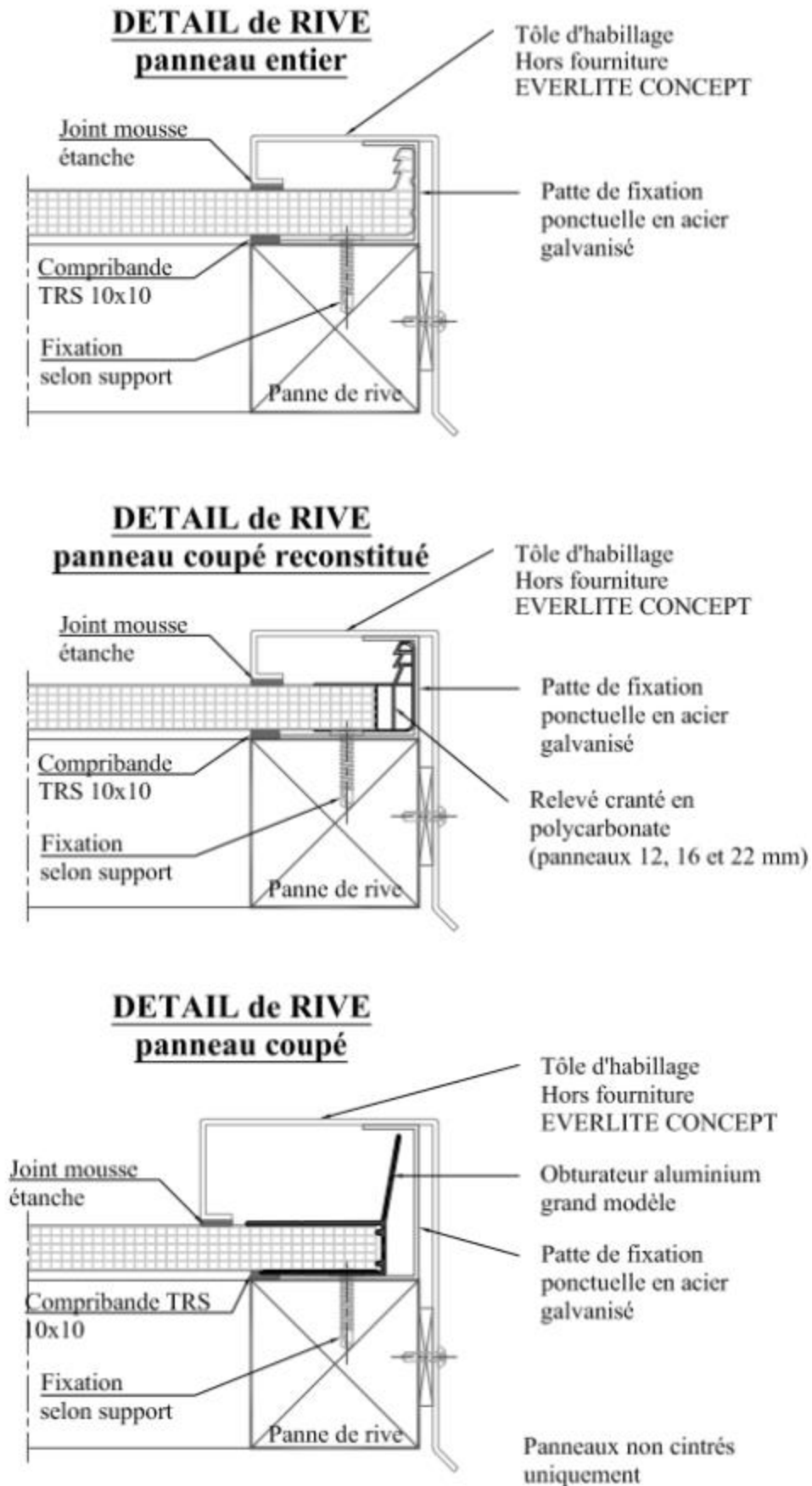
Figure 13 - Point particulier – Rives sur panneaux entiers, panneaux coupés reconstitués avec relevés crantés (12, 16 et 22 mm) et panneaux coupés (uniquement dans le cas de bâtiments ouverts)
