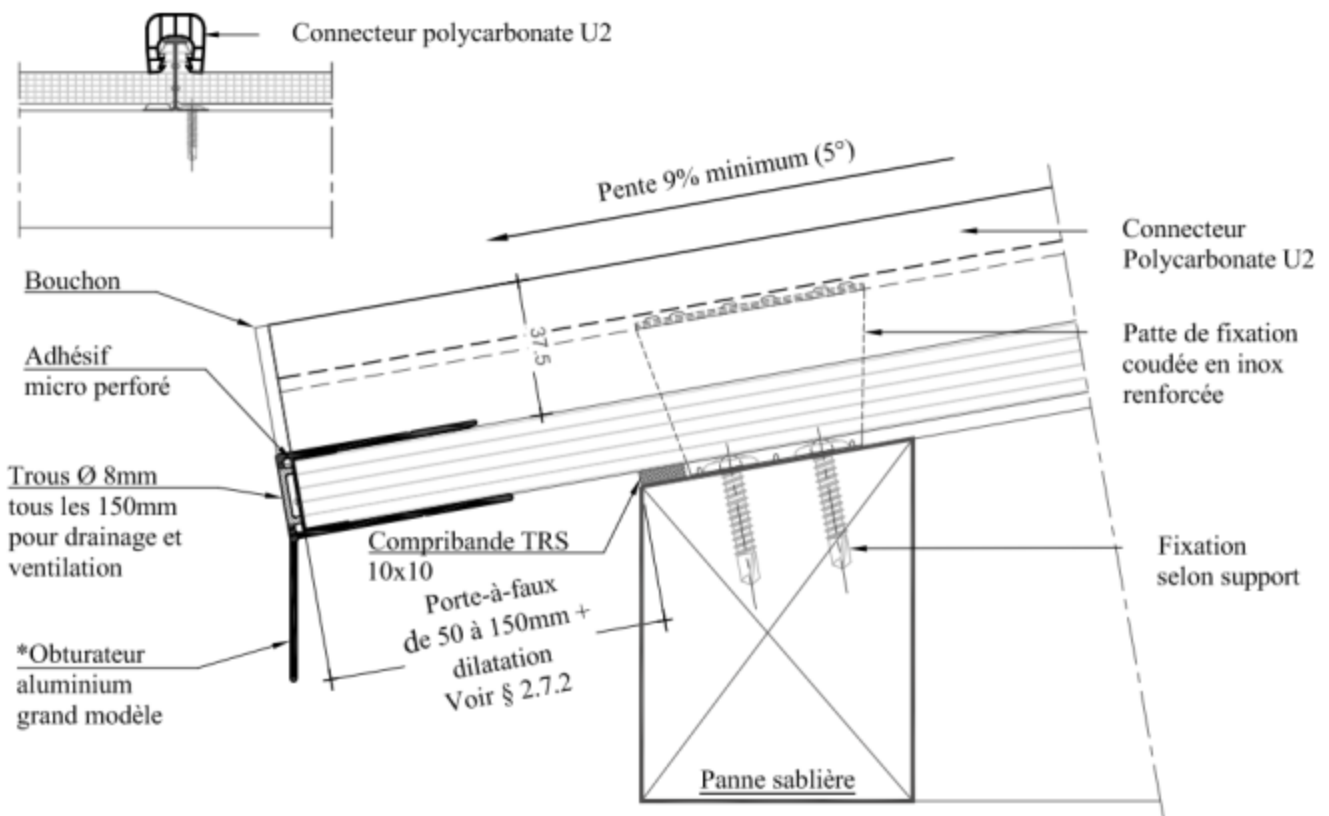
Figure 9.2 – Point particulier - Fixation sur costière ou sablière (point bas) connecteur polycarbonate
