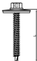
FASTOVIS TH 2C - Supraccoat 2C - Ø 6,5 ou DRILLNOX Bois TH 2C - Inox A4 - Ø 6,3 ou DRILLNOX Bois DF - Inox A4 - Ø 6,5 Support bois Longueur (L) selon l'épaisseur du panneau
