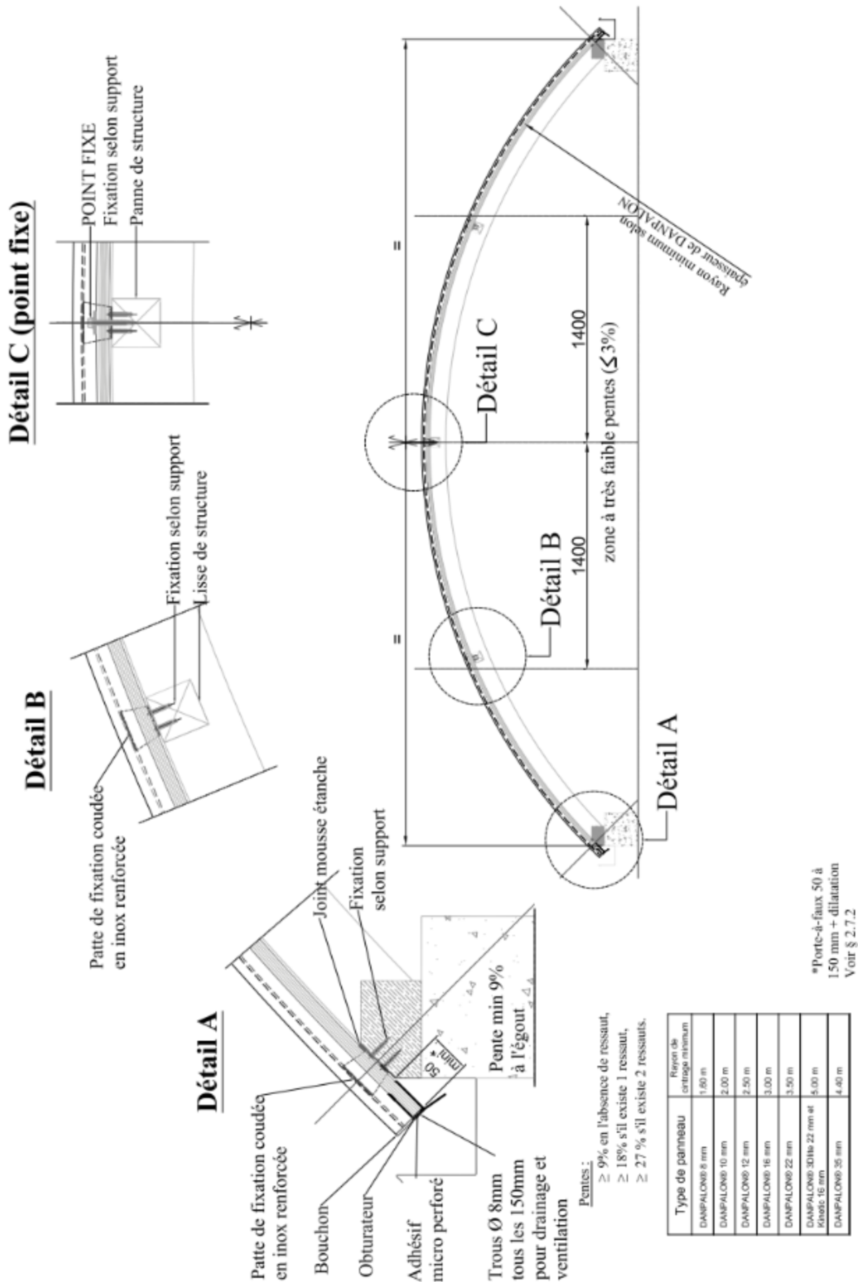
Figure 16 - Pose cintrée – Voûte - Coupe longitudinale et transversale sur connecteur polycarbonate Pente en bas de rampant : cf. § 2.7.3.1
