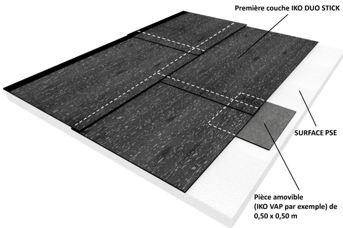
Figure 2 - Protection des recouvrements transversaux de 20 cm pour les membranes IKO DUO STICK, IKO DUO FUSION L4 JA F/F et L4 JA F/MAT, ainsi que L4 SPF
