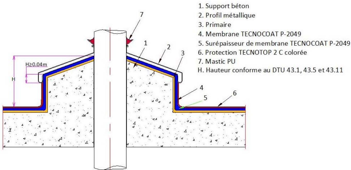
Figure 11 - Exemple de traversée d'une canalisation avec un dé en béton
