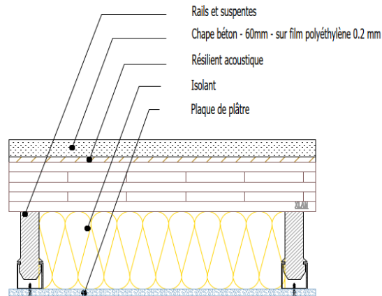
Figure 9 - Schéma de complexe en plancher XLAM
