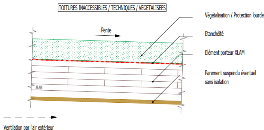
TOITURES INACCESSIBLES / TECHNIQUES / VEGETALISEES
