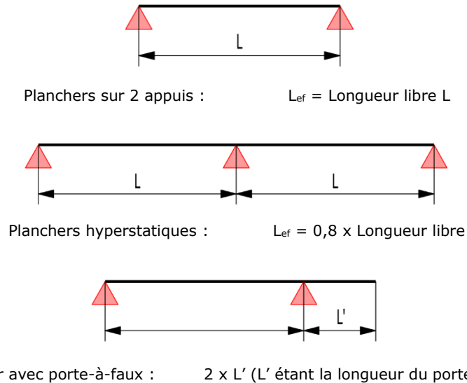
Figure 3 – Longueurs efficaces pour calcul du I_{eff}
