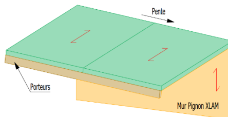
POSE TYPE PANNE
