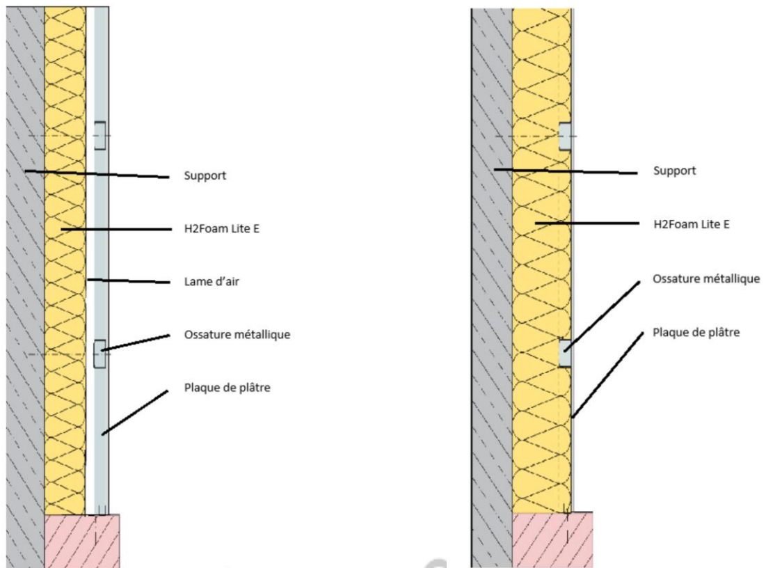
Figure 5 : Projection au niveau des rails avec lame d'air
