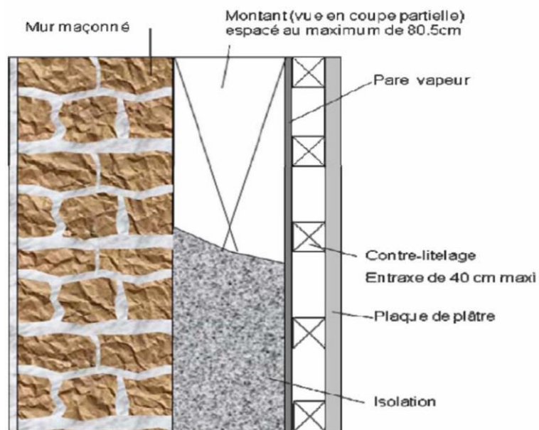
Figure 2 : Mur maçonneré – isolation intérieure derrière un pare-vapeur
