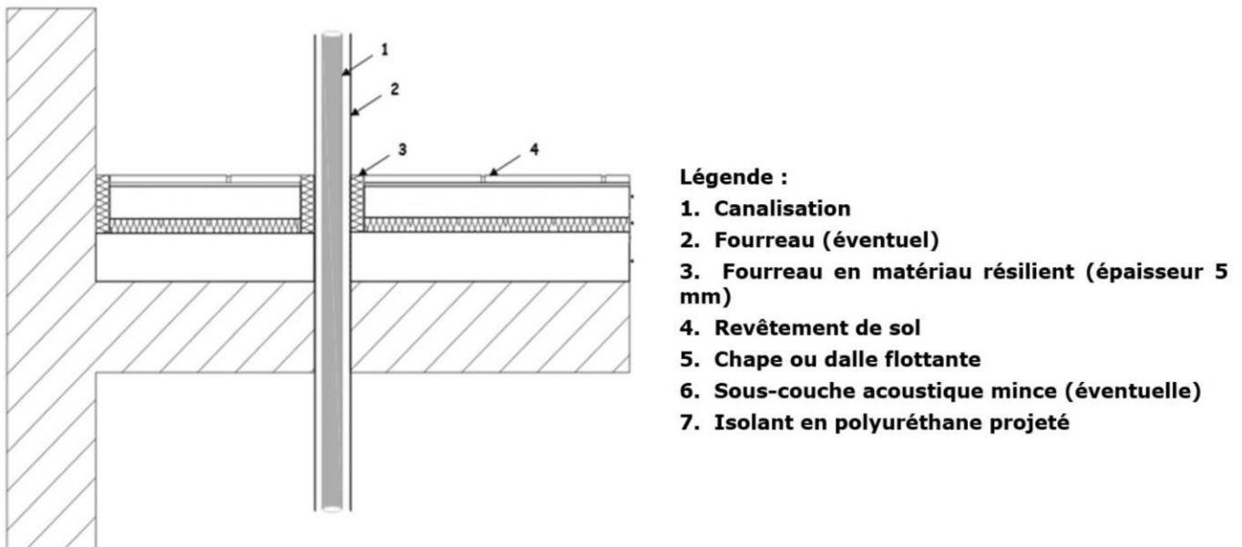
Figure 6 : Traitement d'une canalisation verticale traversant le support
