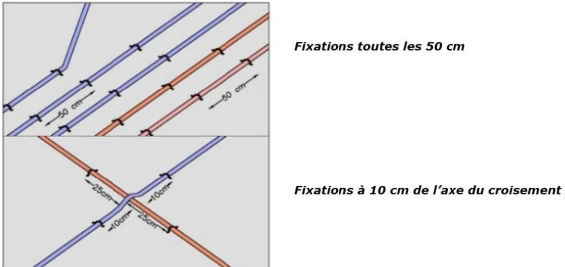
Figure 5 : Traitement des canalisations
