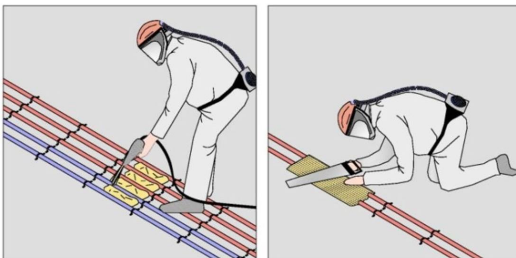
Figure 8 : Enrobage des gaines et arasement de l'excédent
