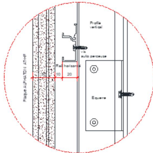
Coupe horizontale - Clip haut
