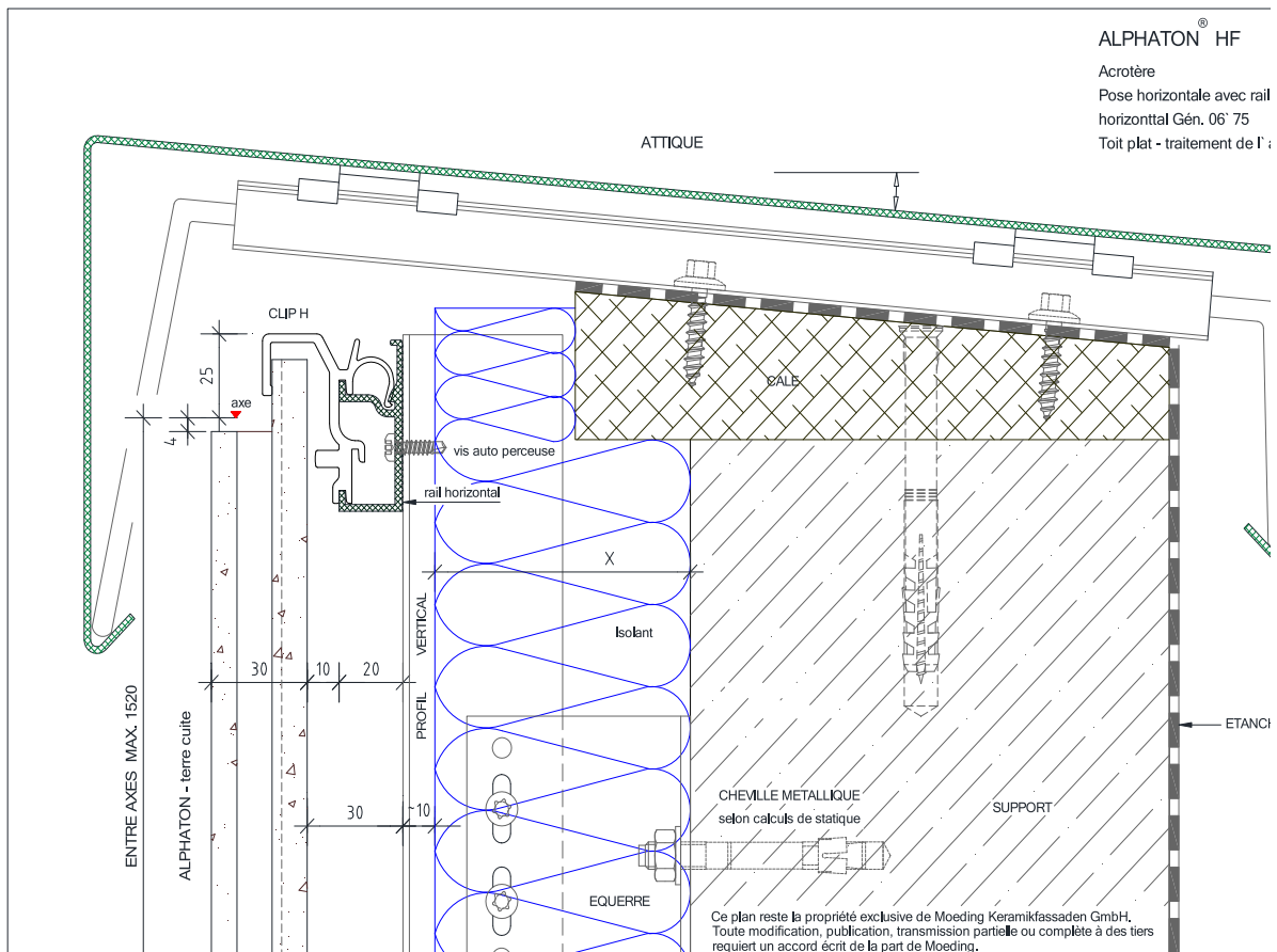
Figure 14 - Acrotère
