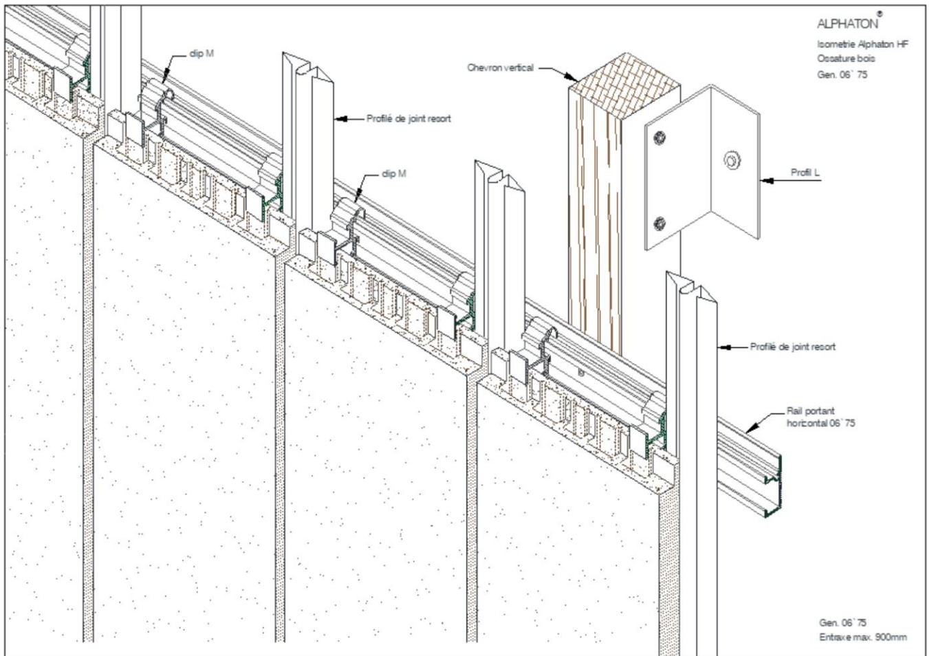
Figure 31 - Vue isométrique
