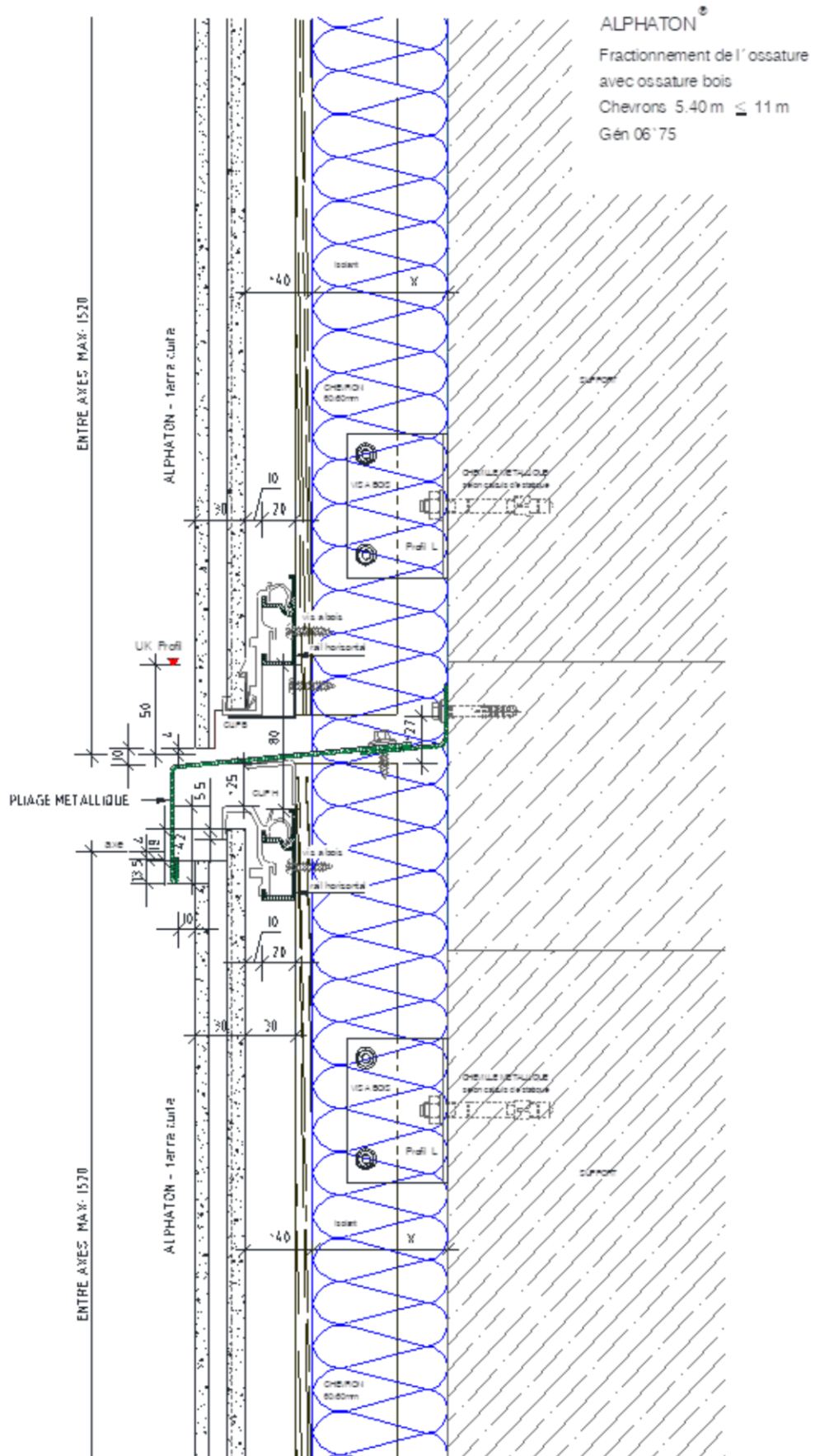
Figure 37 - Fractionnement de l'ossature - Chevrons 5,40m \leq 11m
