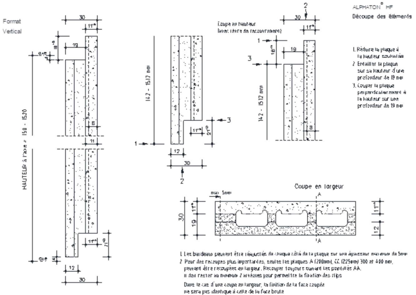
Figure 7 - Découpe des éléments terre cuite Alphonat® HF
