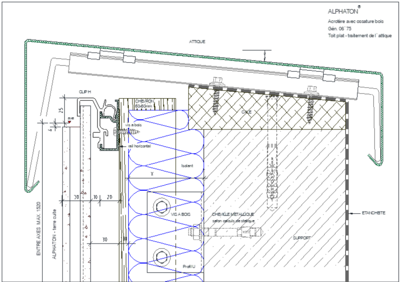
Figure 34 - Acrotère
