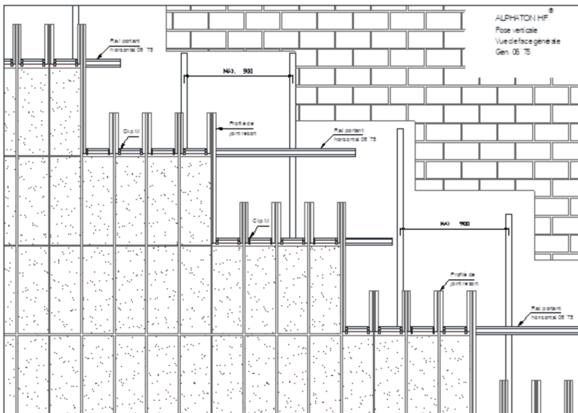
Figure 9 - Vue de face - pose avec rail porteur horizontal 06'75
