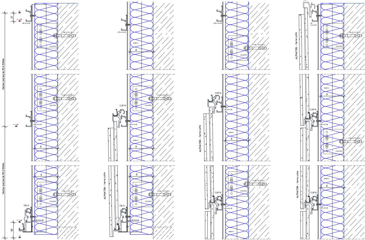
Figure 24 - Montage des bardeaux – méthode 1
