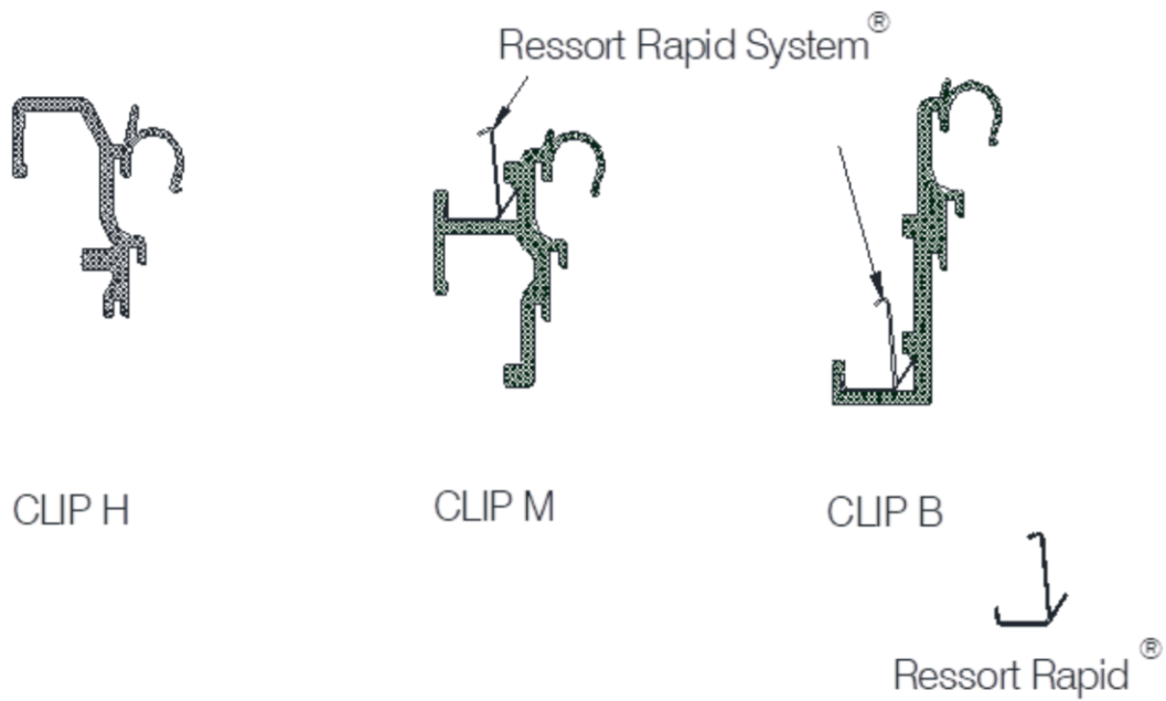
Figure 5 - Clips utilisés - Ossature métallique avec rail portant horizontal
