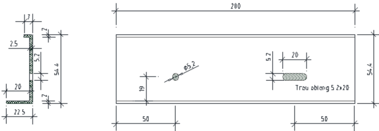
Figure 6bis - Pièce d'aboutage des rails horizontaux 06'75
