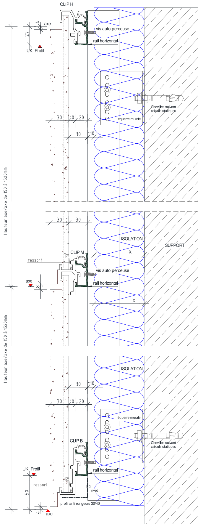
Figure 12 – Coupe verticale avec rail Gén 06'75 ouvert
