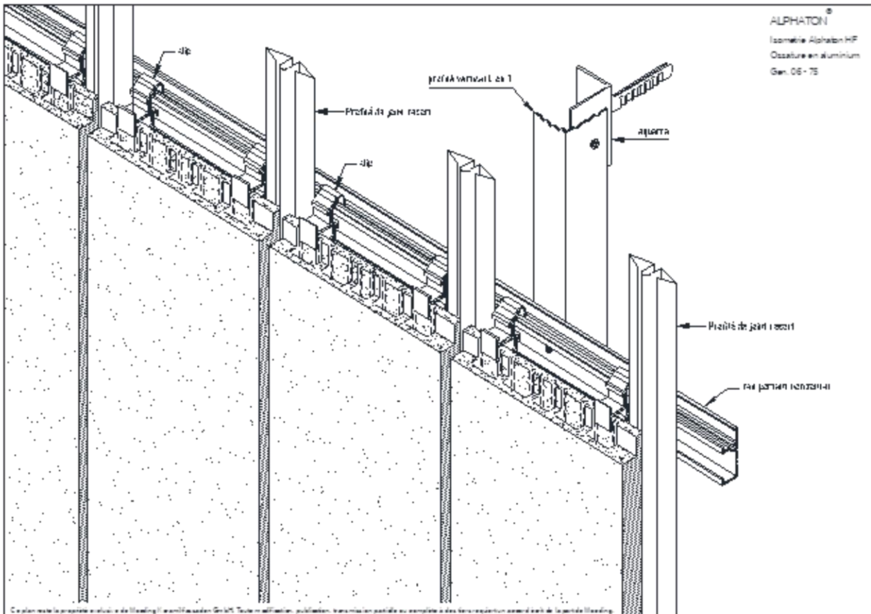
Figure 8 - Schéma de principe ossature métallique - Vue isométrique - pose avec rail porteur horizontal 06'75
