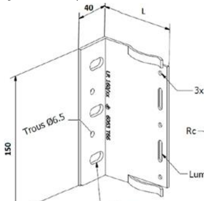
Figure B3 – Pattes-équerres ISOLALU+ LR160x200x50mm
