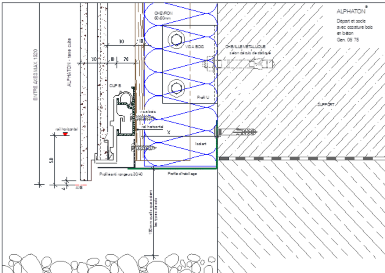
Figure 33 - Départ de façade et socle
