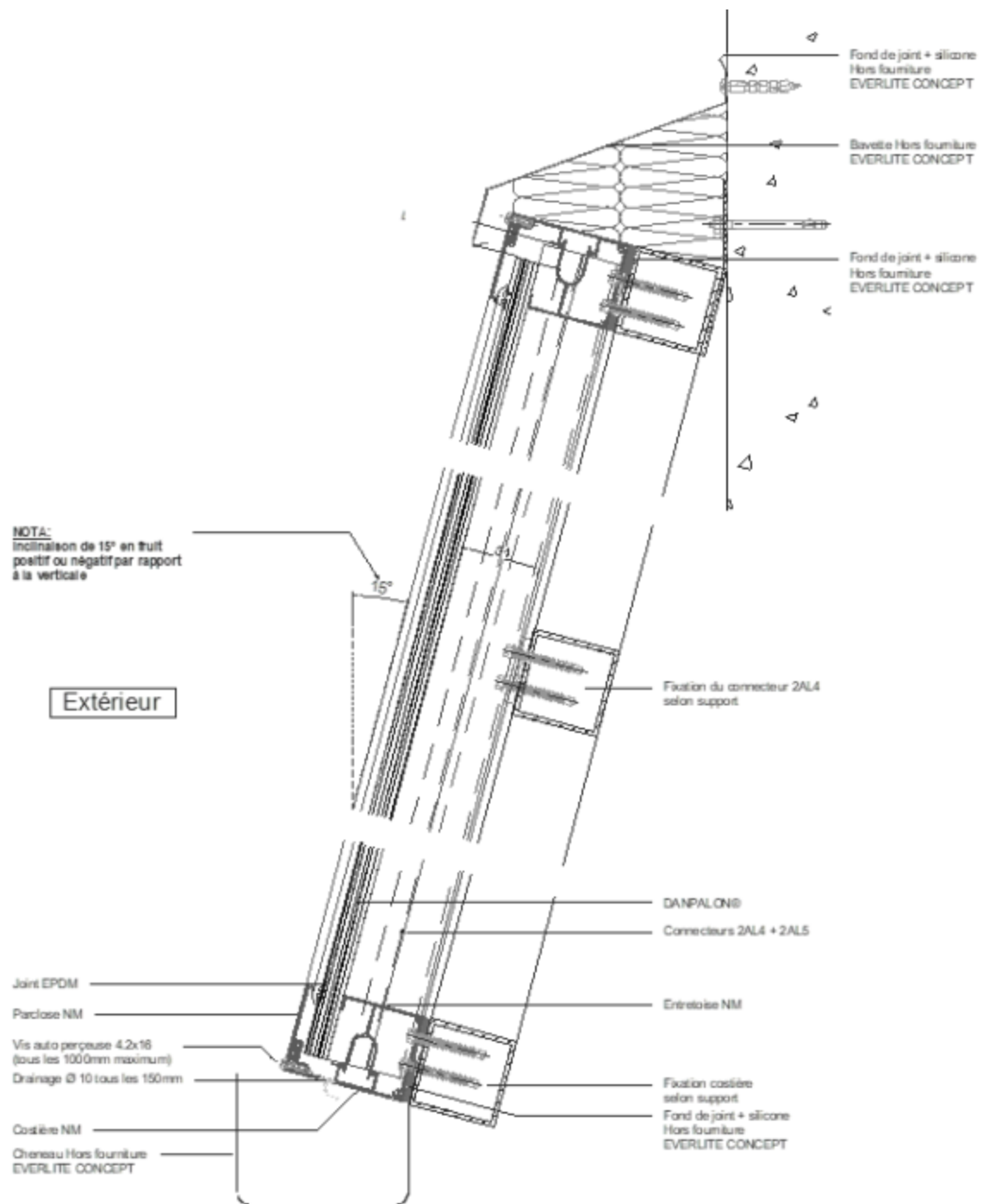
Figure 13.3 - Coupe verticale sur costière NM inclinée (SHED)
