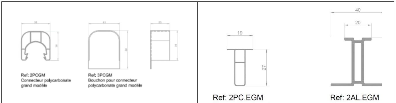
Figure 2.1 - Connecteurs et bouchons polycarbonate
