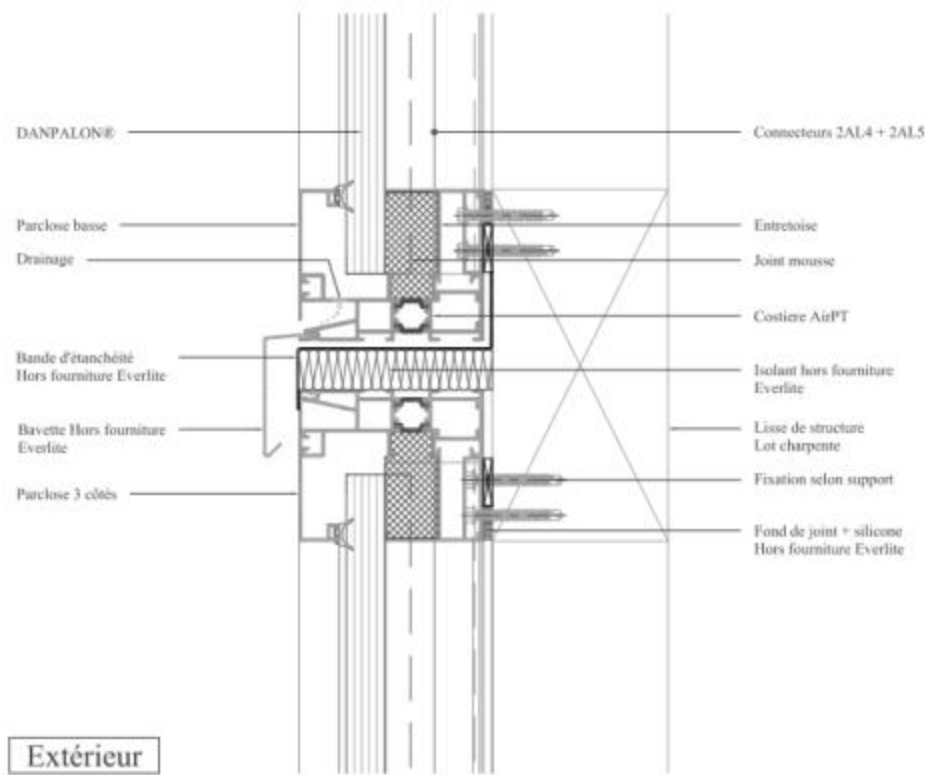
Figure 17.2 - Exemple d'aboutage de panneaux DANPALON® en pose inversée sur costière AirPT
