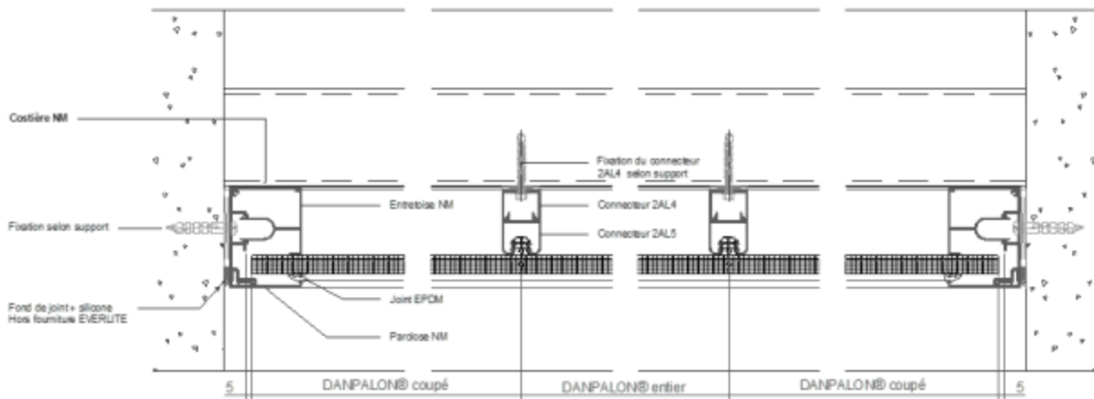
Figure 14.2 – Coupe horizontale sur costière NM (pose en tableau)
