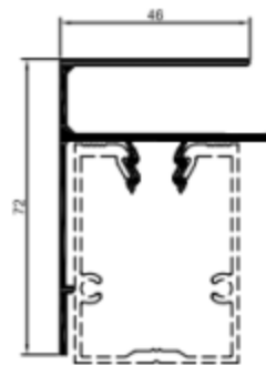
Profil de rive panneau coupé épaisseurs 12 et 16 mm
