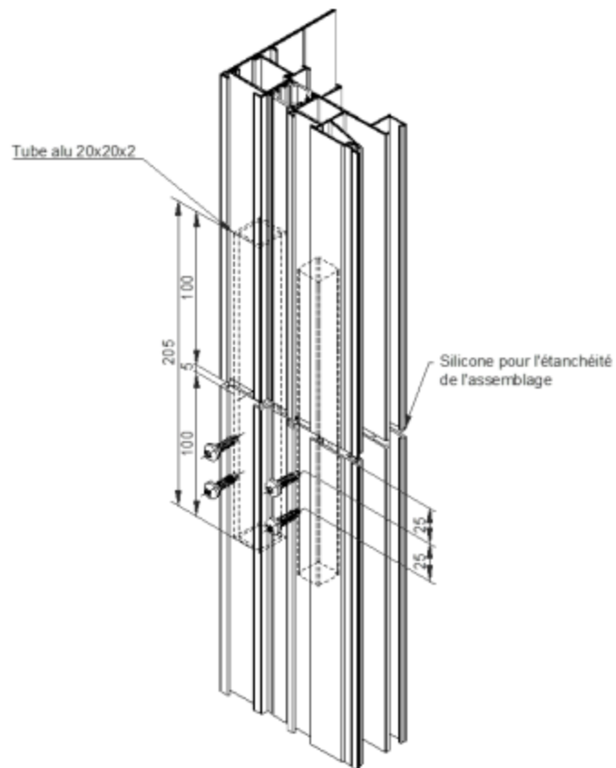
Figure 5.3 – Profils aluminium périphériques – Exemple d'éclissage
