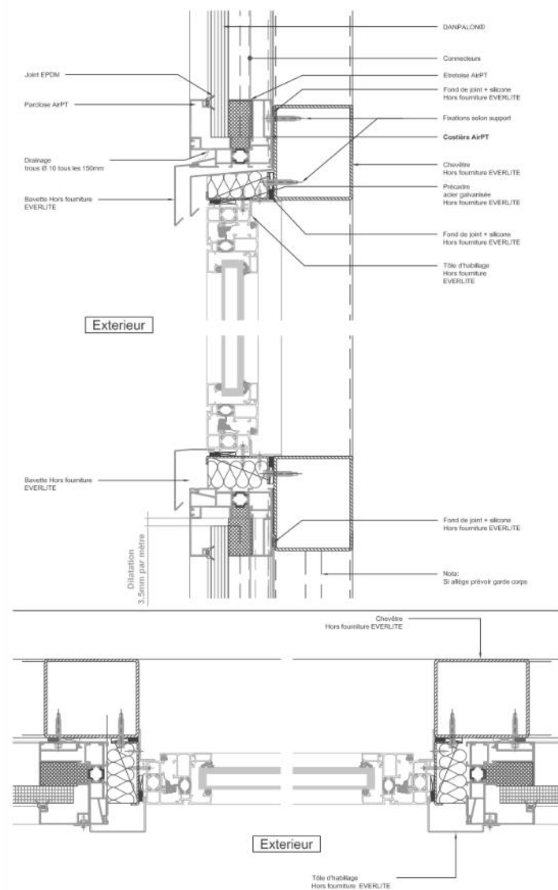
Figure 19 - Encadrement de baie
