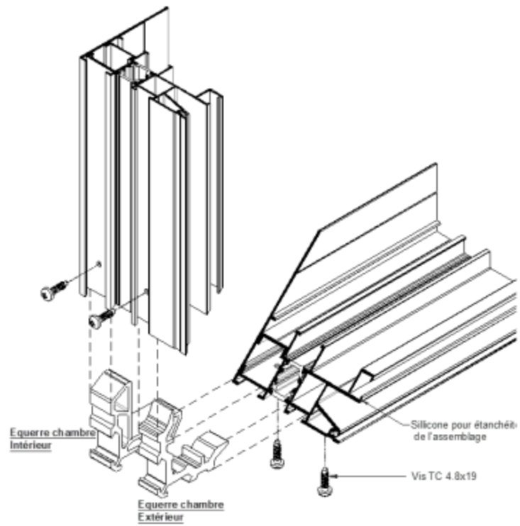
Figure 5.2 - Profils aluminium périphériques – Exemple d'aboutage d'angle
