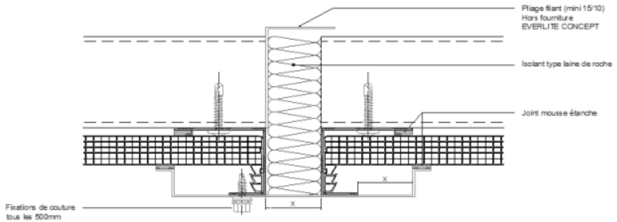
Figure 20.1 – Joint de dilatation avec pattes et pliages
