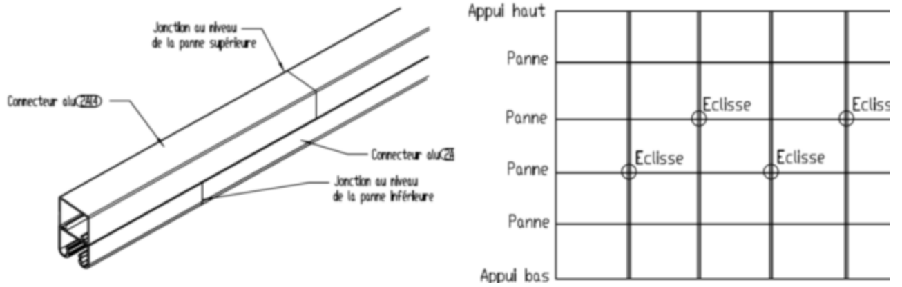
Principe sur connecteur 2AL4/2AL5
