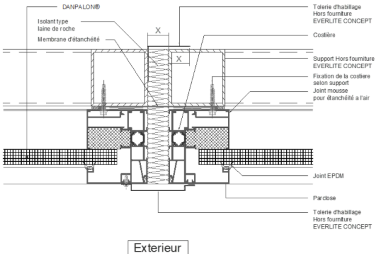
Figure 20.2 – Joint de dilatation avec costière
