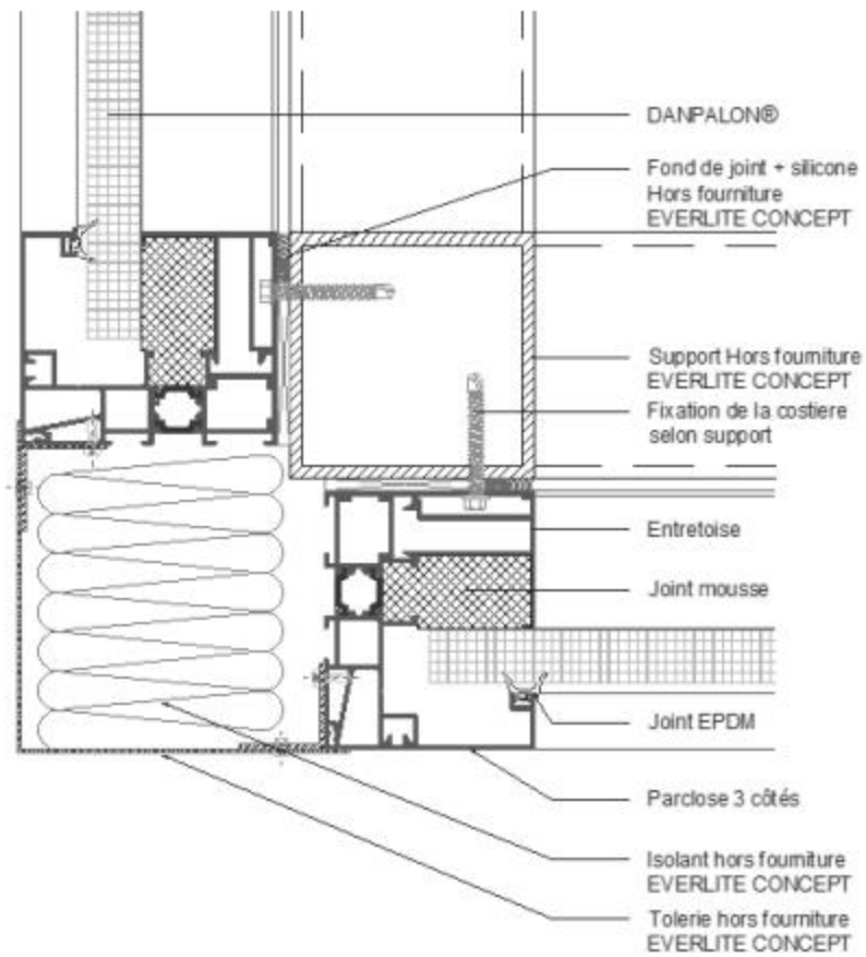
Figure 18.2 - Solution d'angle avec costière AirPT
