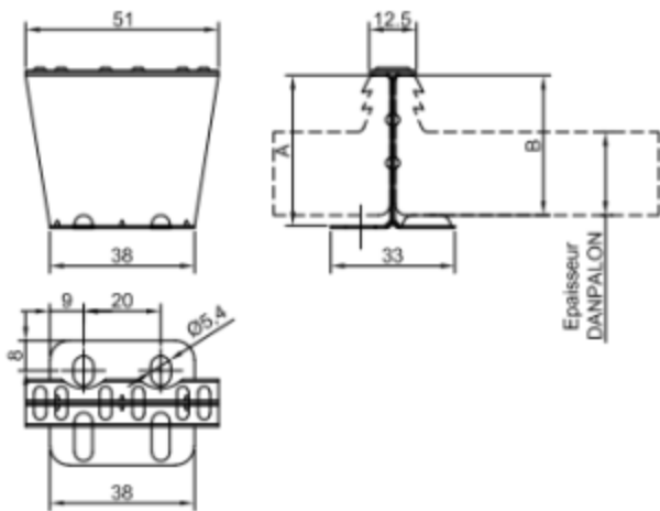
Pattes de fixations coudées - Type 51 DPFE
