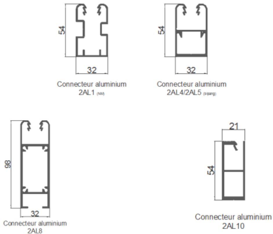
Figure 2.2 - Connecteurs aluminium
