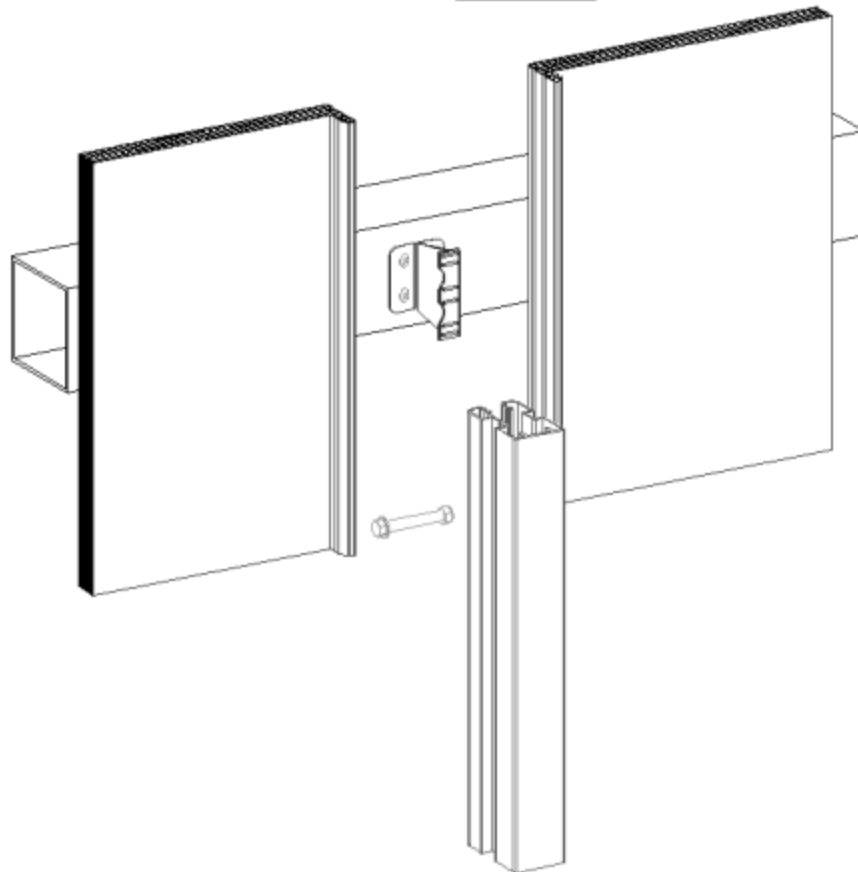
Figure 7 - Principe de mise en œuvre
