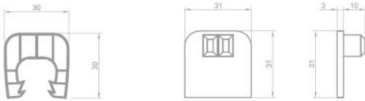
Ref: U2 Connecteur polycarbonate
