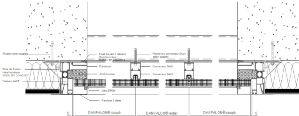
Figure 16.1 – Coupe horizontale sur costière AirPT (pose en applique)
