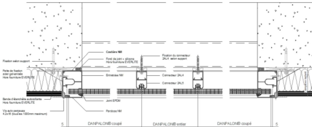
Figure 14.1 – Coupe horizontale sur costière NM (pose en applique)
