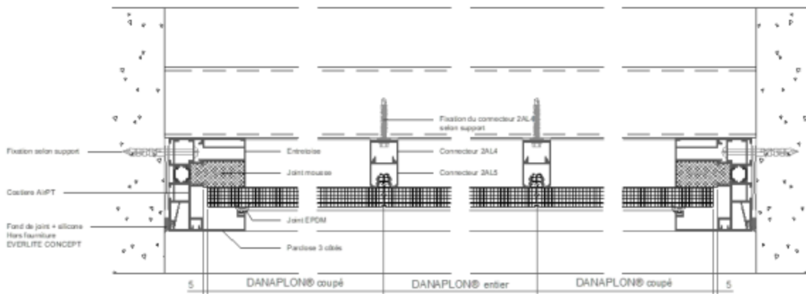
Figure 16.2 – Coupe horizontale sur costière AirPT (pose en tableau)
