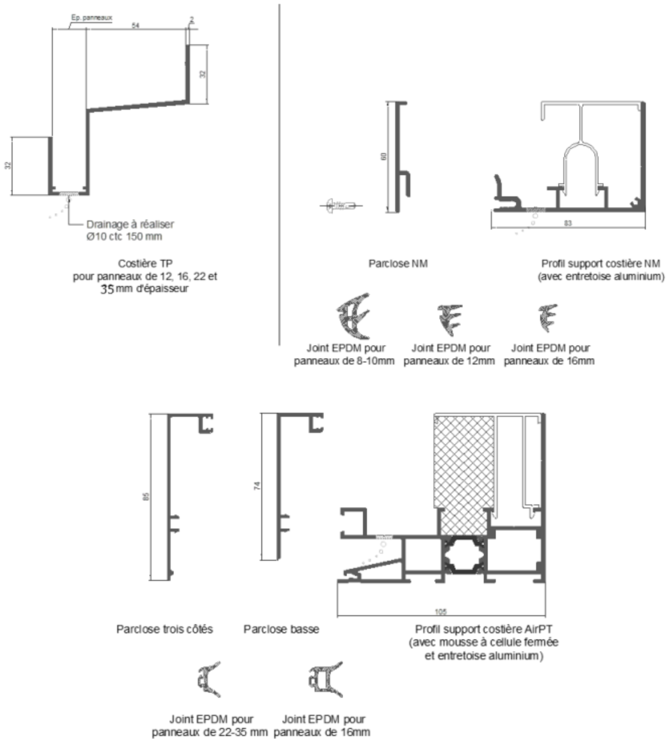
Figure 5.1 – Profils aluminium périphériques
