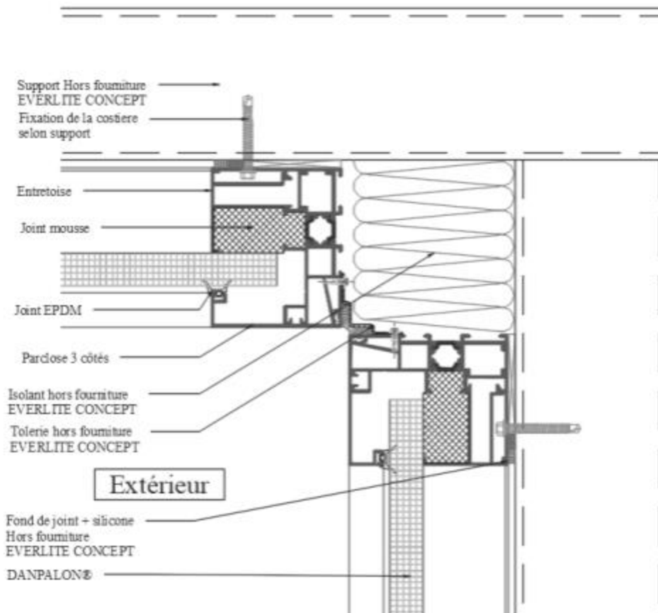
Figure 18.3 - Solution d'angle avec costière AirPT (angle rentrant)
