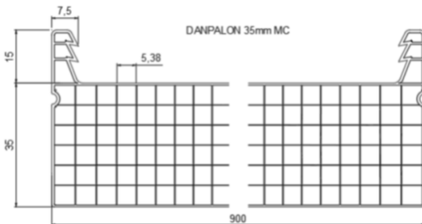
Figure 1.2 - Détails des panneaux DANPALON®16, 22 et 35
