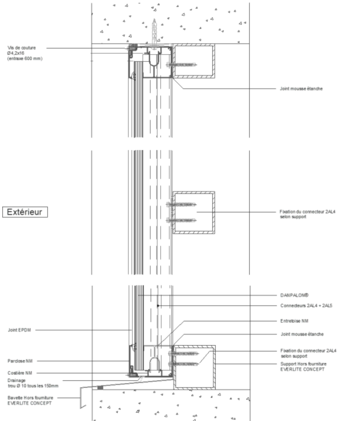
Figure 13.2 - Coupe verticale sur costière NM (pose en tableau)
