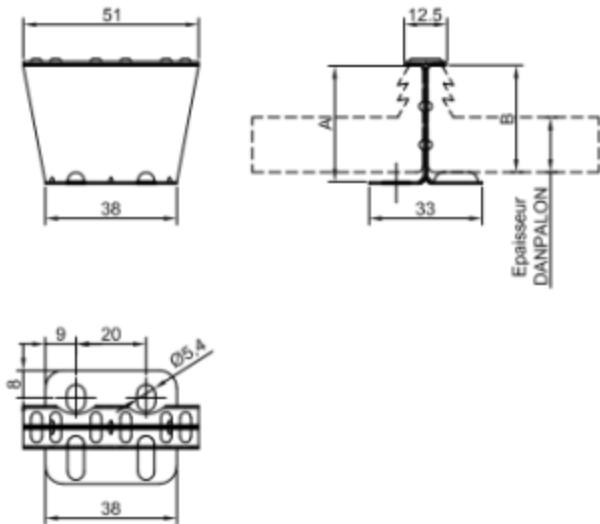
Pattes de fixations coudées - Type 51 CPI
