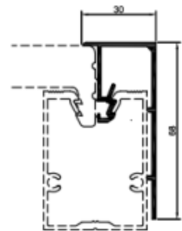
Profil de rive panneau entier épaisseurs 12 et 16 mm
