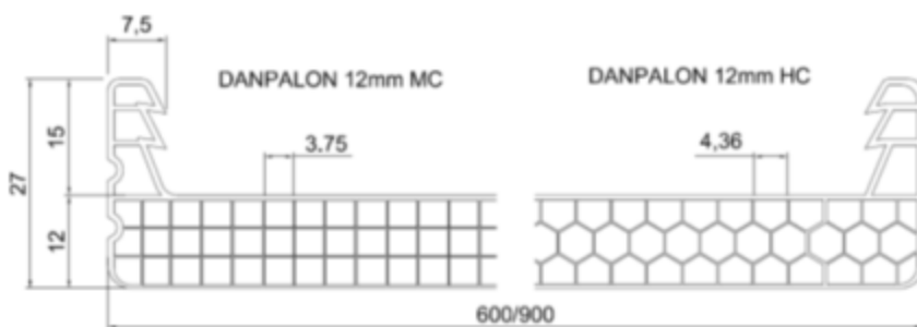
Figure 1.1 – Détail des panneaux DANPALON® 8, 10 et 12mm
