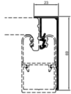
Profil de rive panneau entier épaisseur 16 mm
