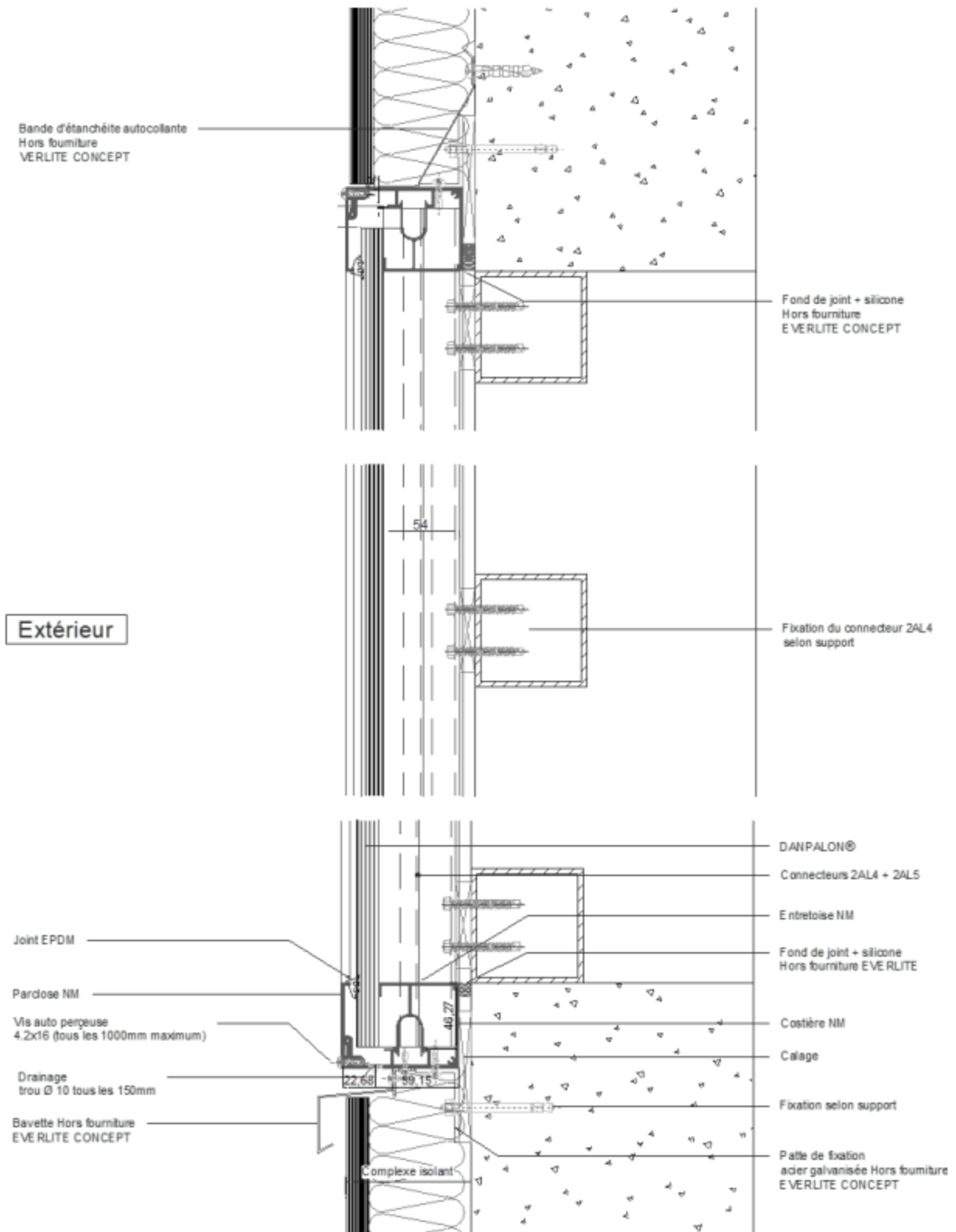
Figure 13.1 - Coupe verticale sur costière NM (pose en applique)
