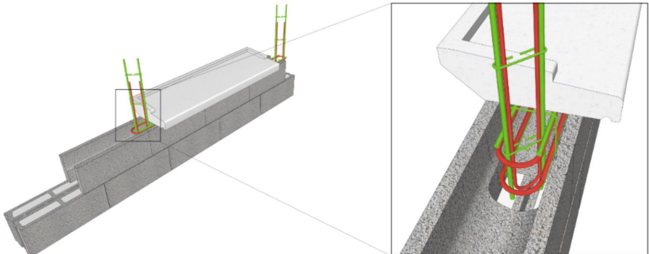
Figure 8 - Réalisation des tableaux de baies
