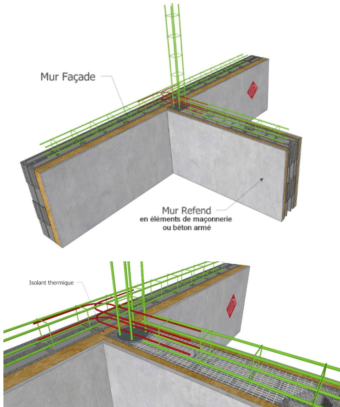
Figure 7 - Jonction par juxtaposition d'un mur de refend à un mur de façade toutes zones sismiques
