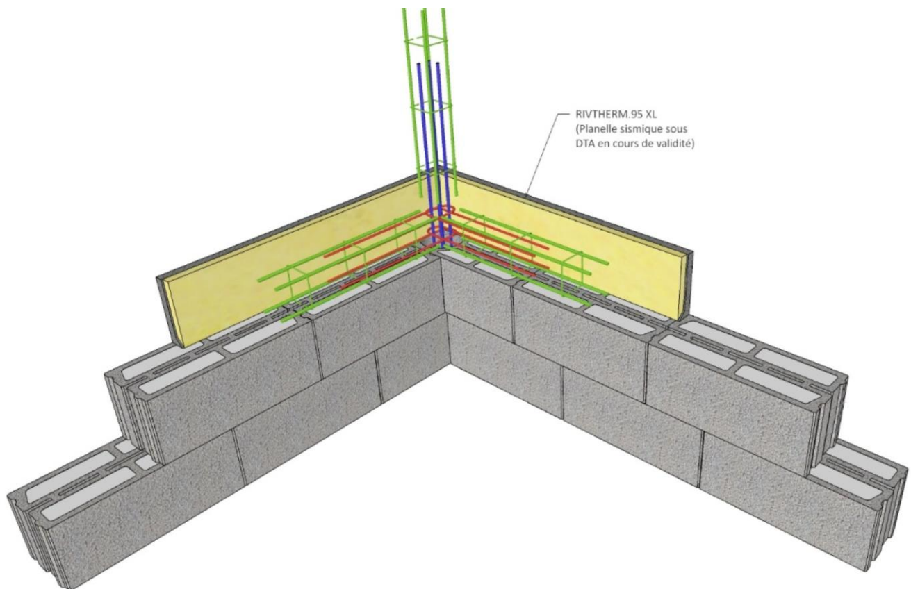
Figure 11 - Schéma de mise en œuvre de la planelle
