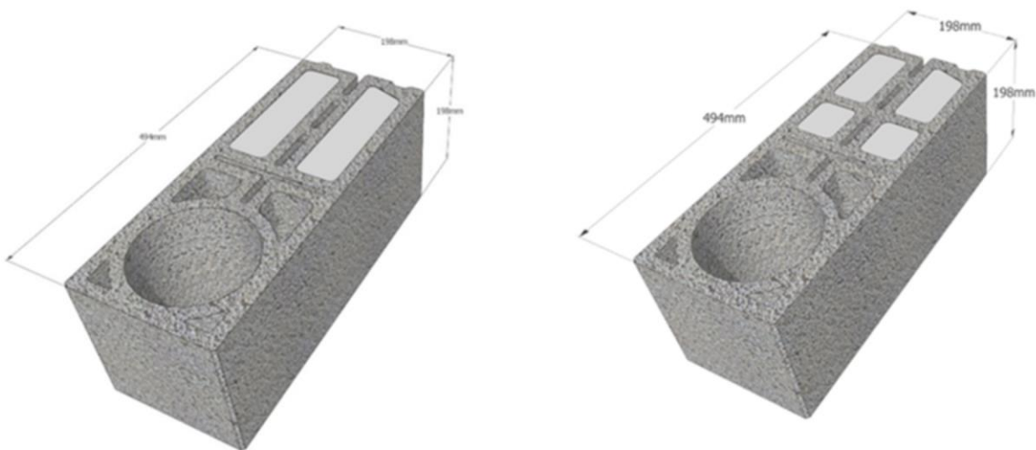
Figure 4 – FABTHERM AIR 1.1 angle de coupe
