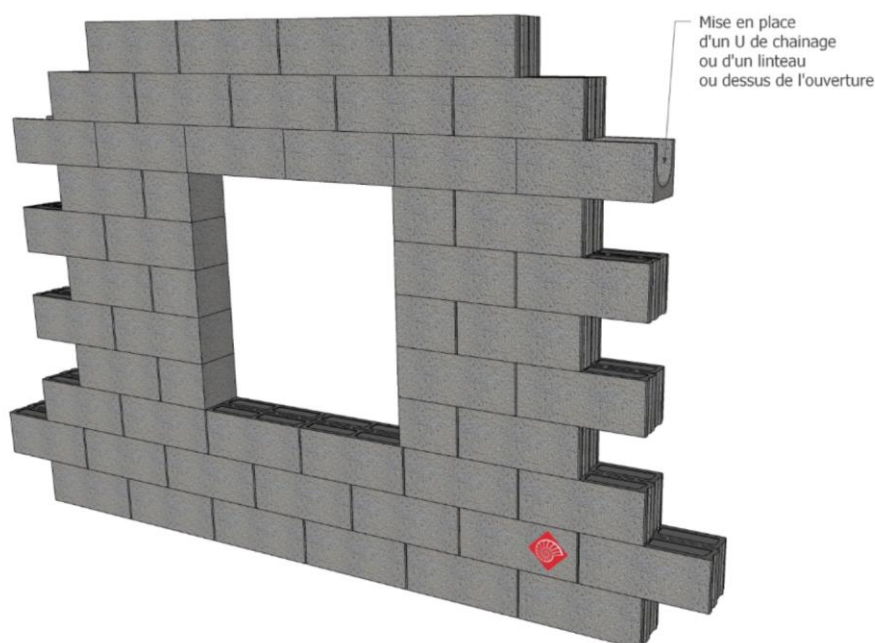
Figure 10 – Réalisation des appuis de fenêtre
