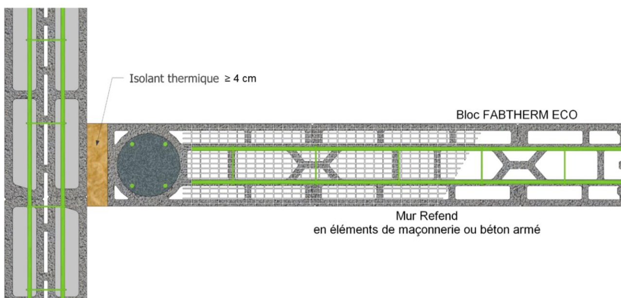
Figure 6 - Jonction par juxtaposition d'un mur de refend à un mur de façade non contreventant en zones sismiques 1 et 2
