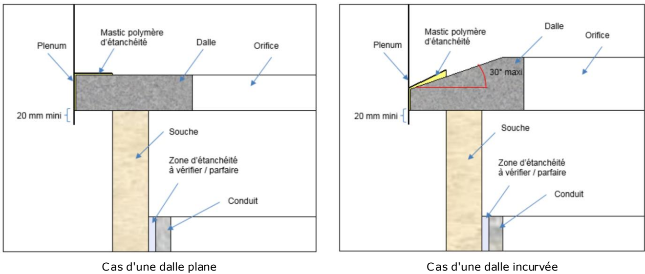
Figure 36 - Coupe verticale d'un plenum de recouvrement avec goutte d'eau sur dalle conservée
