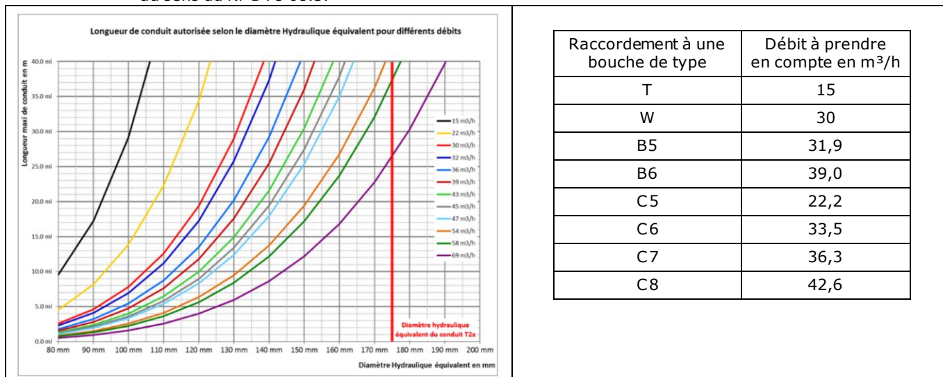
Figure 33 – Abaque de dimensionnement des conduits horizontaux T2a – Longueur maximale
