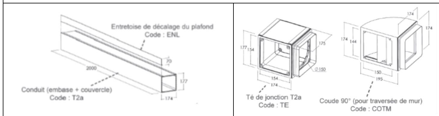
Figure 25 – Conduits horizontaux T2a – Caractéristiques techniques détaillées et dimensions
