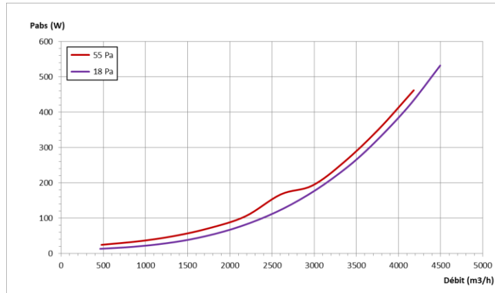
Figure 51 – MATRYS 4000U – courbes caractéristiques (vitesse de rotation maximale : 1500 tr/min)
