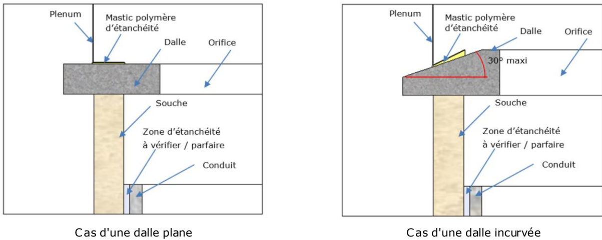
Figure 36 - Coupe verticale d'un plenum de recouvrement avec goutte d'eau sur dalle conservée
