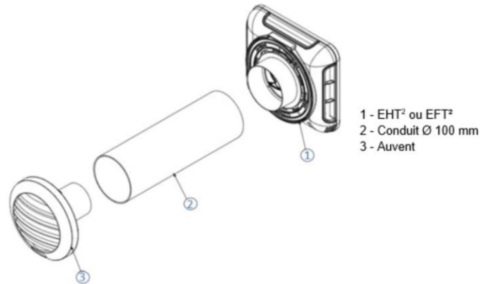
Figure 39 – Mise en œuvre entrée d'air EHT 2 et EFT 2 sans mousse Ø 100 mm L 300 mm
