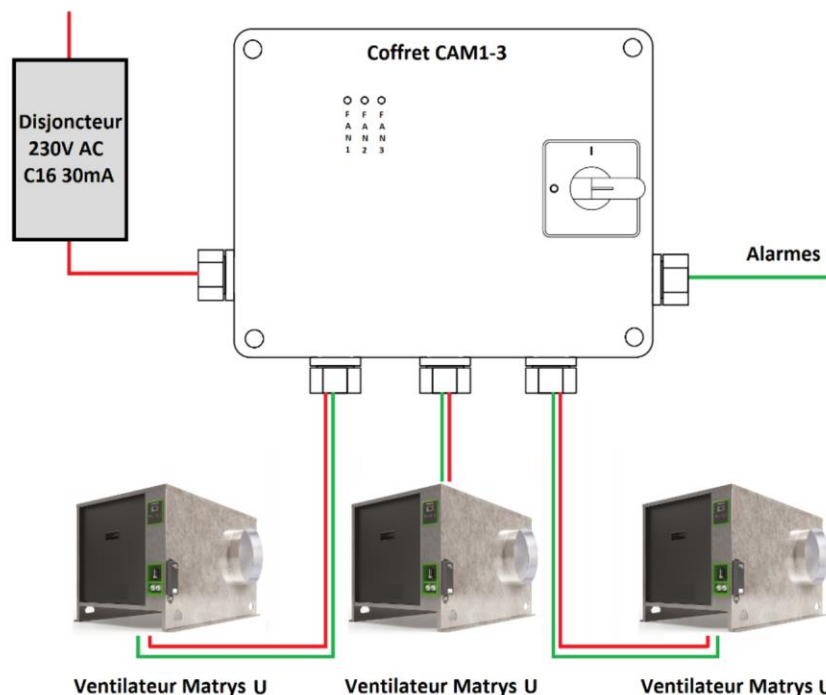
Figure 24 – Coffret d'asservissement CAM 1-3 – Visuel et schéma de principe du câblage
