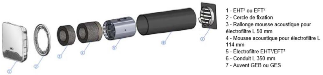
Figure 44 – Mise en œuvre entrée d'air EHT 2 et EFT 2 avec électrofiltre en conduit Ø 125 mm L 350 mm
