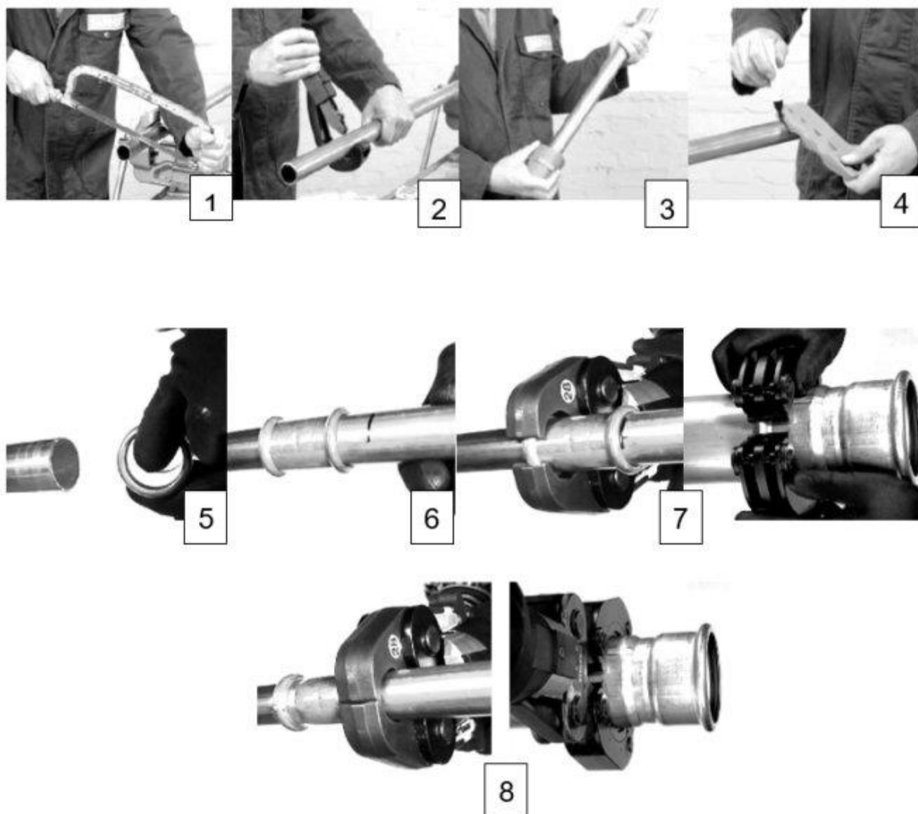
Figure 4 - Réalisation de l'assemblage
