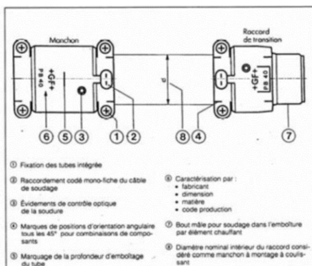
Figure 6 - Raccords électrosoudables
