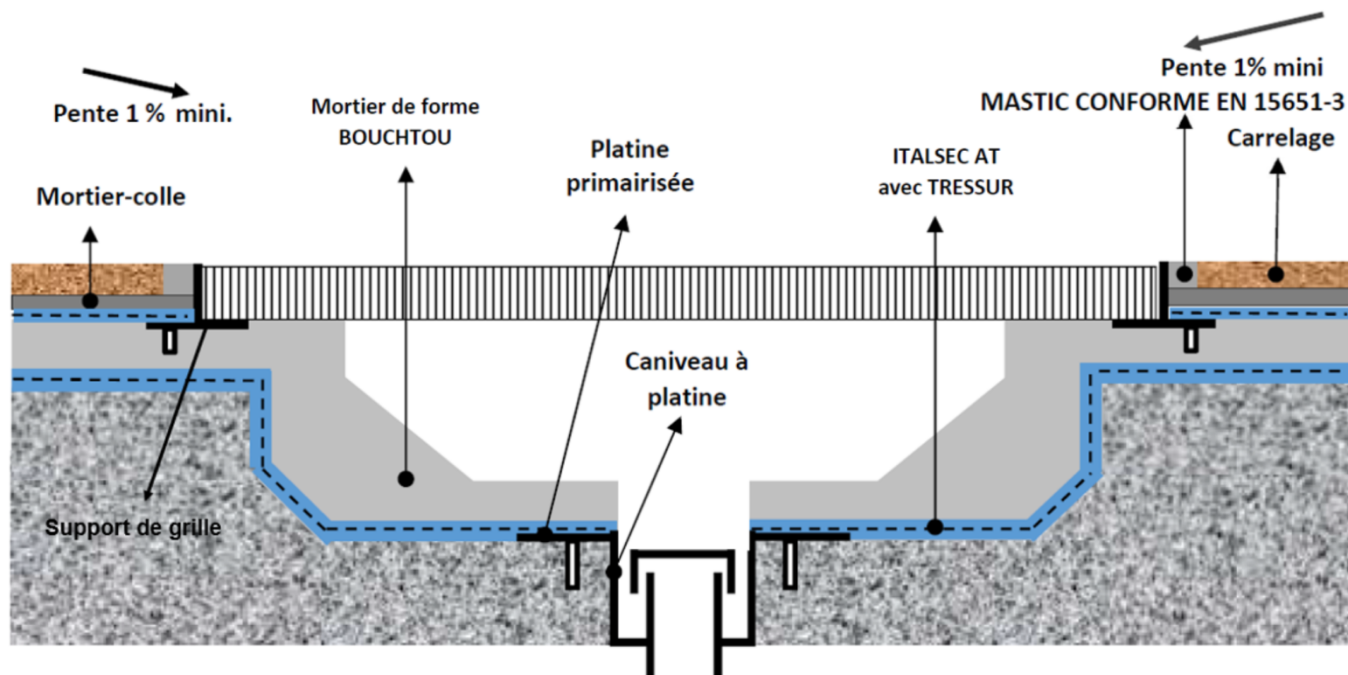
Figure 7a – Dispositif de collecte par caniveau en pose collée
