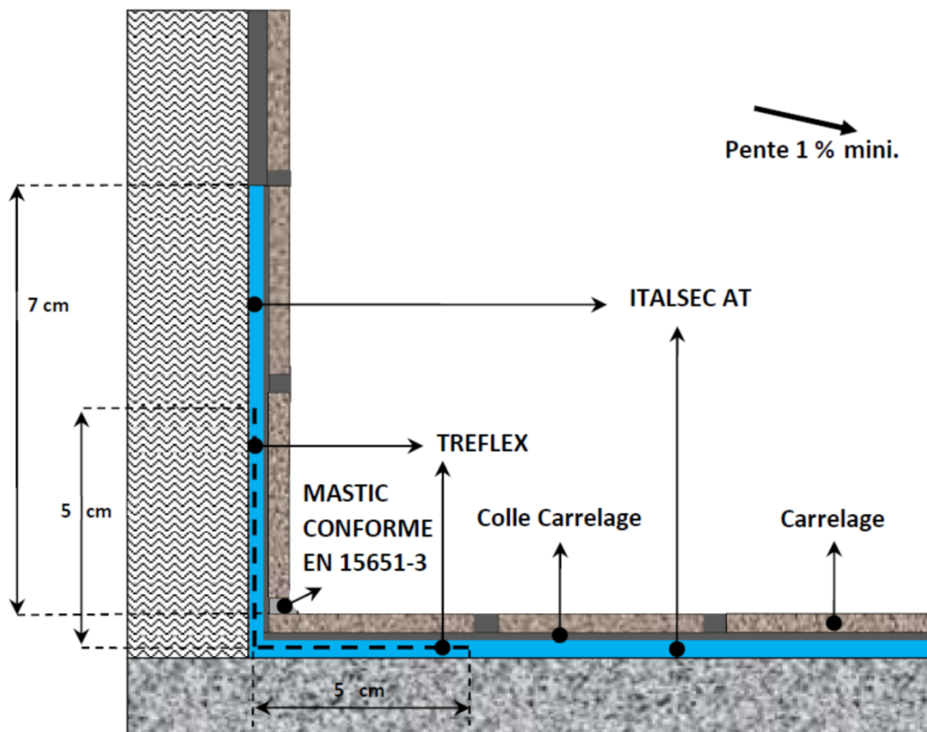
Figure 3 – Relevés et traitement des angles
