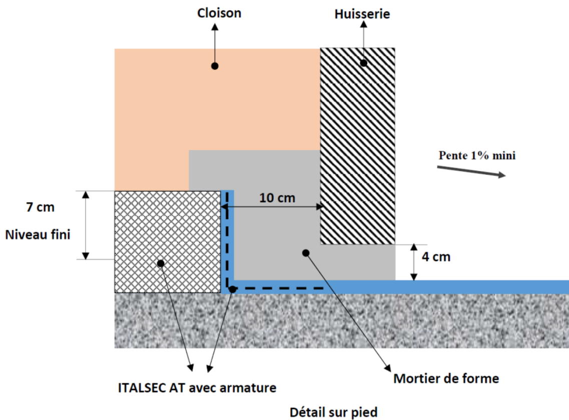
Figure 10b - Traitement huisseries avant pose
