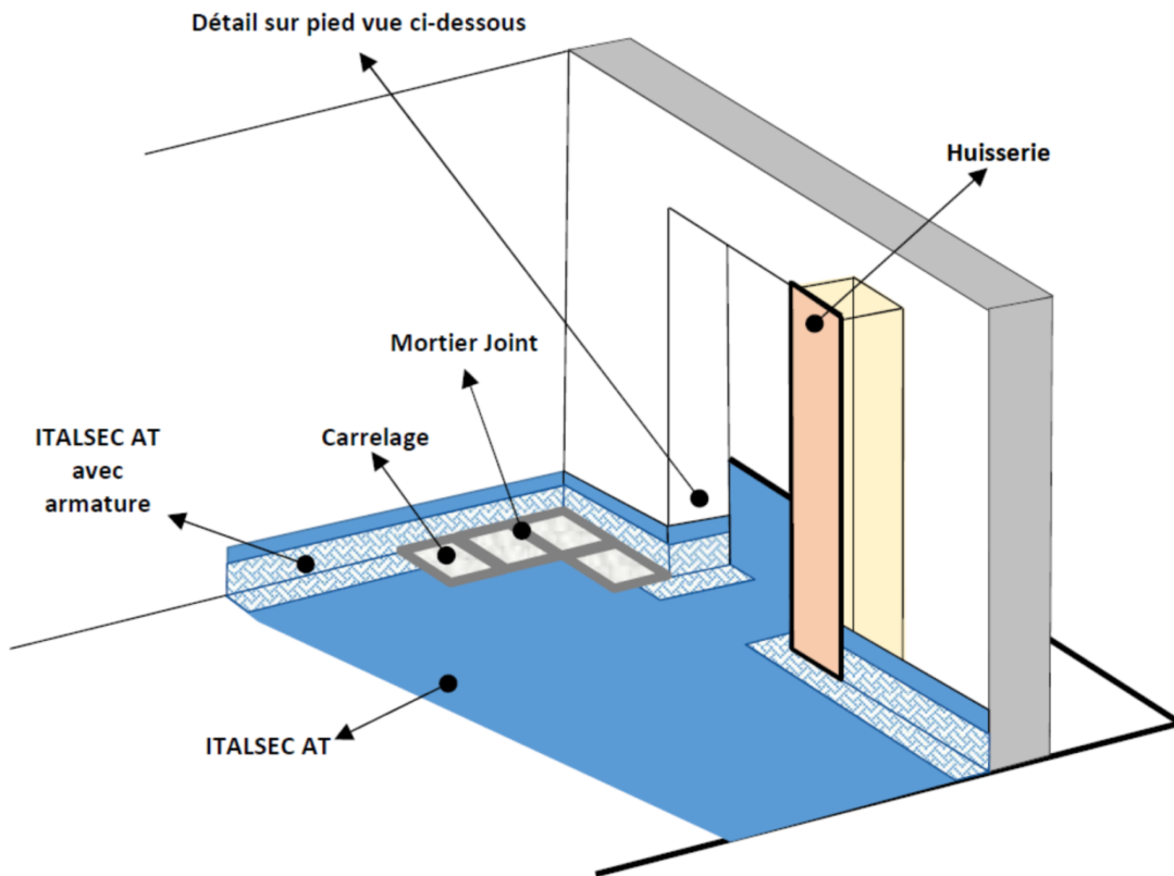
Figure 10a – Traitement huisseries avant pose
