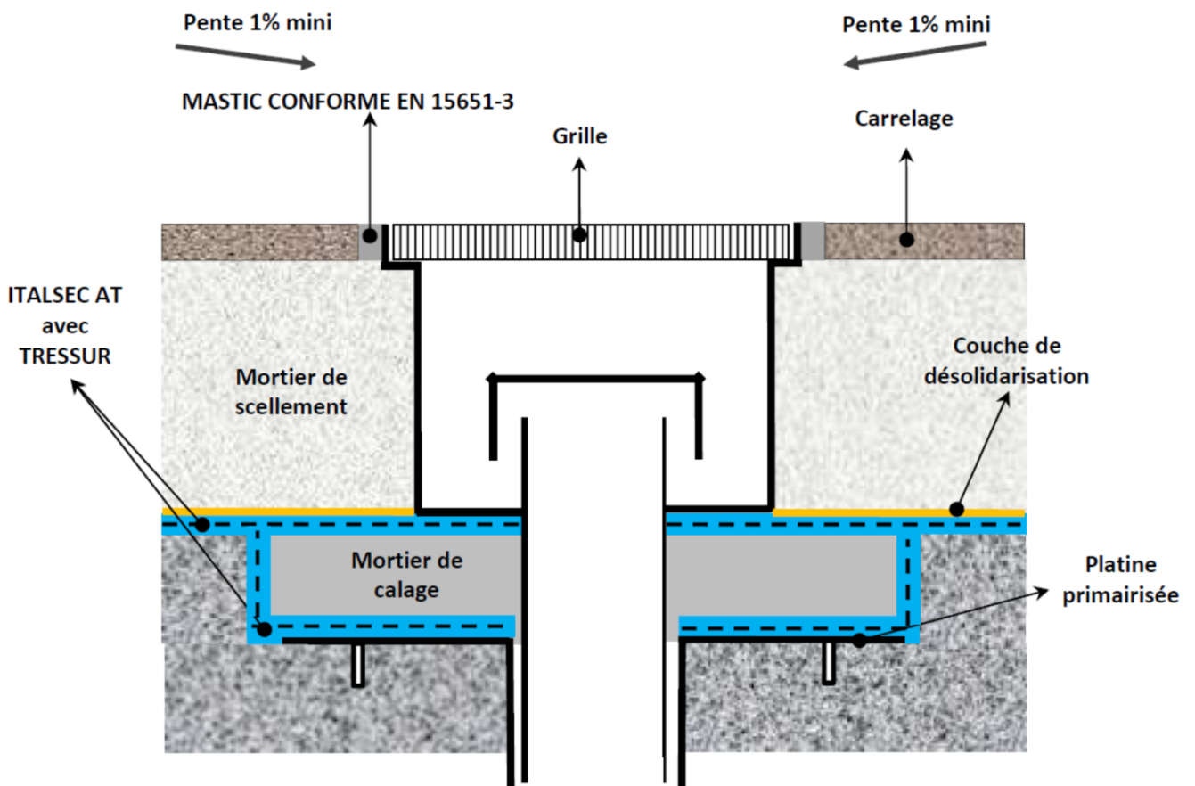
Figure 8b – Dispositif d'évacuation par siphon en pose scellée
