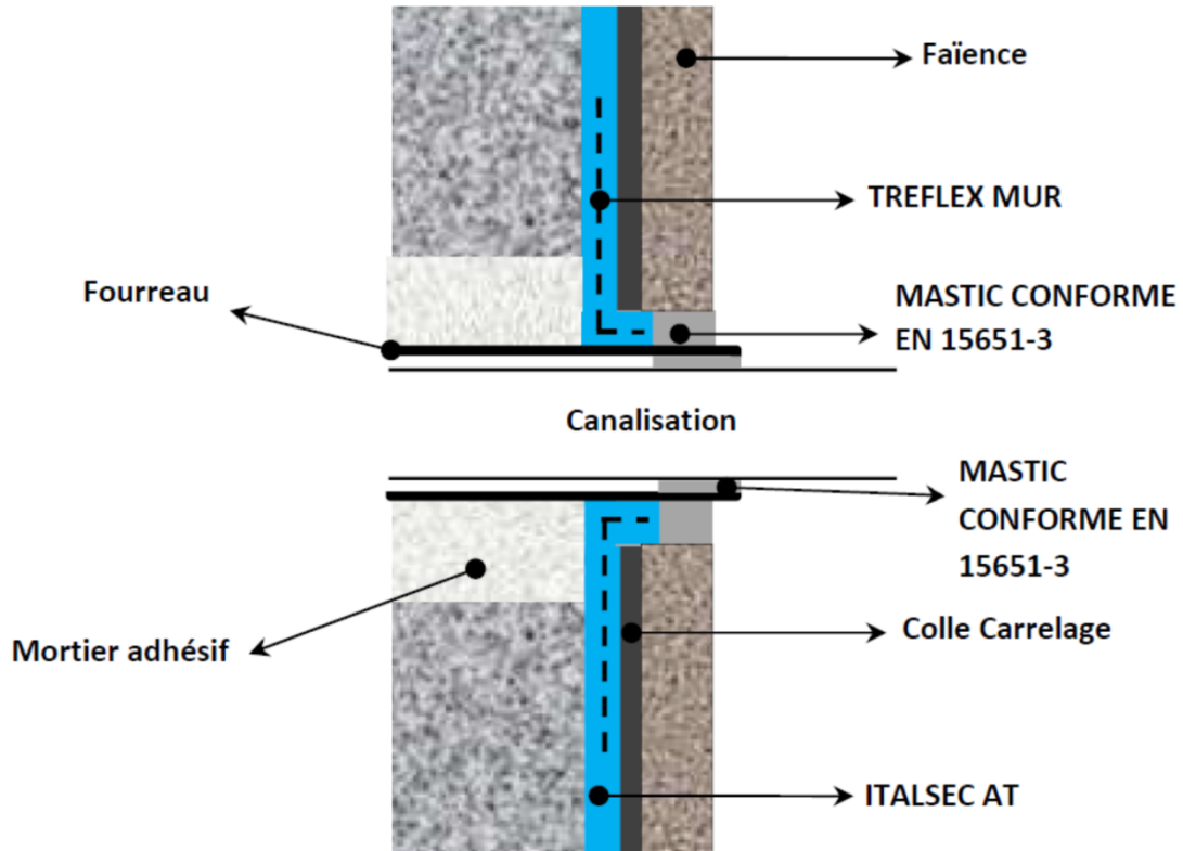
Figure 9a - Traversée de canalisations mur
