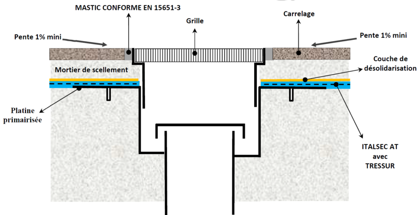
Figure 7b – Dispositif de collecte par caniveau en pose scellée
