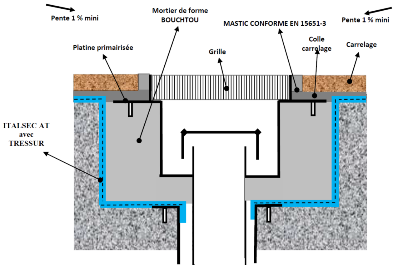
Figure 8a – Dispositif d'évacuation par siphon en pose collée
