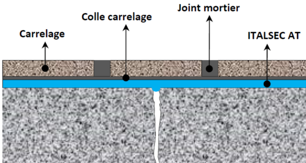
Figure 1 – Microfissures d'ouverture inférieure à 0,3 mm
