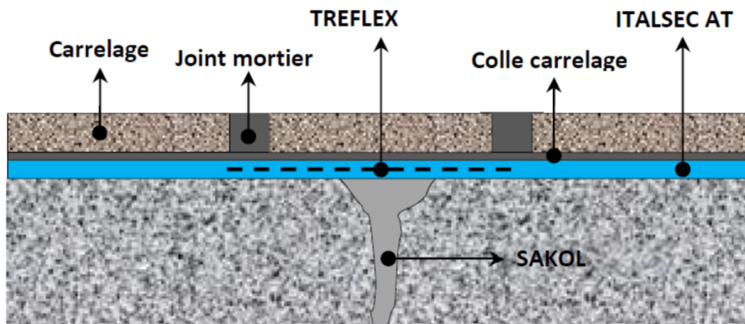
Figure 2 – Fissures d'ouverture comprise entre 0,3 et 2 mm
