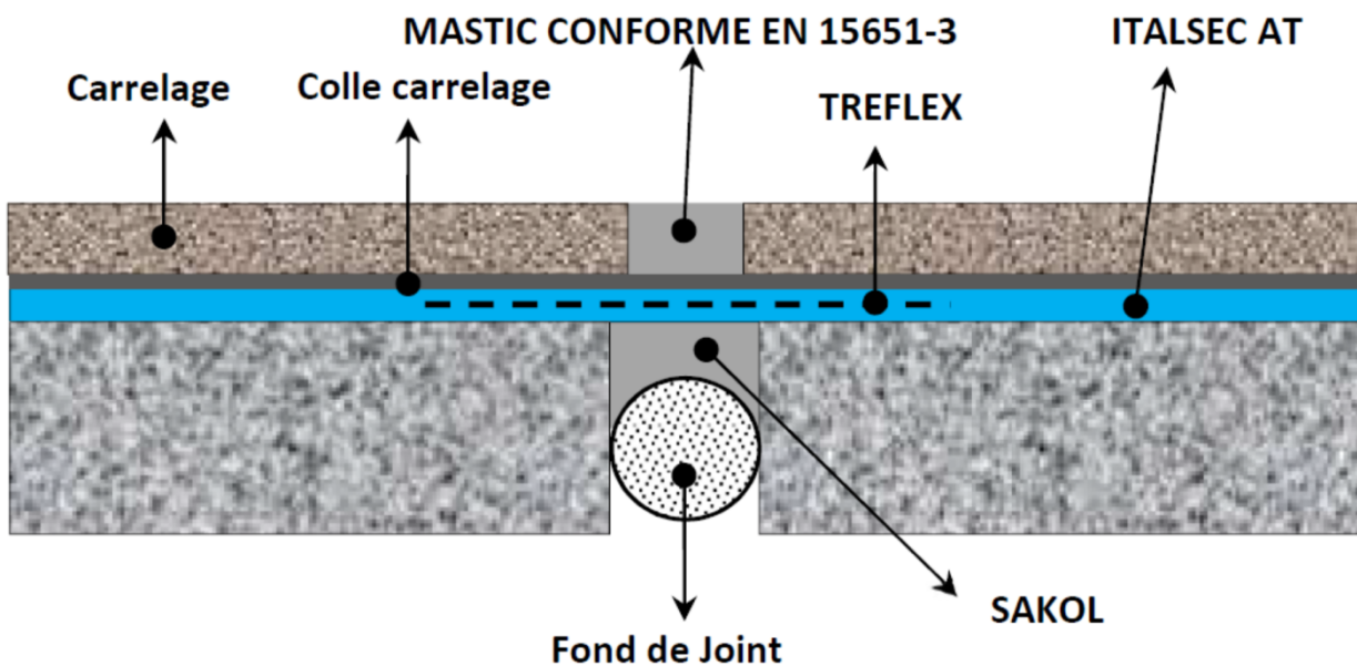
Figure 4 – Joint de retrait et de fractionnement
