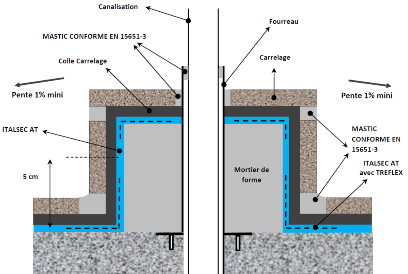
Figure 9b - Traversées de canalisations sol en pose collée
