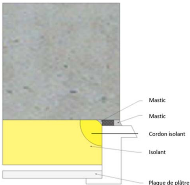
Figure 4 : Menuiserie calfeutrée en applique intérieure, fixée en applique intérieure
