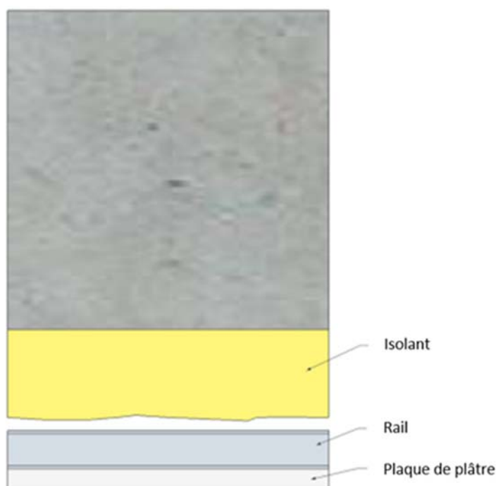
Figure 7 : Projection au niveau des rails
