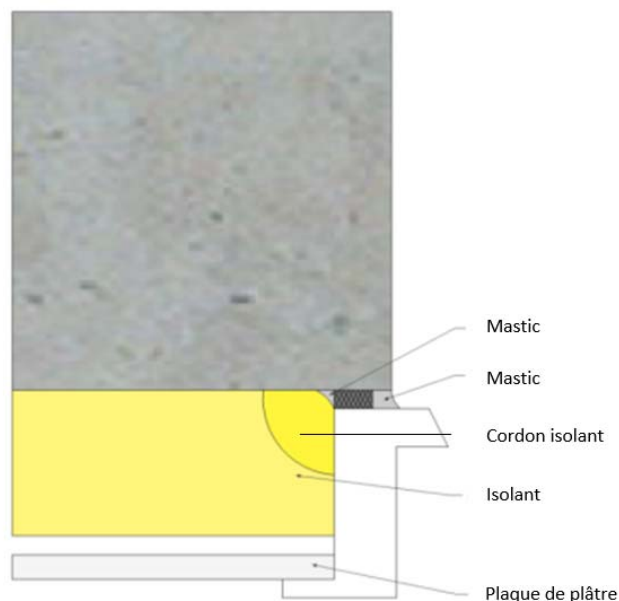
Figure 5 : Menuiserie calfeutrée en tunnel, fixée en tableau
