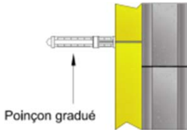
Figure 1 : Contrôle de l'épaisseur
