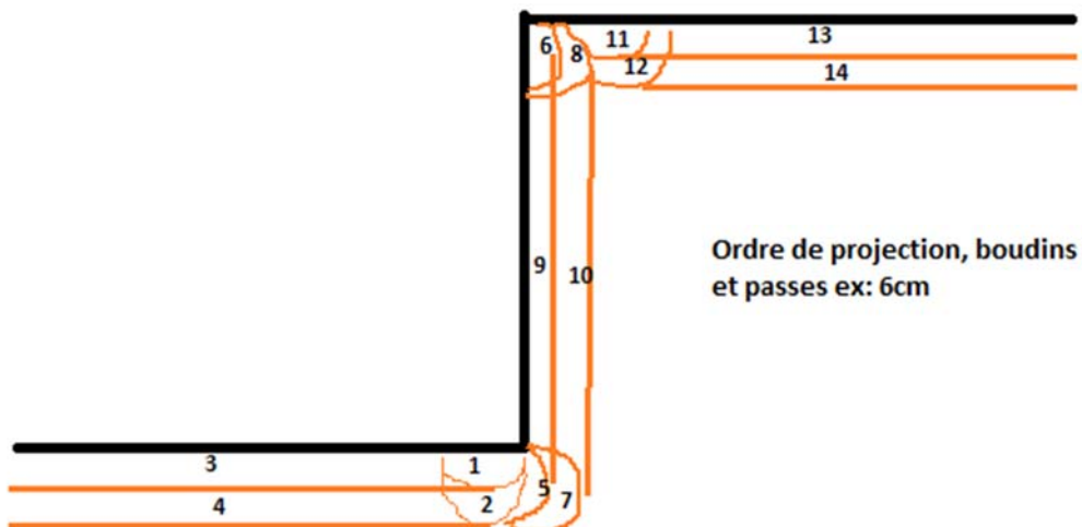
Figure 6 : Traitement des angles rentrants et des angles saillants
