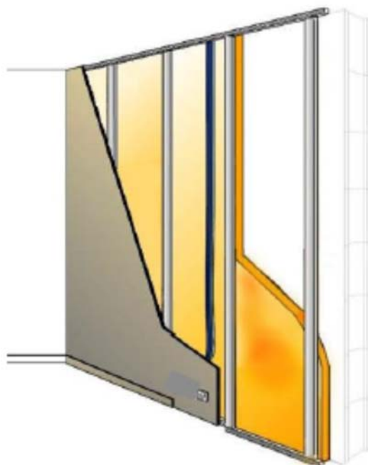
Figure 8 : Contre-cloison constituée de montants simples ou doubles sans fixation intermédiaire au support
