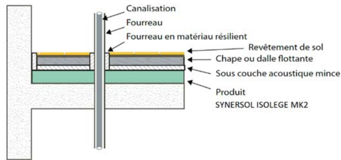
Figure 5 : Traitement d'une canalisation verticale
