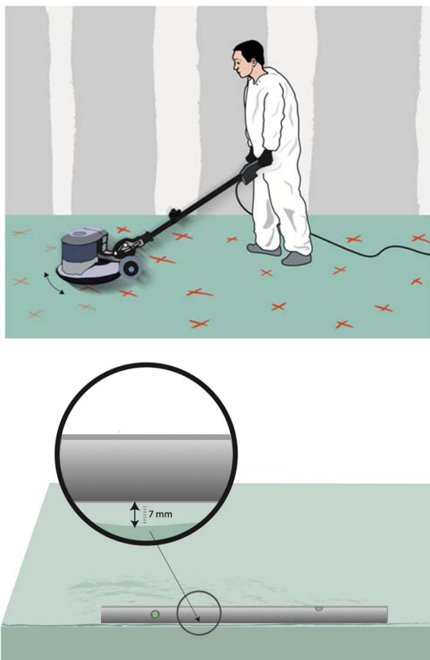
Figure 9 : Tolérance de 7 mm sous la règle de 2 m
