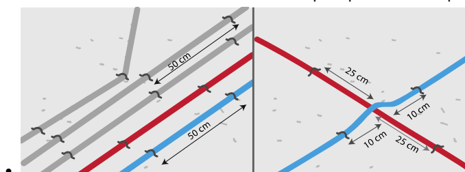
Figure 4 : Fixations des canalisations
