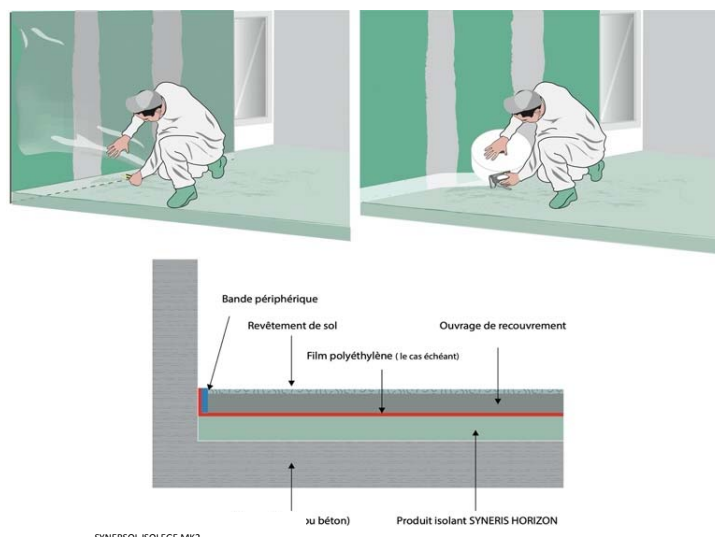
Figure 10 : Réalisation de la désolidarisation périphérique
