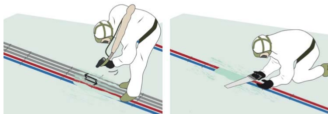
Figure 7 : Enrobage des gaines et arasement de l'excédent
