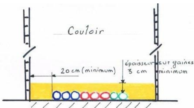
Distance entre périphérie et canalisation
