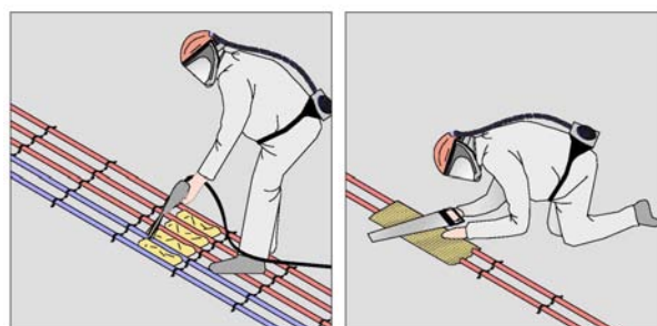
Enrobage des gaines et arasement de l'excédent
