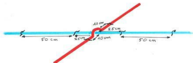
Fixations à 10 cm de l'axe du croisement
