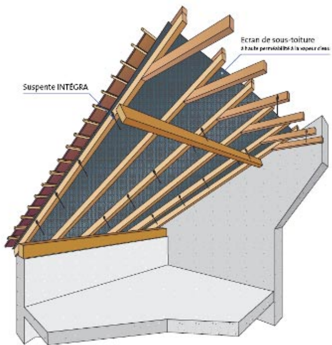
Figure 11 – Pose de suspenes Intégra
