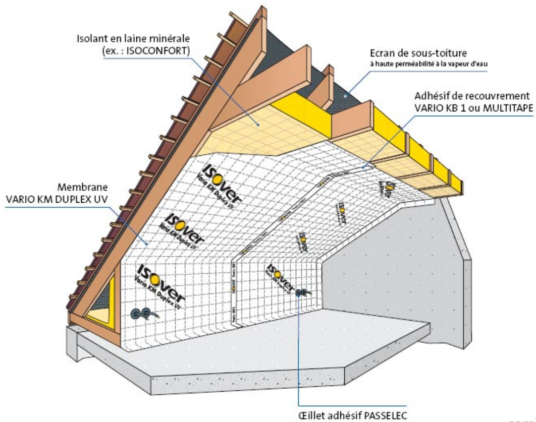
Figure 5 – Jointoiment des lés de membrane VARIO KM DUPLEX UV
