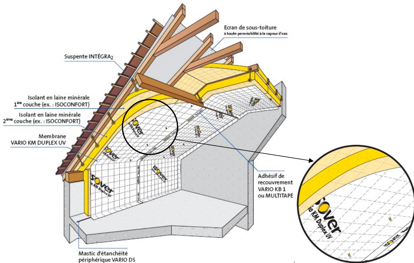
Figure 26 : Pose des lés de membrane VARIO KM DUPLEX UV embrochés sur les corps de suspenstes contre les rondelles
