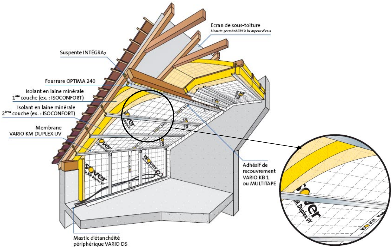
Figure 28 : pose de l'ossature métallique : les fourrures sont clipsées sur les clefs INTEGRA 2 . Les gaines électriques sont passées entre la membrane et l'ossature métallique
