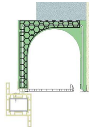
Renfort interne + rail PVC à languette
