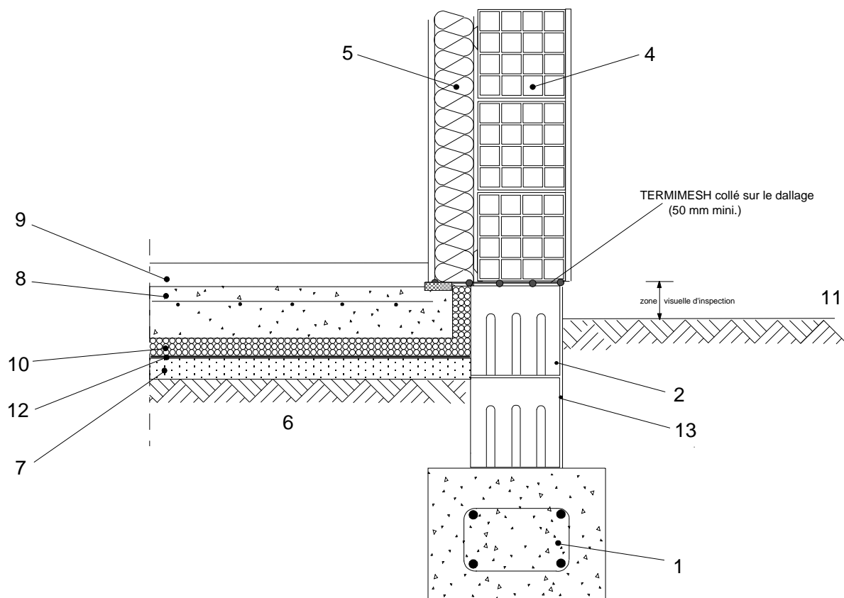
Figure 9 – EU 1.2-2_ dallage-désolidarisée-avec-rupteur (isolant résistant aux termites)
