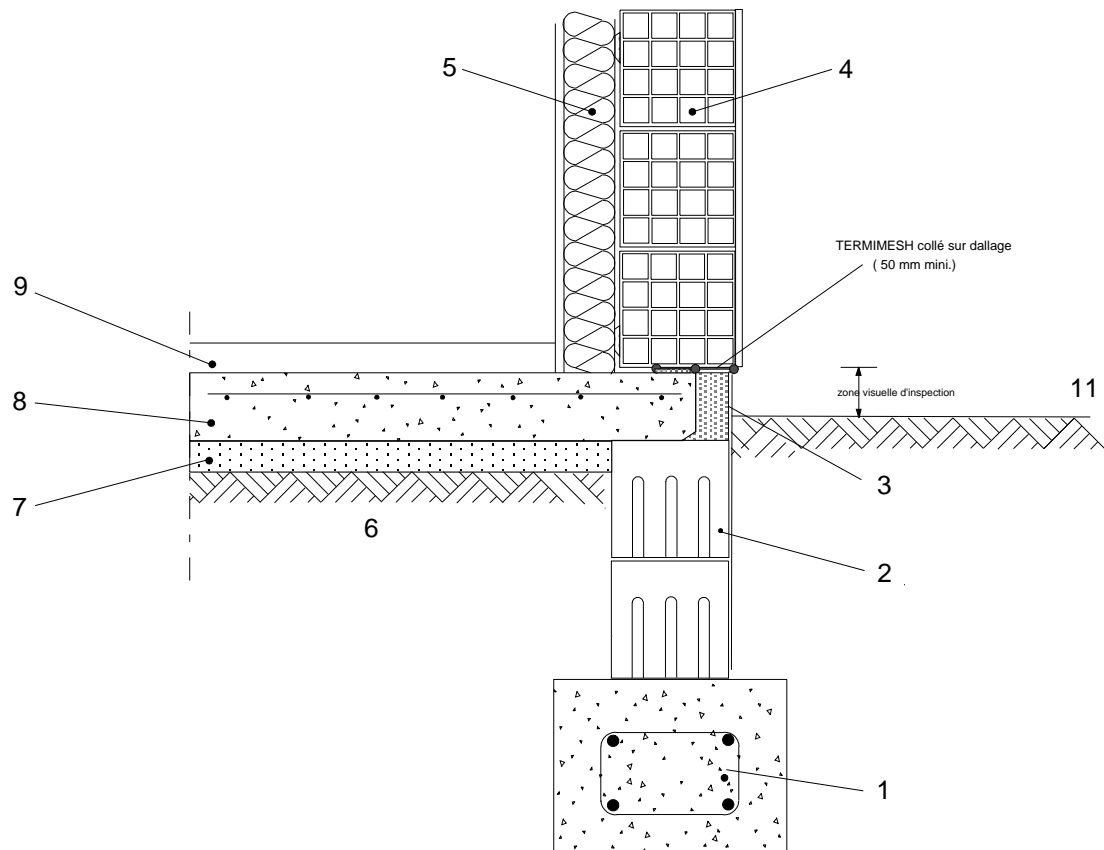
Figure 3 – EU 1.1-1_dallage -mur-maçoné-planelle-béton-et-brique
