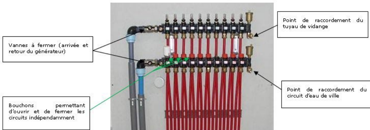
Figure 10 - Procédure de purge avec présence de points hauts
