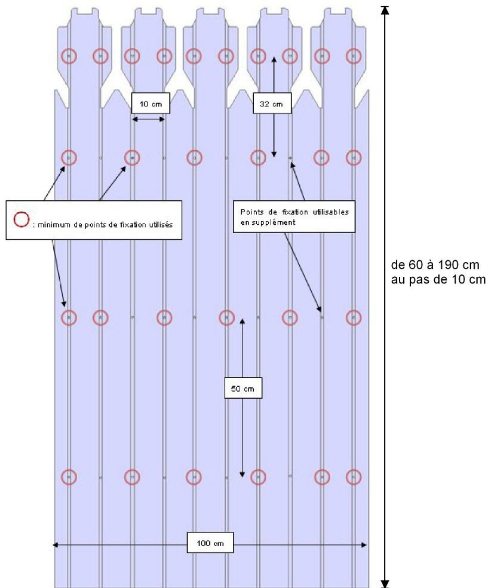
Figure 1 - Présentation d'un diffuseur et plan de vissage
