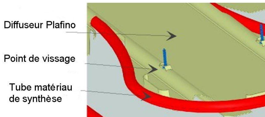
Figure 2 - Détail emboutissage pour fixation
