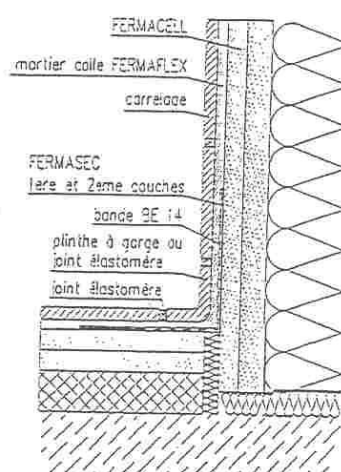
Figure 13 – Liaison cloison séparative et chape sèche FERMACELL avec revêtement carrelage
