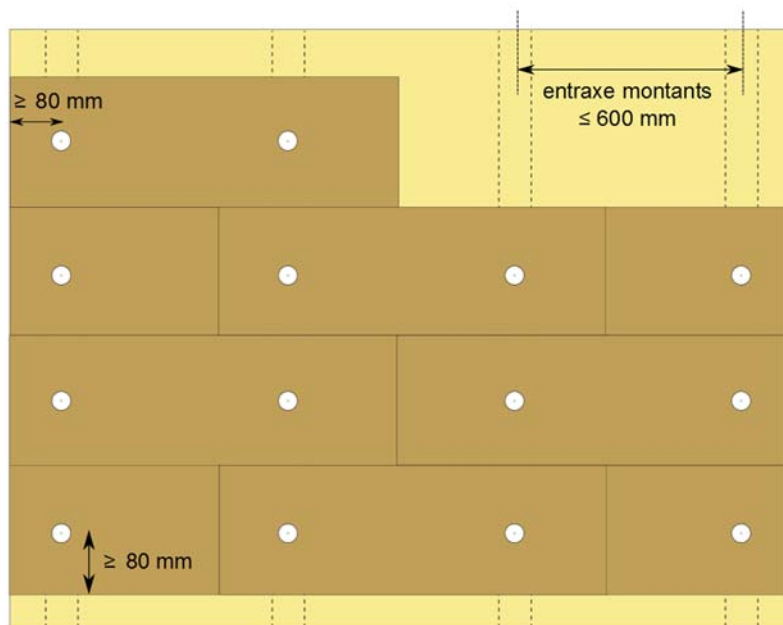
2 vis à rosace par panneau (1 vis par montant)
