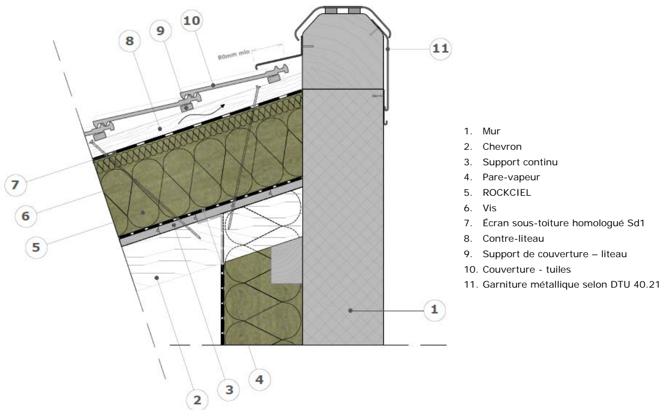
Figure 17 – Exemple de faitage simple pente, climat de plaine
