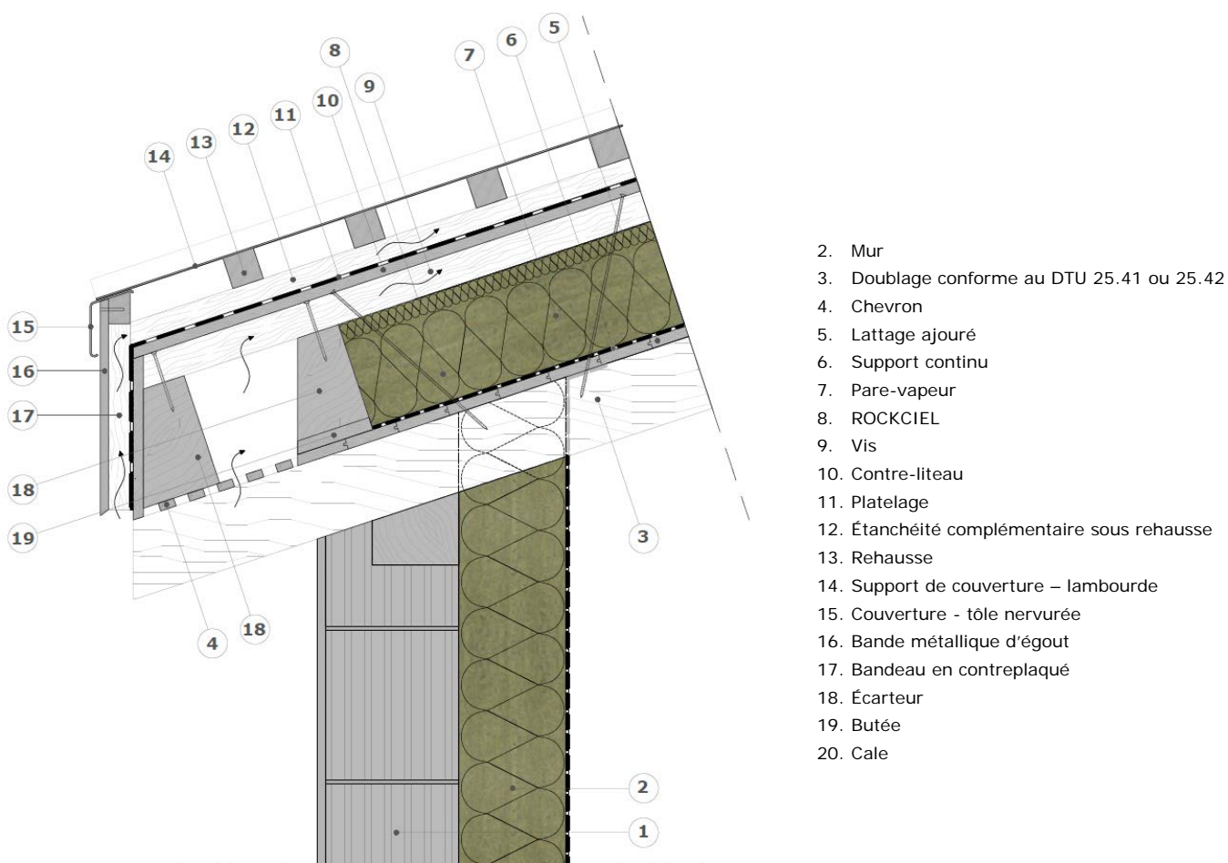
Figure 16 – Exemple de rive d'égout longs débords, climat de montagne
