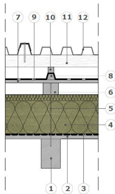
Figure 1 – Nomenclature des éléments de toiture en partie courante, climat de plaine, avec écran sous-toiture homologué Sd1 ( gauche ) et avec écran sous-toiture homologué Sd2 ou Sd3 en pose tendue ( droite )
