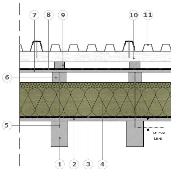
Figure 1 – Nomenclature des éléments de toiture en partie courante, climat de plaine, avec écran sous-toiture homologué Sd1 ( gauche ) et avec écran sous-toiture homologué Sd2 ou Sd3 en pose tendue ( droite )
