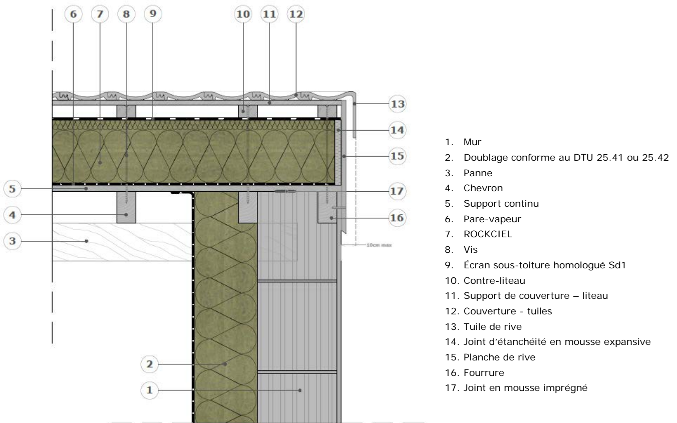
Figure 7 – Exemple de rive petits débords, climat de plaine
