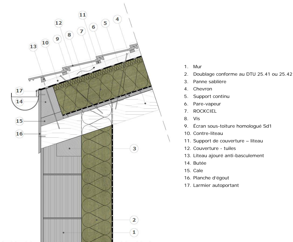
Figure 14 – Exemple de rive d'égout petits débords, climat de plaine
