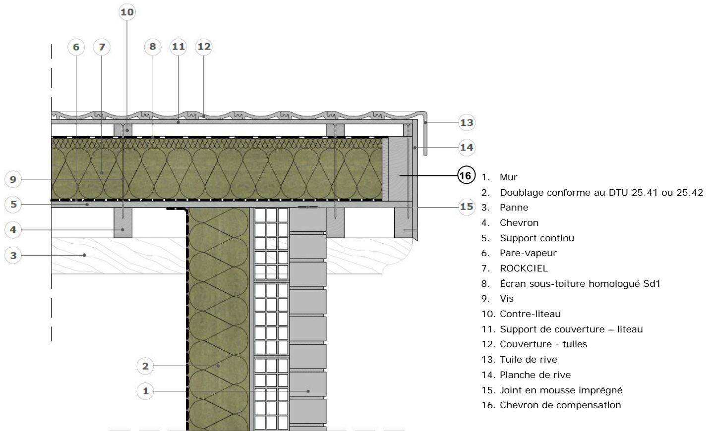
Figure 9 – Exemple de rive longs débords, climat de plaine
