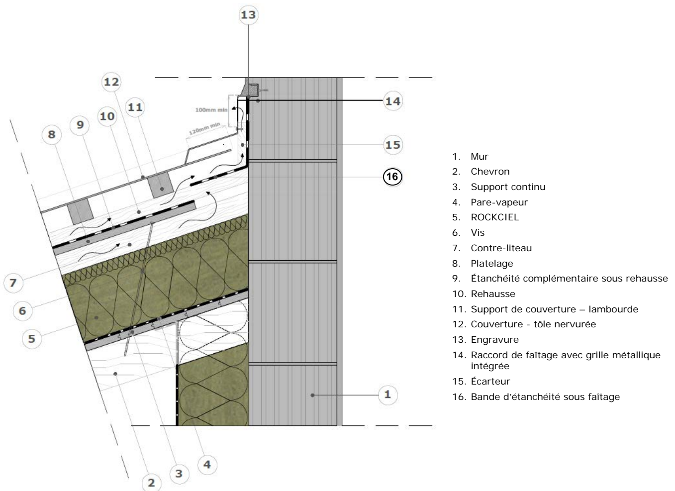
Figure 12 – Exemple de faitage ventilé contre mur, climat de montagne
