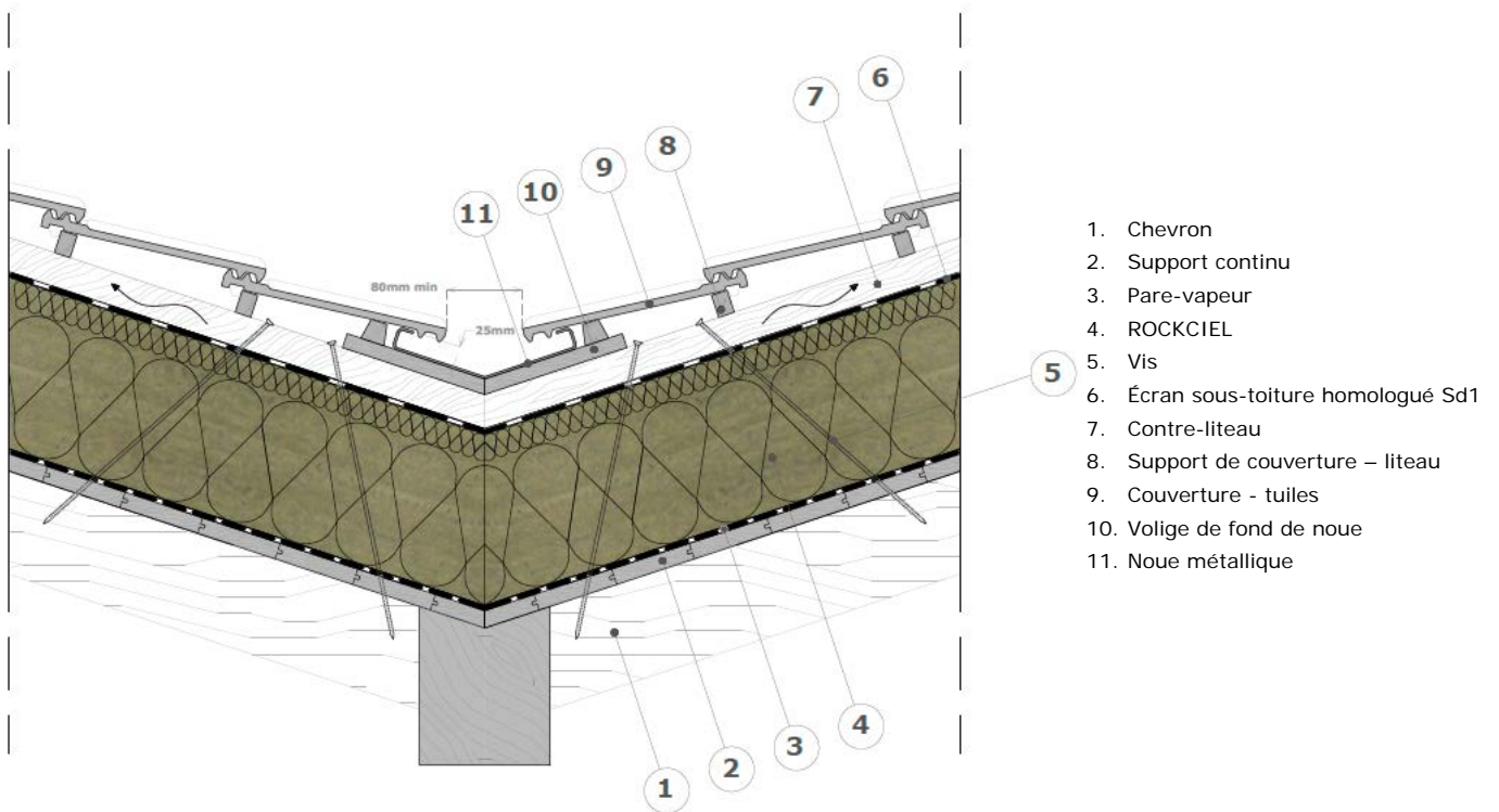
Figure 21 – Exemple de noue, climat de plaine
