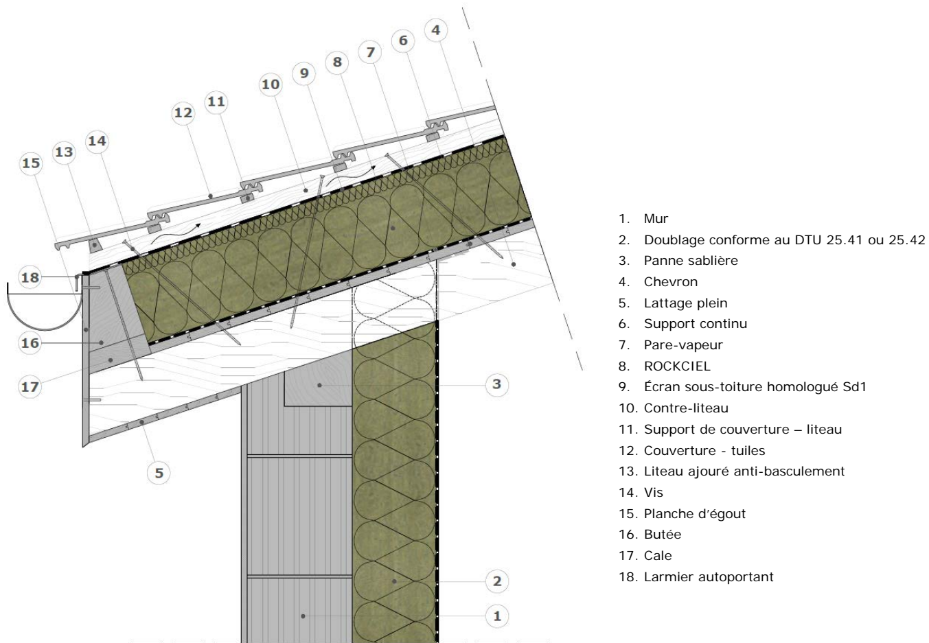
Figure 15 – Exemple de rive d'égout longs débords, climat de plaine
