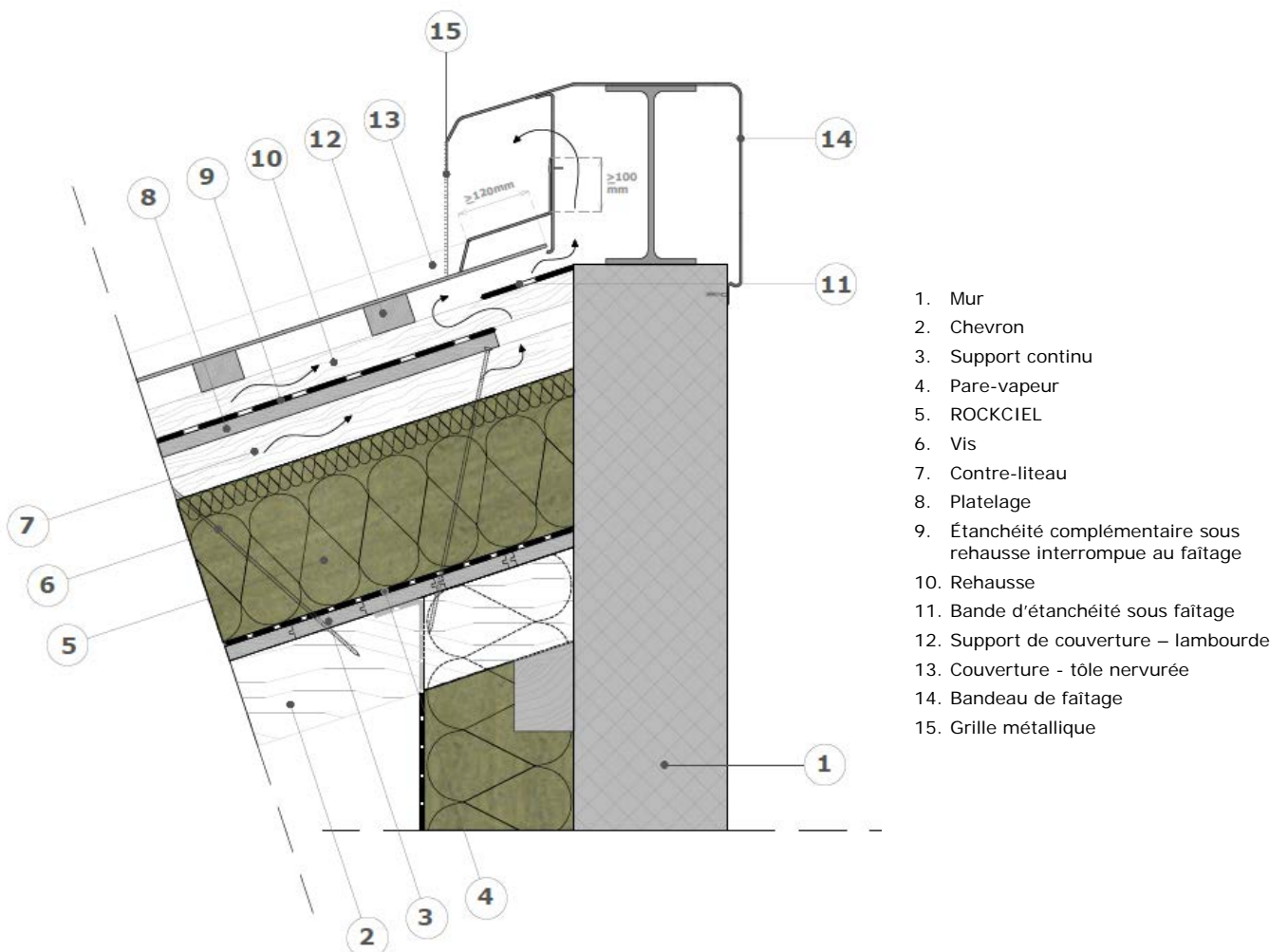
Figure 18 – Exemple de faitage simple pente, climat de montagne
