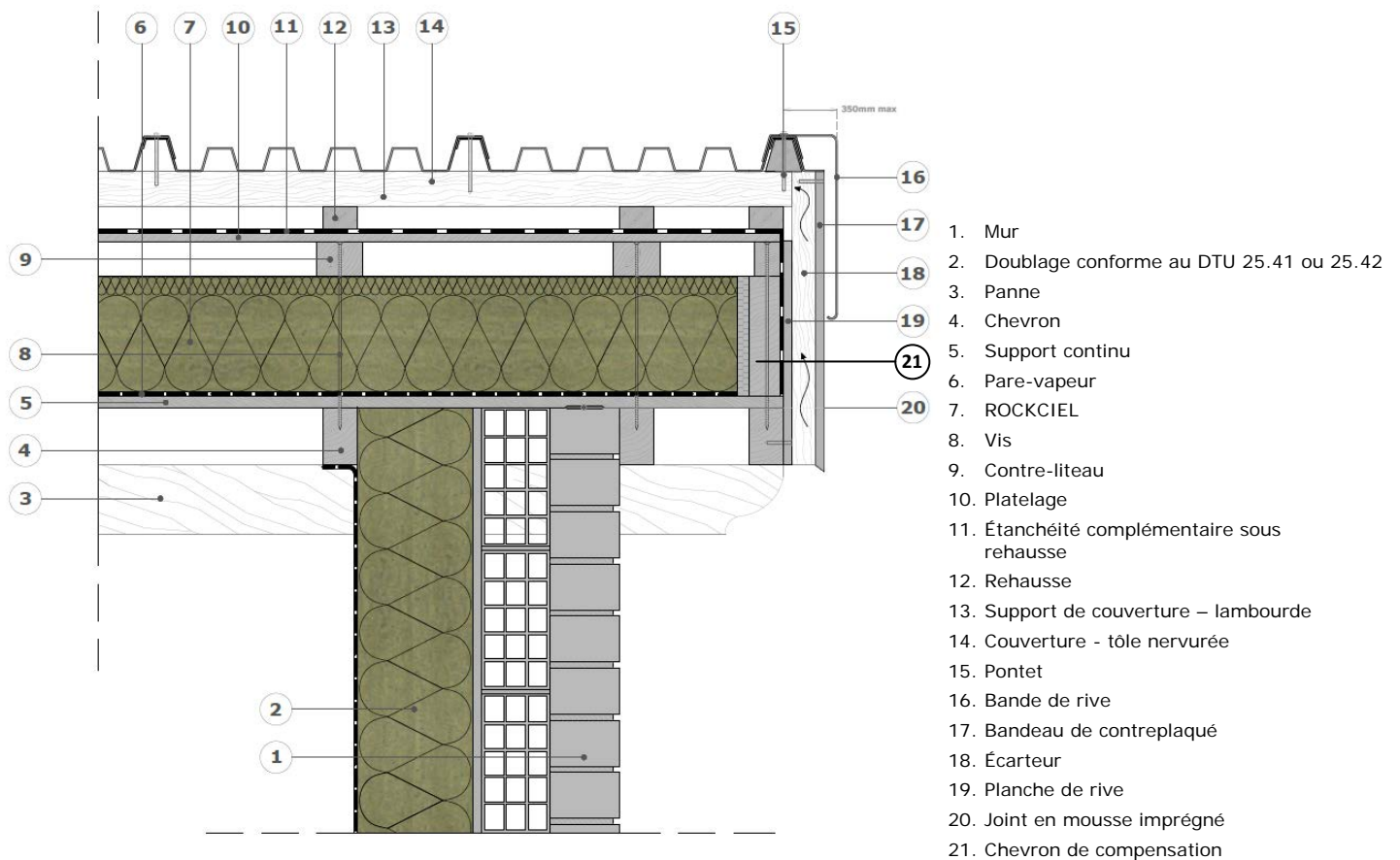
Figure 10 – Exemple de rive longs débords, climat de montagne
