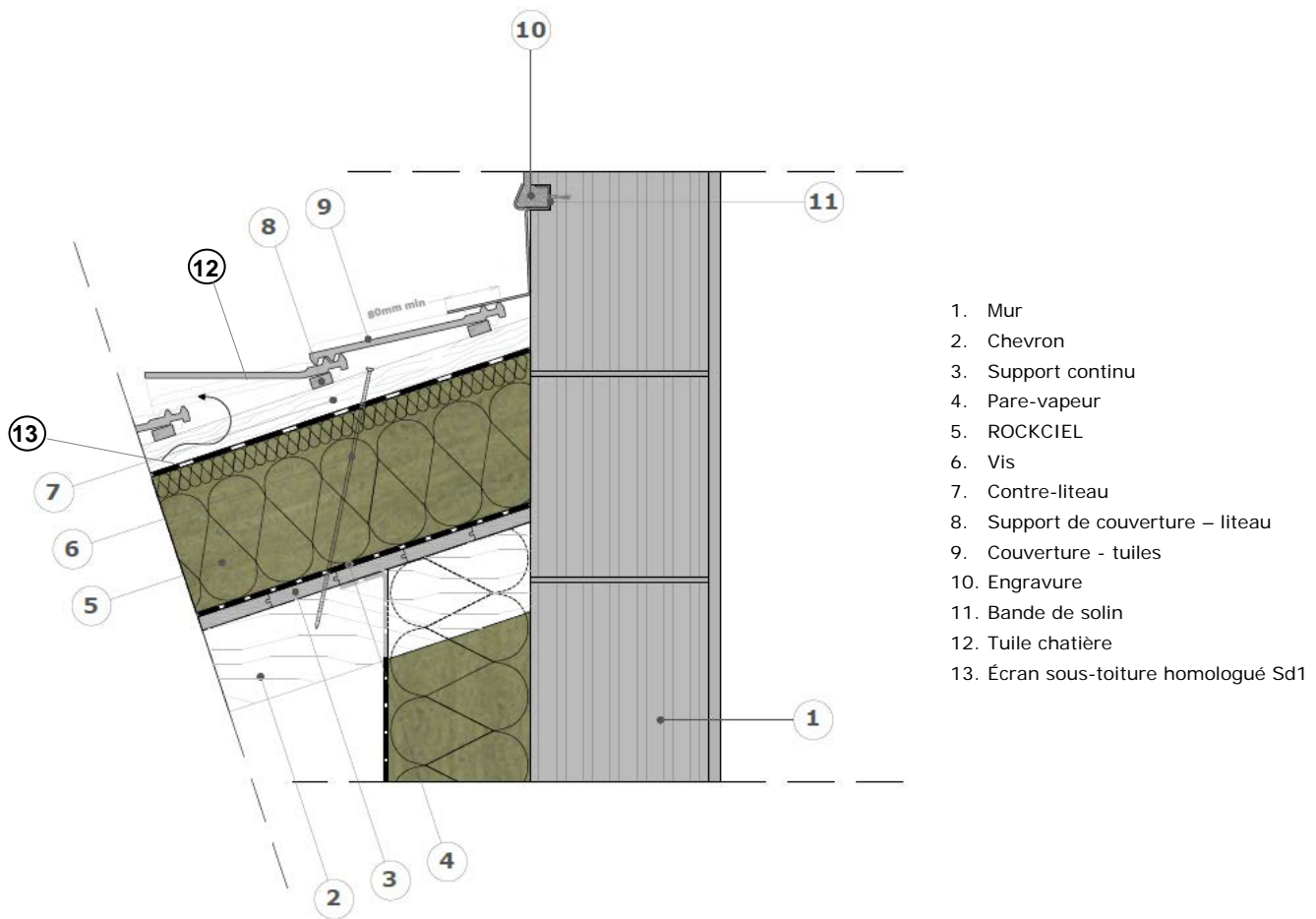
Figure 11 – Exemple de faitage contre mur, climat de plaine
