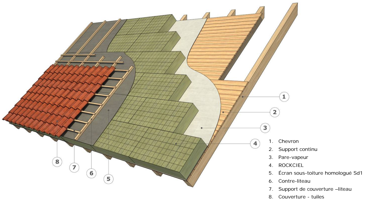
Figure 3 – Vue générale du procédé Sarking Rockciel en partie courante, climat de plaine
