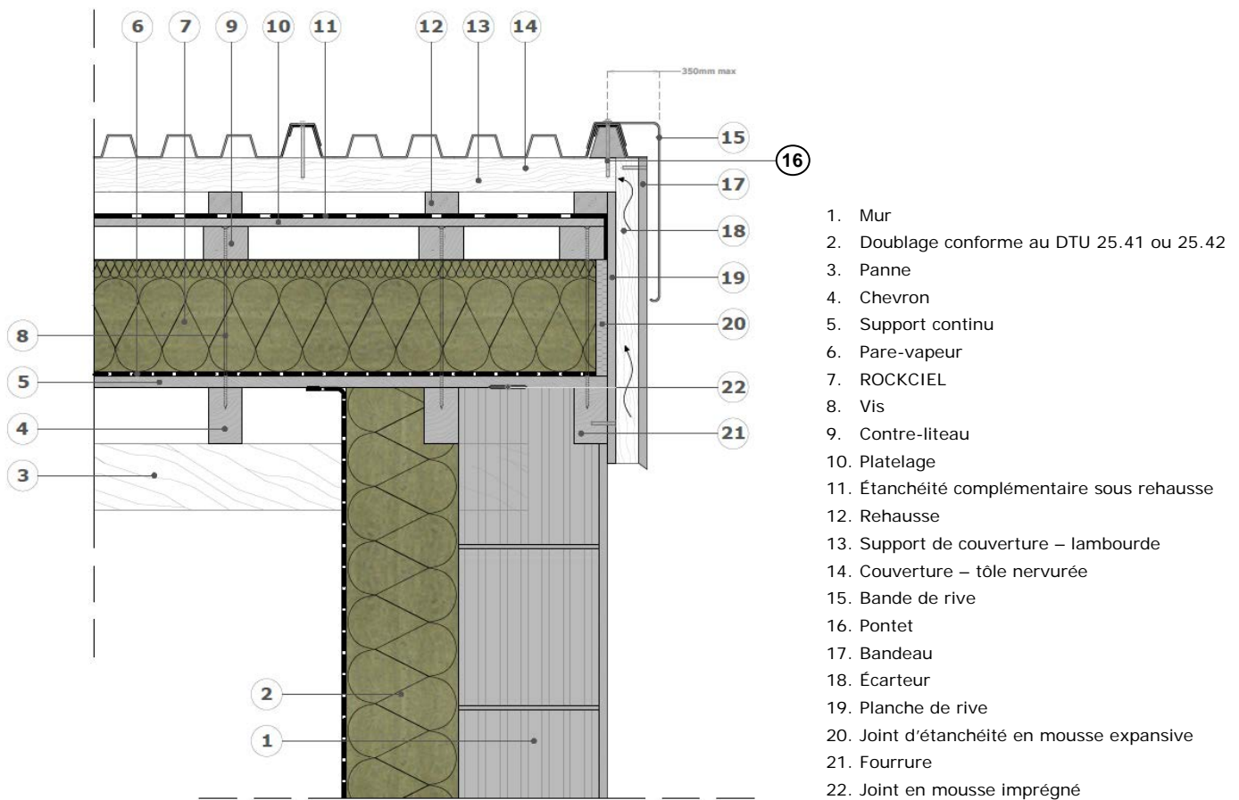
Figure 8 – Exemple de rive petits débords, climat de montagne
