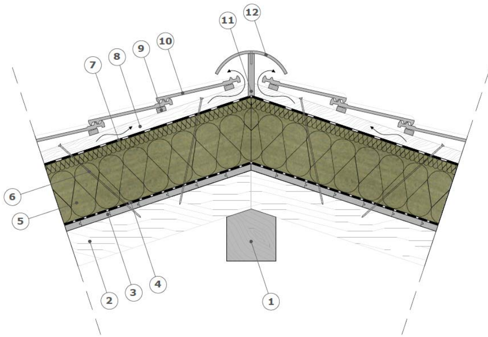
Figure 19 – Exemple de faitage double pente, climat de plaine
