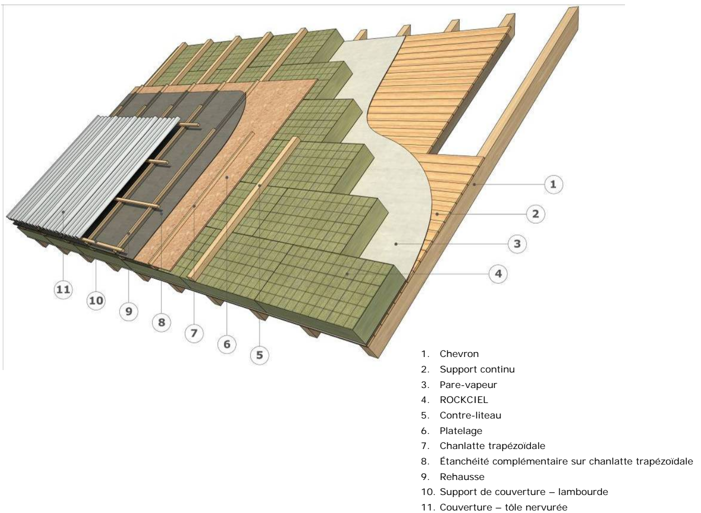
Figure 4 – Vue générale du procédé Sarking Rockciel en partie courante, climat de montagne
